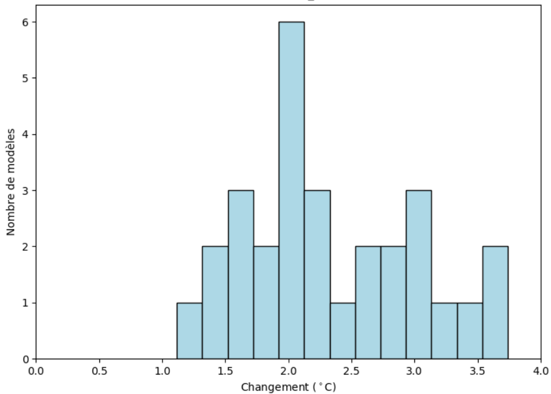
Zone de la côte guinéenne : Changements du maximum de Température Maximale Journalière (juin ; rcp85; BC_0.5x0.5)
