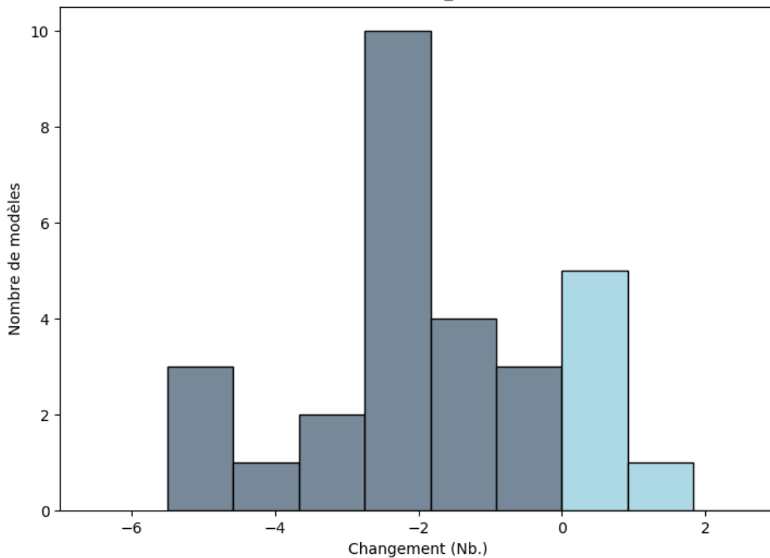
Zone de la côte guinéenne: Changements du nombre de séquences pluvieuses de plus de 10 jours (juin; rcp85; BC_0.5x0.5)
