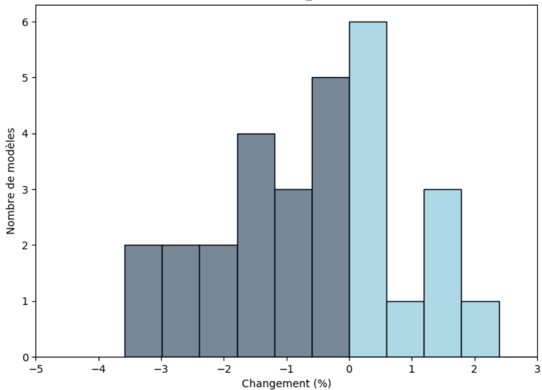
Zone de la côte guinéenne : Changements (%) du maximum de Flux Solaire Entrant À La Surface (juin ; rcp85; BC_0.5x0.5)
