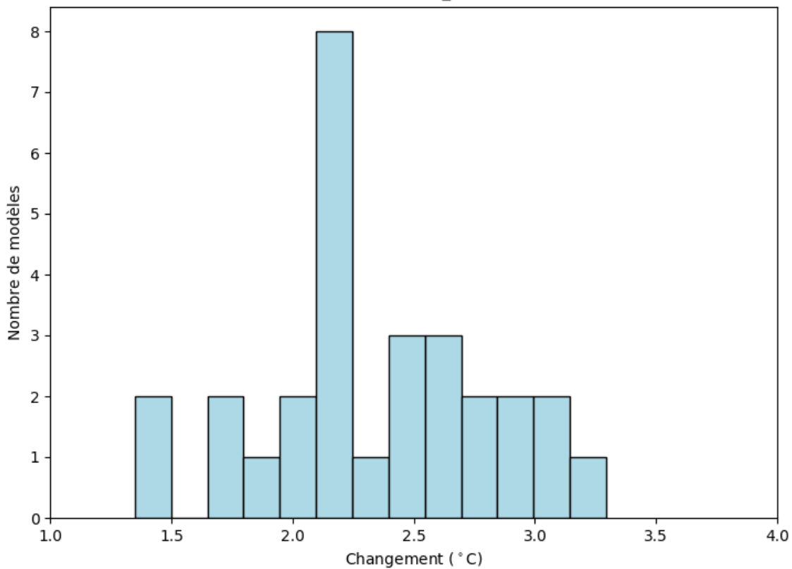
Zone de la côte guinéenne : Changements de la minimum de Température Minimale Journalière (juin ; rcp85; BC_0.5x0.5)
