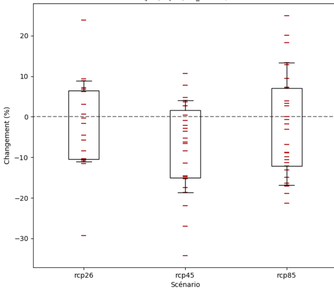
Zone de la côte guinéenne: Changements (%) du maximum de précipitations totales sur une période de 3 jours (juin; rcp85; BC_0.5x0.5)
