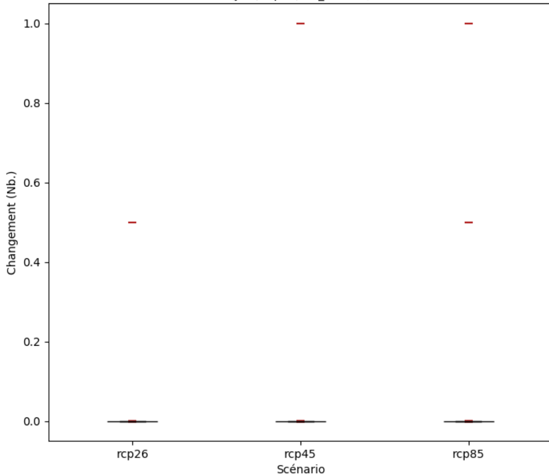
Zone de la côte guinéenne: Changements du nombre de jours avec des précipitations > 30 \text{ mm jour}^{-1} (juin; rcp85; BC_0.5x0.5)
