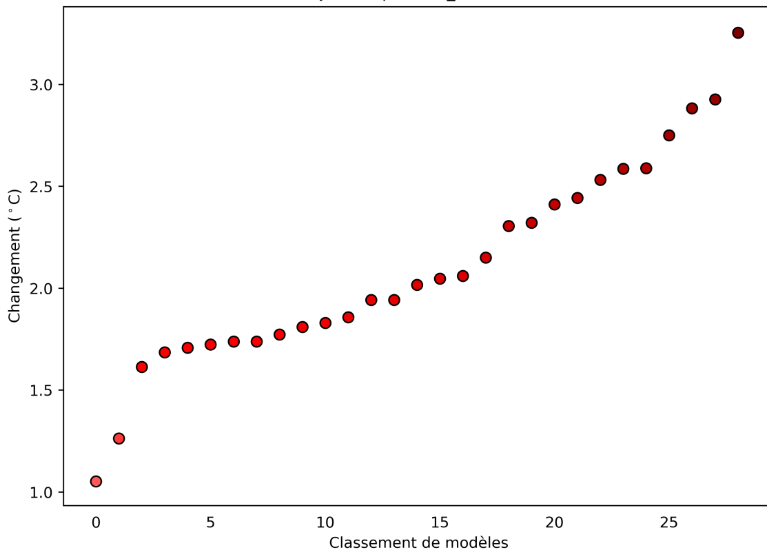
Zone de la côte guinéenne : Changements de la moyenne de Température Moyenne Journalière (juin ; rcp85; BC_0.5x0.5)
