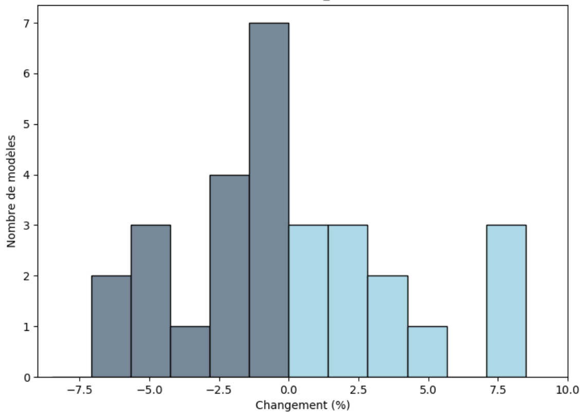
Zone de la côte guinéenne : Changements (%) de la moyenne de Flux Solaire Entrant À La Surface (juin ; rcp85; BC_0.5x0.5)
