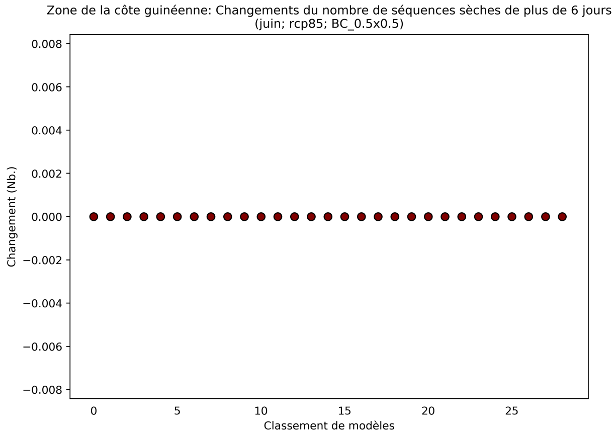
Figure 24: Ce diagramme de dispersion illustre la variation absolue du nombre de séquences sèches de plus de 6 jours entre 2040 et 2059 (par rapport à la période de référence de 1950 à 2000) pour juin. Chaque point indique la moyenne spatiale d'un modèle sur Zone de la côte guinéenne; les points sont organisés ("rank", sur l'axe des abscisses) en fonction de la magnitude de leur valeur sur l'axe des ordonnées. Ce diagramme montre la variation absolue pour le scénario RCP8.5.
