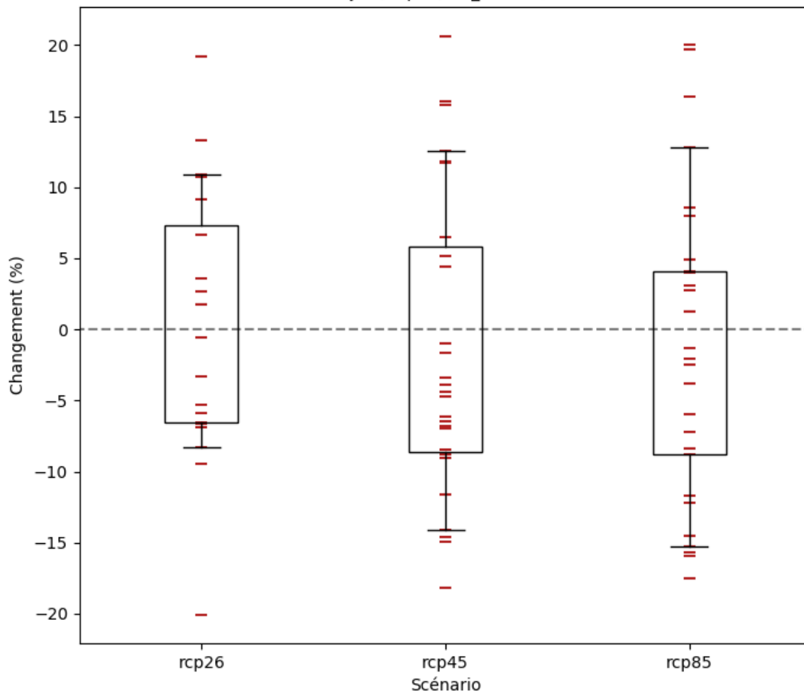
Zone de la côte guinéenne: Changements (%) du maximum de précipitations totales sur une période de 5 jours (juin; rcp85; BC_0.5x0.5)
