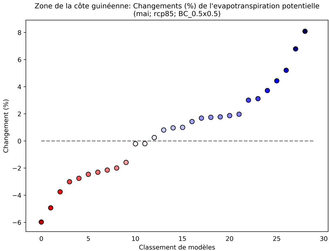
Figure 4: Ce diagramme de dispersion illustre du pourcentage de variation de l'évapotranspiration potentielle entre 2040 et 2059 (par rapport à la période de référence de 1950 à 2000) pour mai. Chaque point indique la moyenne spatiale d'un modèle sur Zone de la côte guinéenne; les points sont organisés ("rank", sur l'axe des abscisses) en fonction de la magnitude de leur valeur sur l'axe des ordonnées. Ce diagramme montre le pourcentage de variation pour le scénario RCP8.5.
