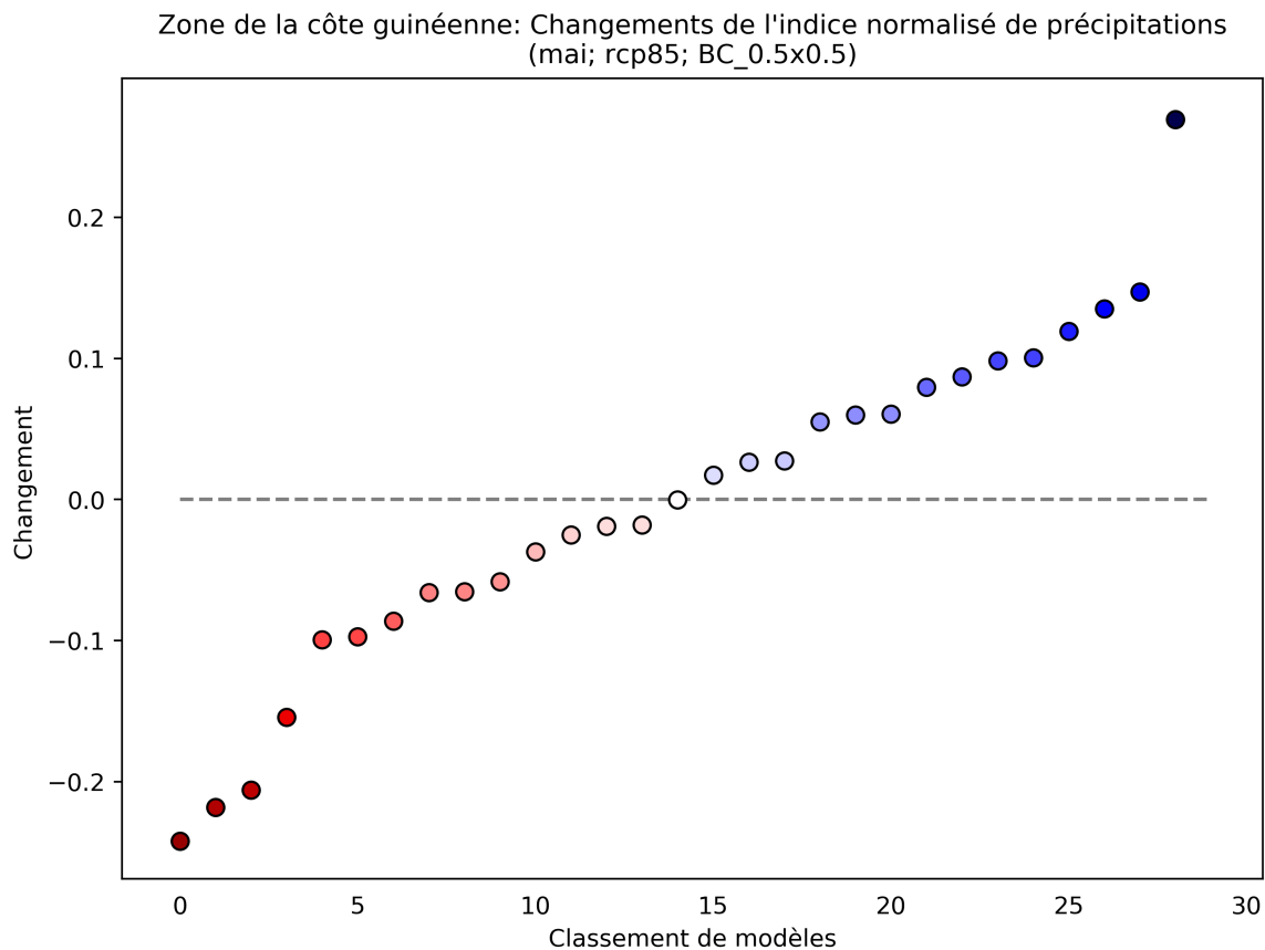
Figure 12: Ce diagramme de dispersion illustre la variation absolue de l'indice normalisé de précipitations entre 2040 et 2059 (par rapport à la période de référence de 1950 à 2000) pour mai. Chaque point indique la moyenne spatiale d'un modèle sur Zone de la côte guinéenne; les points sont organisés ("rank", sur l'axe des abscisses) en fonction de la magnitude de leur valeur sur l'axe des ordonnées. Ce diagramme montre la variation absolue pour le scénario RCP8.5.
