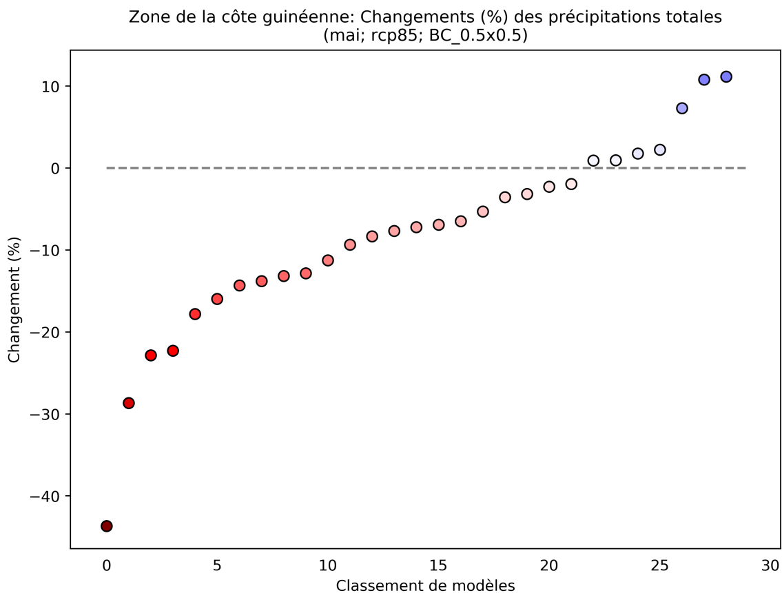
Figure 44: Ce diagramme de dispersion illustre du pourcentage de variation des précipitations totales entre 2040 et 2059 (par rapport à la période de référence de 1950 à 2000) pour mai. Chaque point indique la moyenne spatiale d'un modèle sur Zone de la côte guinéenne; les points sont organisés ("rank", sur l'axe des abscisses) en fonction de la magnitude de leur valeur sur l'axe des ordonnées. Ce diagramme montre le pourcentage de variation pour le scénario RCP8.5.
