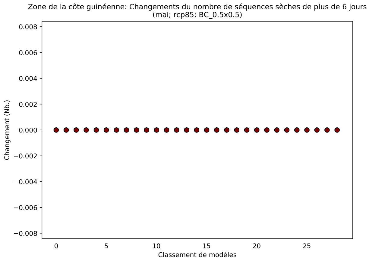
Figure 24: Ce diagramme de dispersion illustre la variation absolue du nombre de séquences sèches de plus de 6 jours entre 2040 et 2059 (par rapport à la période de référence de 1950 à 2000) pour mai. Chaque point indique la moyenne spatiale d'un modèle sur Zone de la côte guinéenne; les points sont organisés ("rank", sur l'axe des abscisses) en fonction de la magnitude de leur valeur sur l'axe des ordonnées. Ce diagramme montre la variation absolue pour le scénario RCP8.5.
