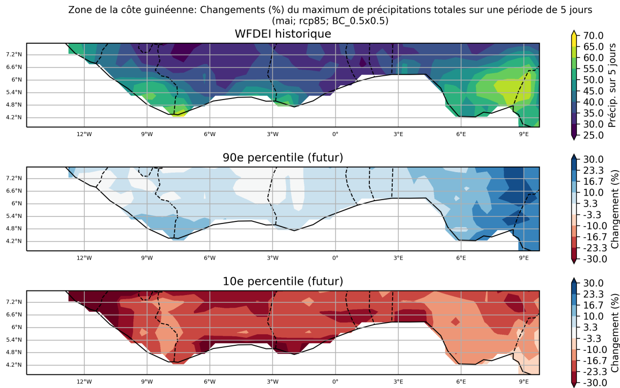
Figure 80: Ces cartes illustrent la projection multi-modèles pour du pourcentage de variation du maximum de précipitations totales sur une période de 5 jours, pour la période entre 2040 et 2059 (par rapport à la période de référence de 1950 à 2000) pour mai. Elles indiquent les 90ème et 10ème percentiles de la distribution des modèles dans l'ensemble multi-modèles, calculés séparément en chaque point de grille, sur la région Zone de la côte guinéenne. Ce diagramme montre le pourcentage de variation pour le scénario RCP8.5.
