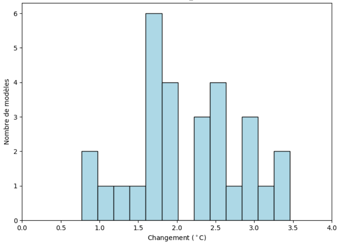
Zone de la côte guinéenne : Changements du maximum de Température Maximale Journalière (mai ; rcp85; BC_0.5x0.5)
