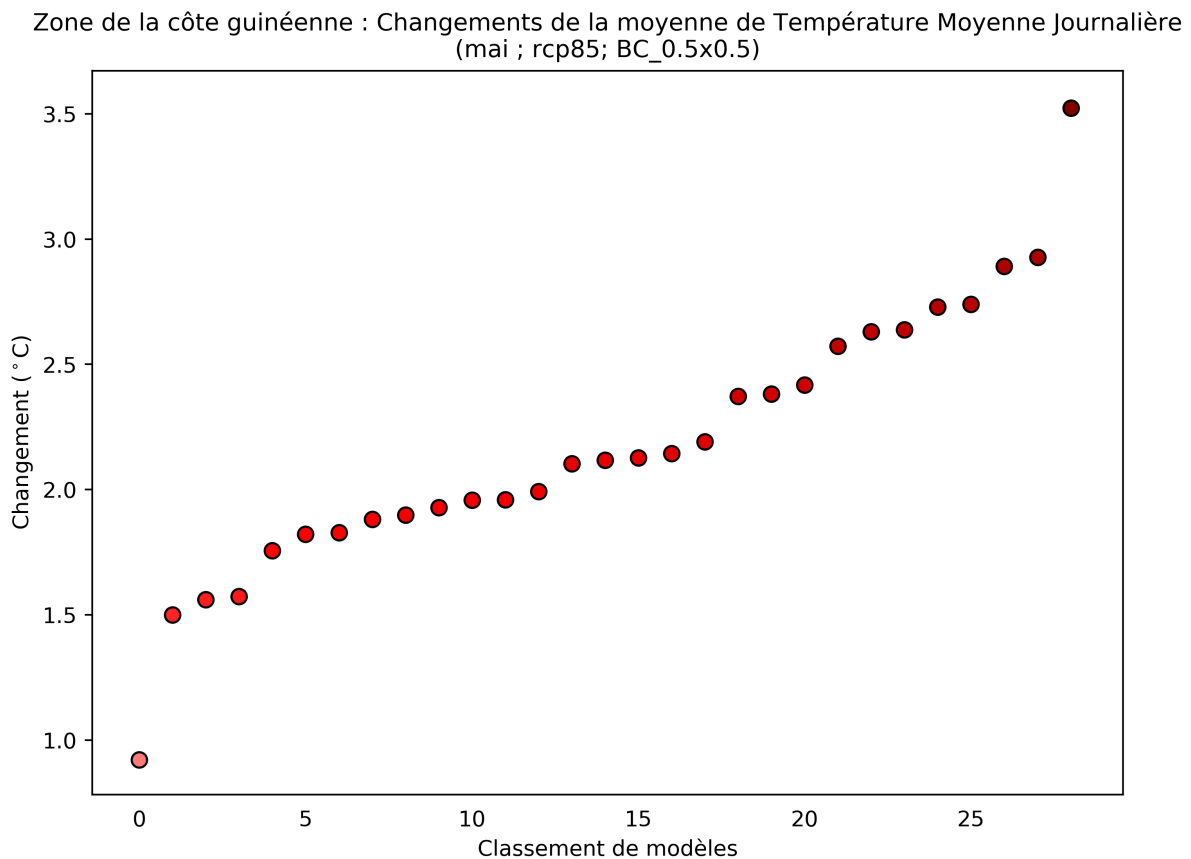
Figure 48: Ce diagramme de dispersion illustre la variation absolue de la moyenne de température moyenne journalière entre 2040 et 2059 (par rapport à la période de référence de 1950 à 2000) pour mai. Chaque point indique la moyenne spatiale d'un modèle sur Zone de la côte guinéenne; les points sont organisés ("rank", sur l'axe des abscisses) en fonction de la magnitude de leur valeur sur l'axe des ordonnées. Ce diagramme montre la variation absolue pour le scénario RCP8.5.
