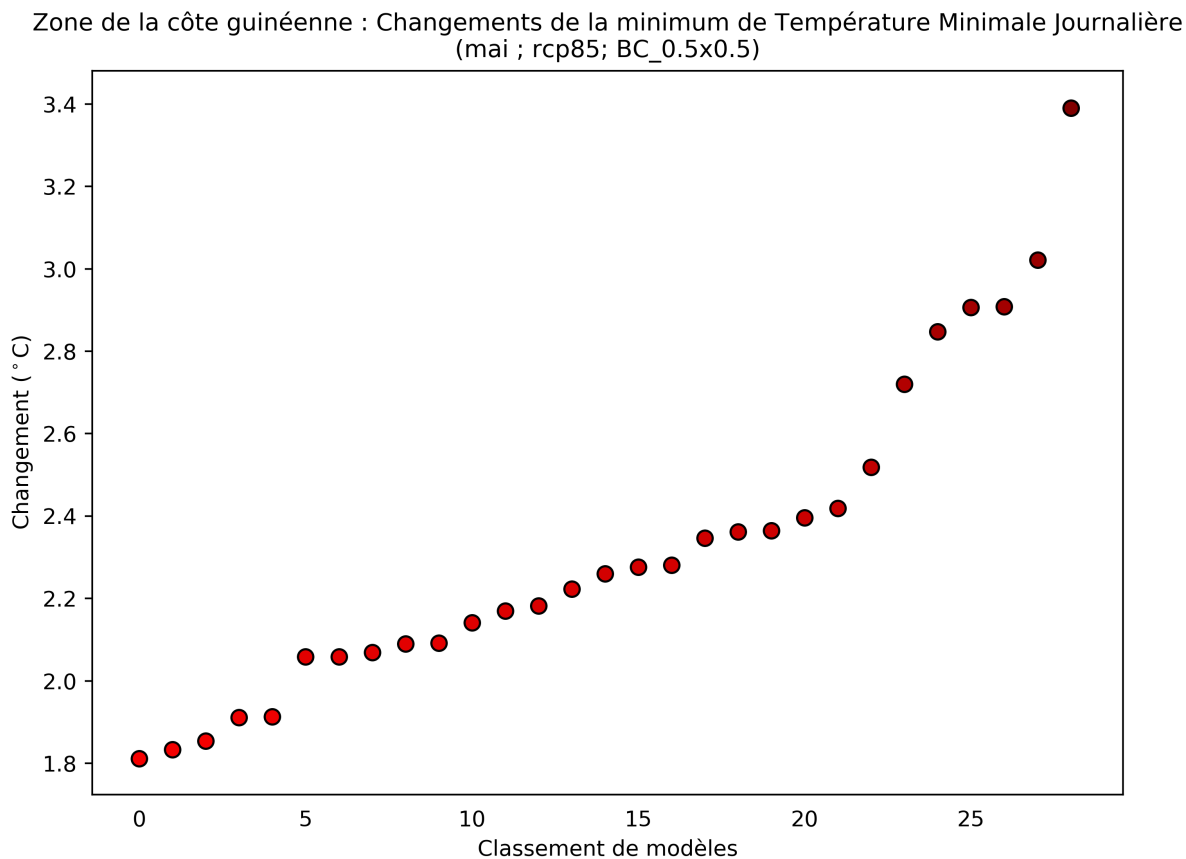
Figure 40: Ce diagramme de dispersion illustre la variation absolue de la minimum de température minimale journalière entre 2040 et 2059 (par rapport à la période de référence de 1950 à 2000) pour mai. Chaque point indique la moyenne spatiale d'un modèle sur Zone de la côte guinéenne; les points sont organisés ("rank", sur l'axe des abscisses) en fonction de la magnitude de leur valeur sur l'axe des ordonnées. Ce diagramme montre la variation absolue pour le scénario RCP8.5.
