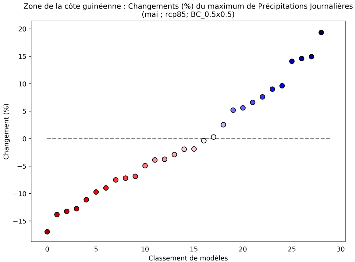
Figure 28: Ce diagramme de dispersion illustre du pourcentage de variation du maximum de précipitations journalières entre 2040 et 2059 (par rapport à la période de référence de 1950 à 2000) pour mai. Chaque point indique la moyenne spatiale d'un modèle sur Zone de la côte guinéenne; les points sont organisés ("rank", sur l'axe des abscisses) en fonction de la magnitude de leur valeur sur l'axe des ordonnées. Ce diagramme montre le pourcentage de variation pour le scénario RCP8.5.
