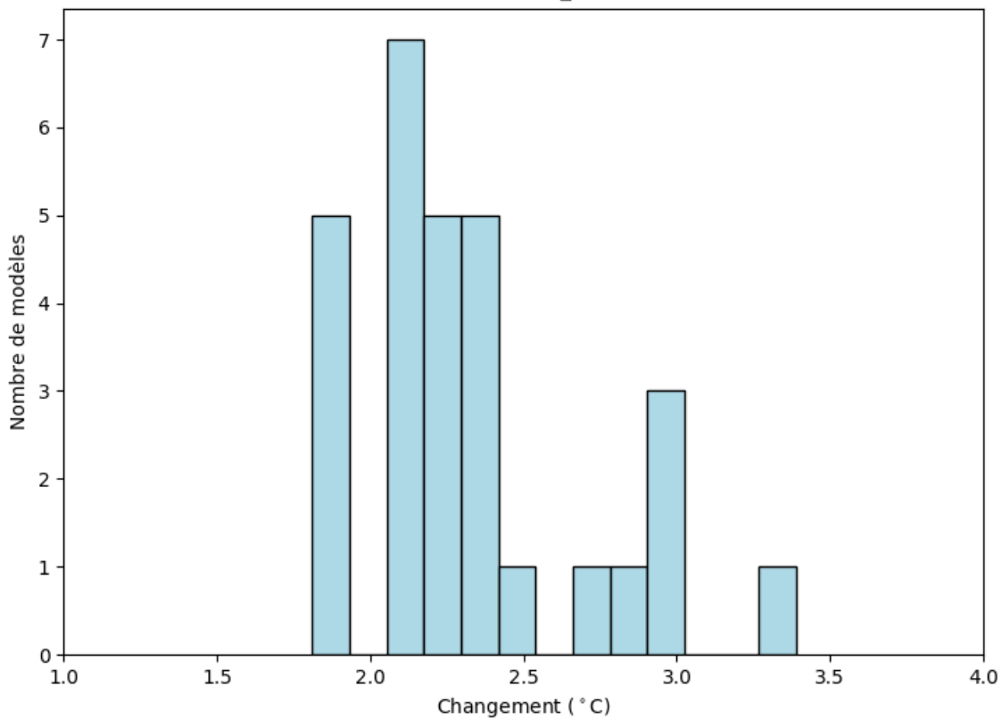
Zone de la côte guinéenne : Changements de la minimum de Température Minimale Journalière (mai ; rcp85; BC_0.5x0.5)
