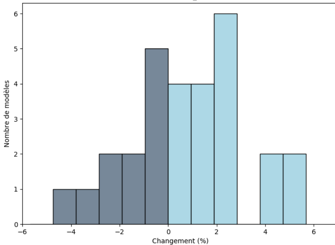
Zone de la côte guinéenne : Changements (%) de la moyenne de Flux Solaire Entrant À La Surface (mai ; rcp85; BC_0.5x0.5)
