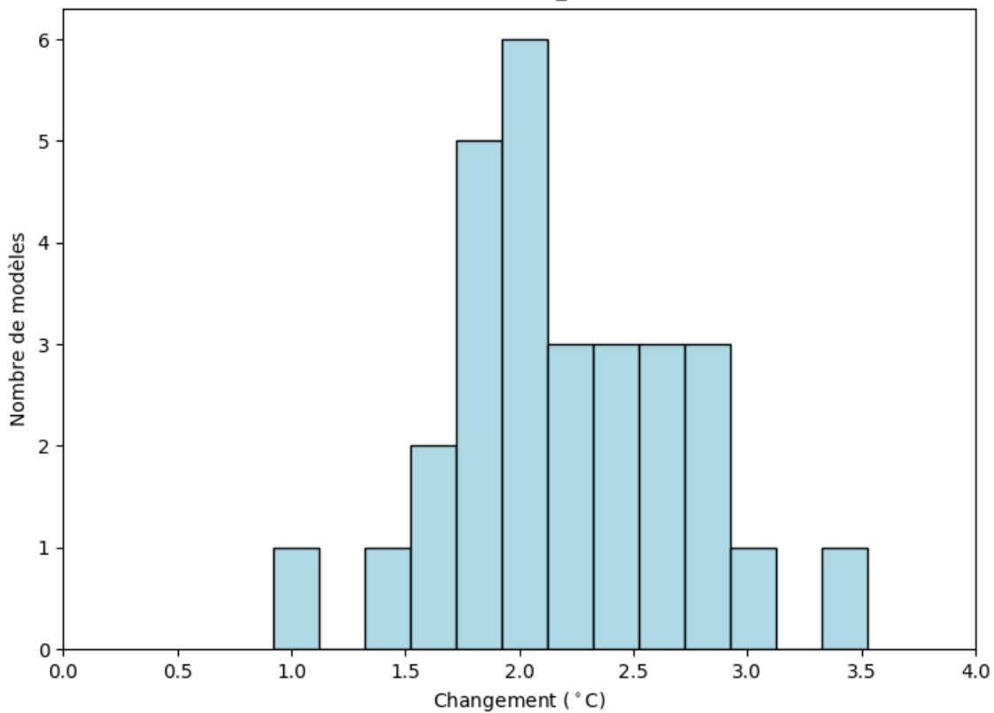
Zone de la côte guinéenne : Changements de la moyenne de Température Moyenne Journalière (mai ; rcp85; BC_0.5x0.5)
