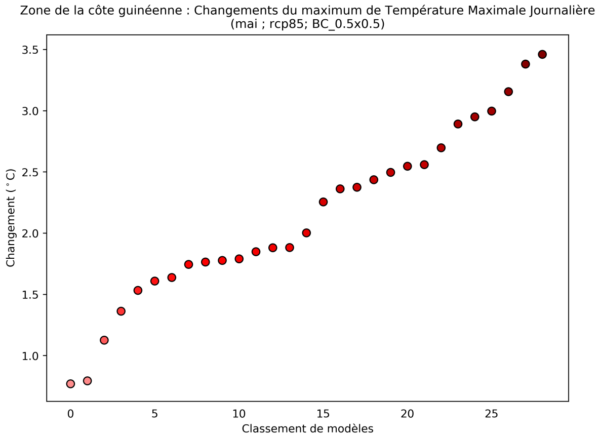
Figure 32: Ce diagramme de dispersion illustre la variation absolue du maximum de température maximale journalière entre 2040 et 2059 (par rapport à la période de référence de 1950 à 2000) pour mai. Chaque point indique la moyenne spatiale d'un modèle sur Zone de la côte guinéenne; les points sont organisés ("rank", sur l'axe des abscisses) en fonction de la magnitude de leur valeur sur l'axe des ordonnées. Ce diagramme montre la variation absolue pour le scénario RCP8.5.
