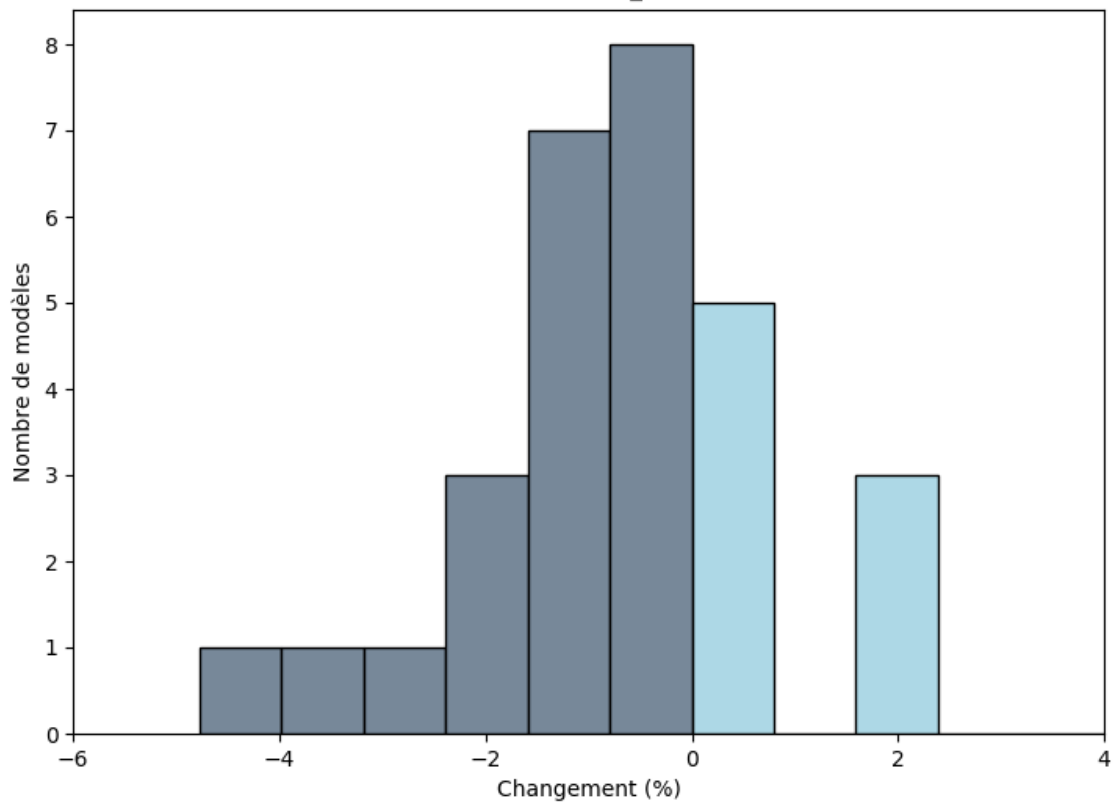
Zone de la côte guinéenne : Changements (%) du maximum de Flux Solaire Entrant À La Surface (mai ; rcp85; BC_0.5x0.5)
