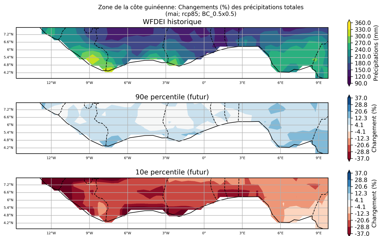
Figure 41: Ces cartes illustrent la projection multi-modèles pour du pourcentage de variation des précipitations totales, pour la période entre 2040 et 2059 (par rapport à la période de référence de 1950 à 2000) pour mai. Elles indiquent les 90ème et 10ème percentiles de la distribution des modèles dans l'ensemble multi-modèles, calculés séparément en chaque point de grille, sur la région Zone de la côte guinéenne. Ce diagramme montre le pourcentage de variation pour le scénario RCP8.5.
