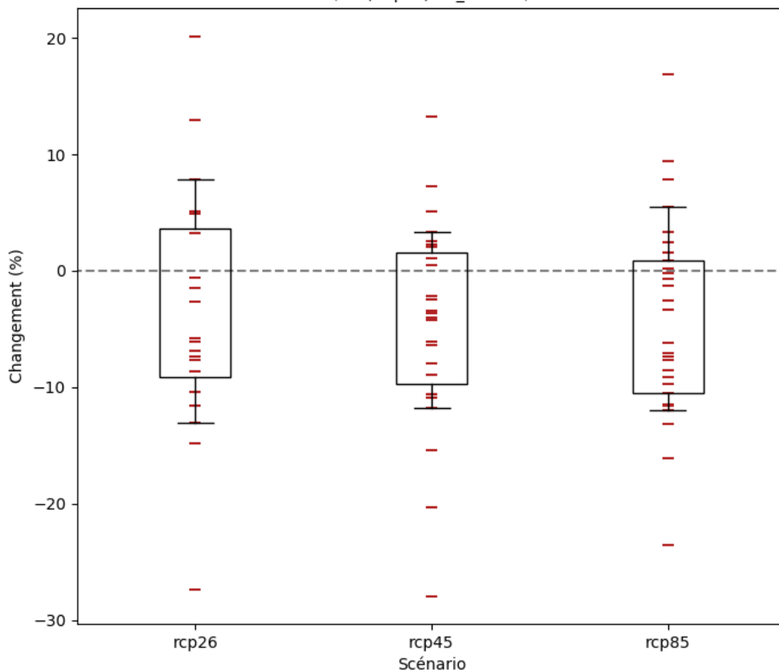
Zone de la côte guinéenne: Changements (%) du maximum de précipitations totales sur une période de 3 jours (mai; rcp85; BC_0.5x0.5)
