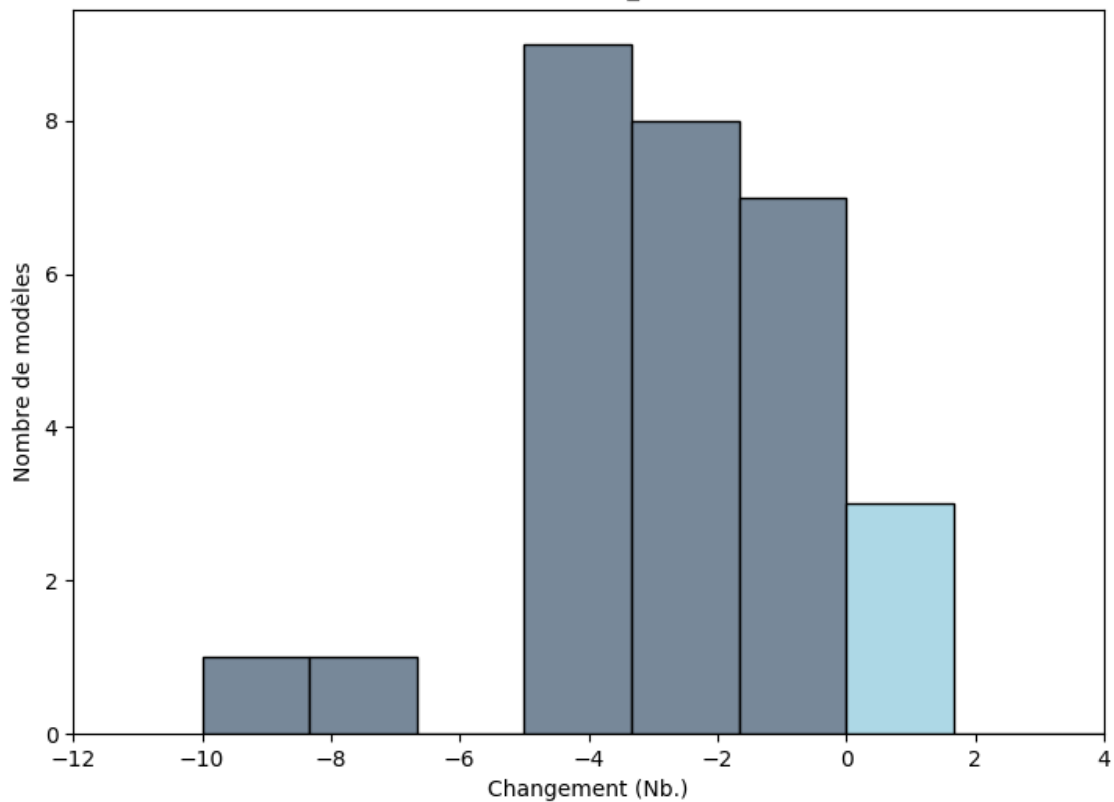
Zone de la côte guinéenne: Changements du nombre de séquences pluvieuses de plus de 10 jours (mai; rcp85; BC_0.5x0.5)
