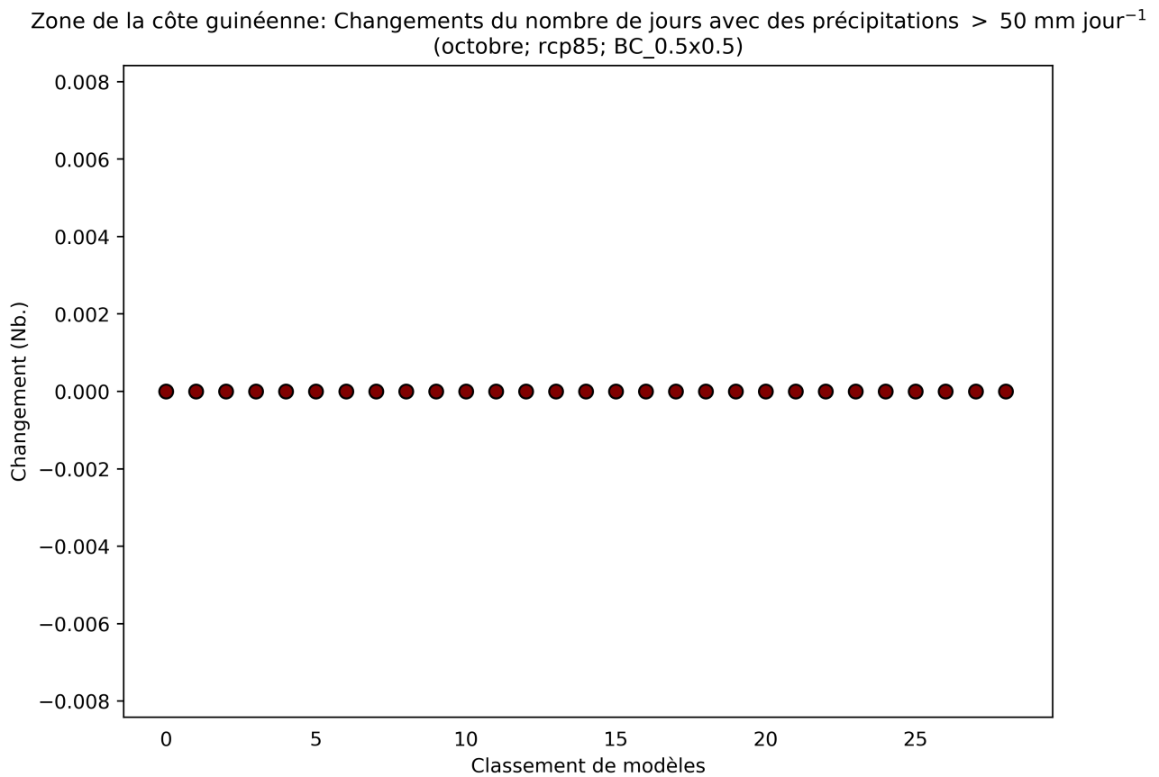
Figure 79: Ce diagramme de dispersion illustre la variation absolue du nombre de jours avec des précipitations > 50 \text{ mm jour}^{-1} entre 2040 et 2059 (par rapport à la période de référence de 1950 à 2000) pour octobre. Chaque point indique la moyenne spatiale d'un modèle sur Zone de la côte guinéenne; les points sont organisés ("rank", sur l'axe des abscisses) en fonction de la magnitude de leur valeur sur l'axe des ordonnées. Ce diagramme montre la variation absolue pour le scénario RCP8.5.
