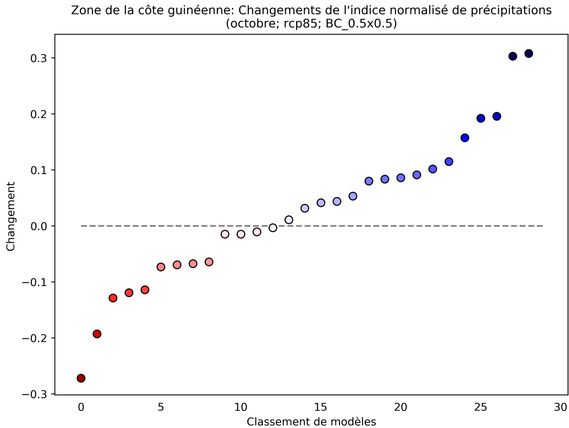
Figure 12: Ce diagramme de dispersion illustre la variation absolue de l'indice normalisé de précipitations entre 2040 et 2059 (par rapport à la période de référence de 1950 à 2000) pour octobre. Chaque point indique la moyenne spatiale d'un modèle sur Zone de la côte guinéenne; les points sont organisés ("rank", sur l'axe des abscisses) en fonction de la magnitude de leur valeur sur l'axe des ordonnées. Ce diagramme montre la variation absolue pour le scénario RCP8.5.
