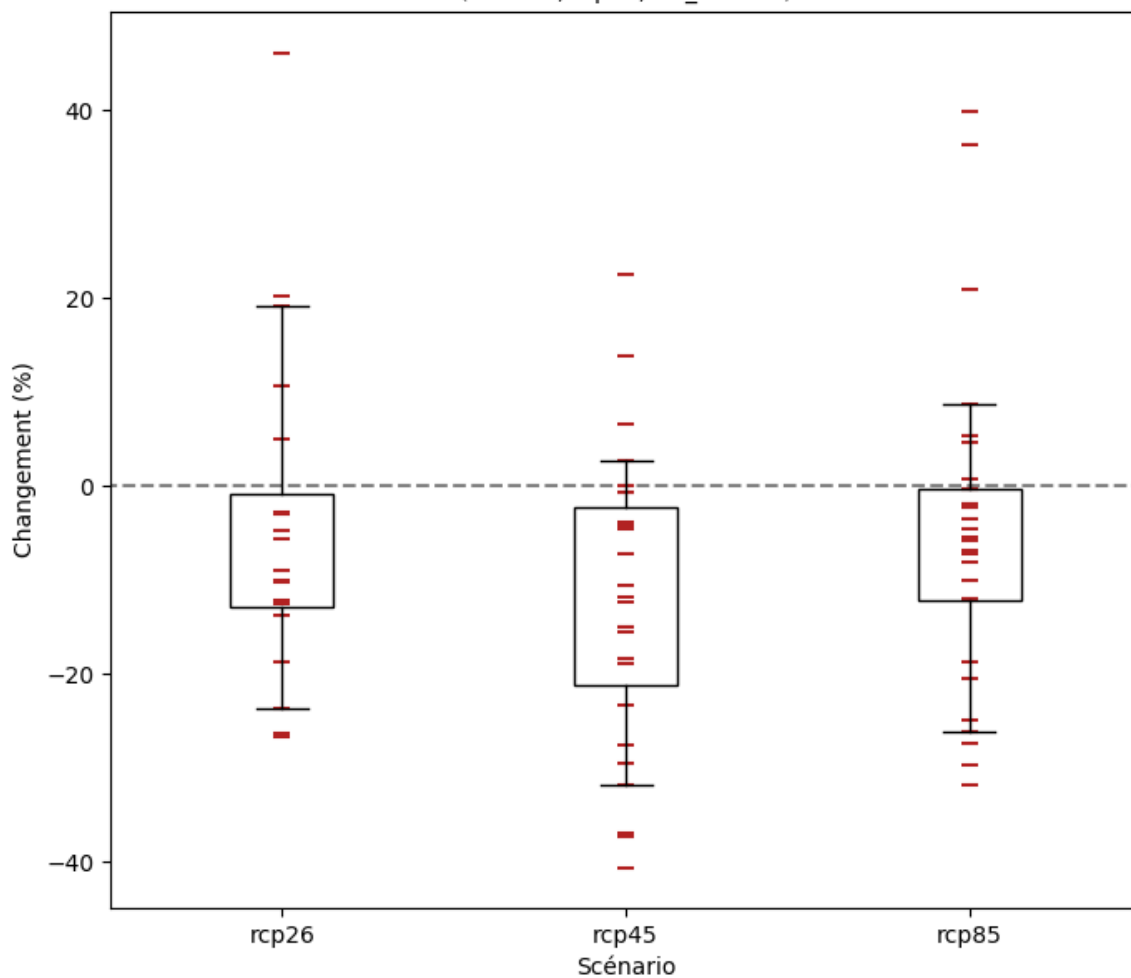
Zone de la côte guinéenne: Changements (%) du maximum de précipitations totales sur une période de 2 jours (octobre; rcp85; BC_0.5x0.5)
