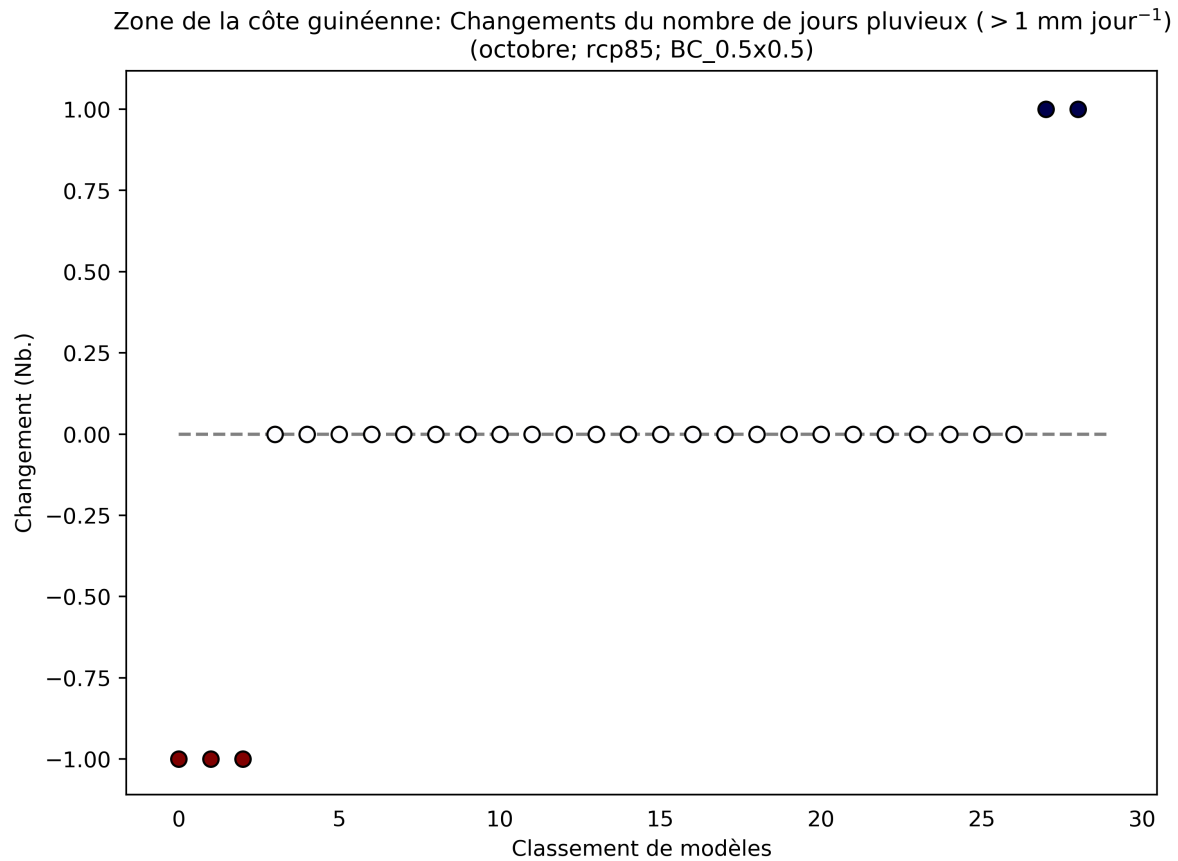
Figure 67: Ce diagramme de dispersion illustre la variation absolue du nombre de jours pluvieux ( >1 \text{ mm jour}^{-1} ) entre 2040 et 2059 (par rapport à la période de référence de 1950 à 2000) pour octobre. Chaque point indique la moyenne spatiale d'un modèle sur Zone de la côte guinéenne; les points sont organisés ("rank", sur l'axe des abscisses) en fonction de la magnitude de leur valeur sur l'axe des ordonnées. Ce diagramme montre la variation absolue pour le scénario RCP8.5.
