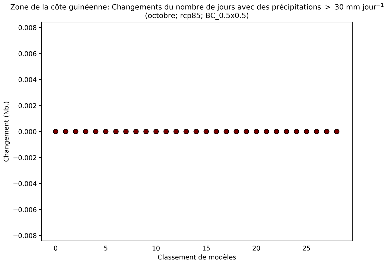
Figure 75: Ce diagramme de dispersion illustre la variation absolue du nombre de jours avec des précipitations > 30 \text{ mm jour}^{-1} entre 2040 et 2059 (par rapport à la période de référence de 1950 à 2000) pour octobre. Chaque point indique la moyenne spatiale d'un modèle sur Zone de la côte guinéenne; les points sont organisés ("rank", sur l'axe des abscisses) en fonction de la magnitude de leur valeur sur l'axe des ordonnées. Ce diagramme montre la variation absolue pour le scénario RCP8.5.
