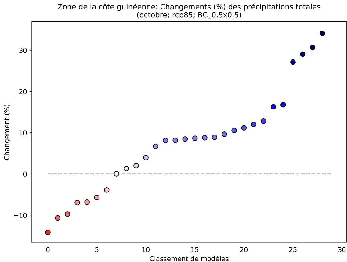
Figure 44: Ce diagramme de dispersion illustre du pourcentage de variation des précipitations totales entre 2040 et 2059 (par rapport à la période de référence de 1950 à 2000) pour octobre. Chaque point indique la moyenne spatiale d'un modèle sur Zone de la côte guinéenne; les points sont organisés ("rank", sur l'axe des abscisses) en fonction de la magnitude de leur valeur sur l'axe des ordonnées. Ce diagramme montre le pourcentage de variation pour le scénario RCP8.5.
