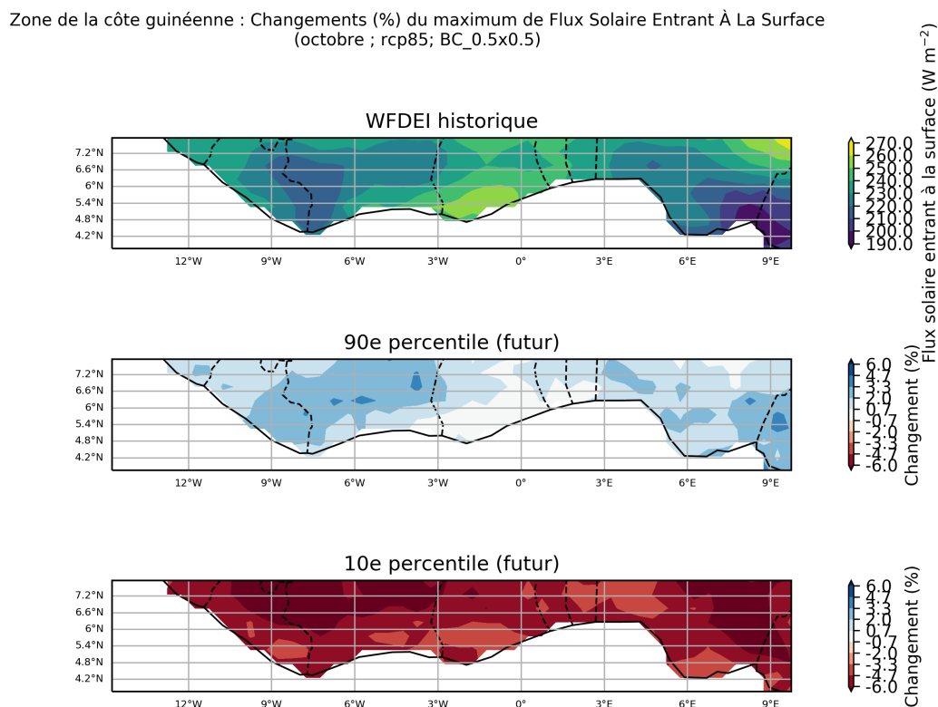
Figure 33: Ces cartes illustrent la projection multi-modèles pour du pourcentage de variation du maximum de flux solaire entrant à la surface, pour la période entre 2040 et 2059 (par rapport à la période de référence de 1950 à 2000) pour octobre. Elles indiquent les 90ème et 10ème percentiles de la distribution des modèles dans l'ensemble multi-modèles, calculés séparément en chaque point de grille, sur la région Zone de la côte guinéenne. Ce diagramme montre le pourcentage de variation pour le scénario RCP8.5.
