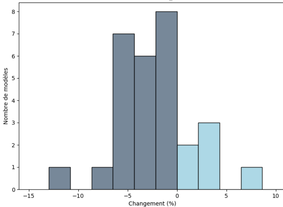
Zone de la côte guinéenne : Changements (%) de la moyenne de Flux Solaire Entrant À La Surface (octobre ; rcp85; BC_0.5x0.5)
