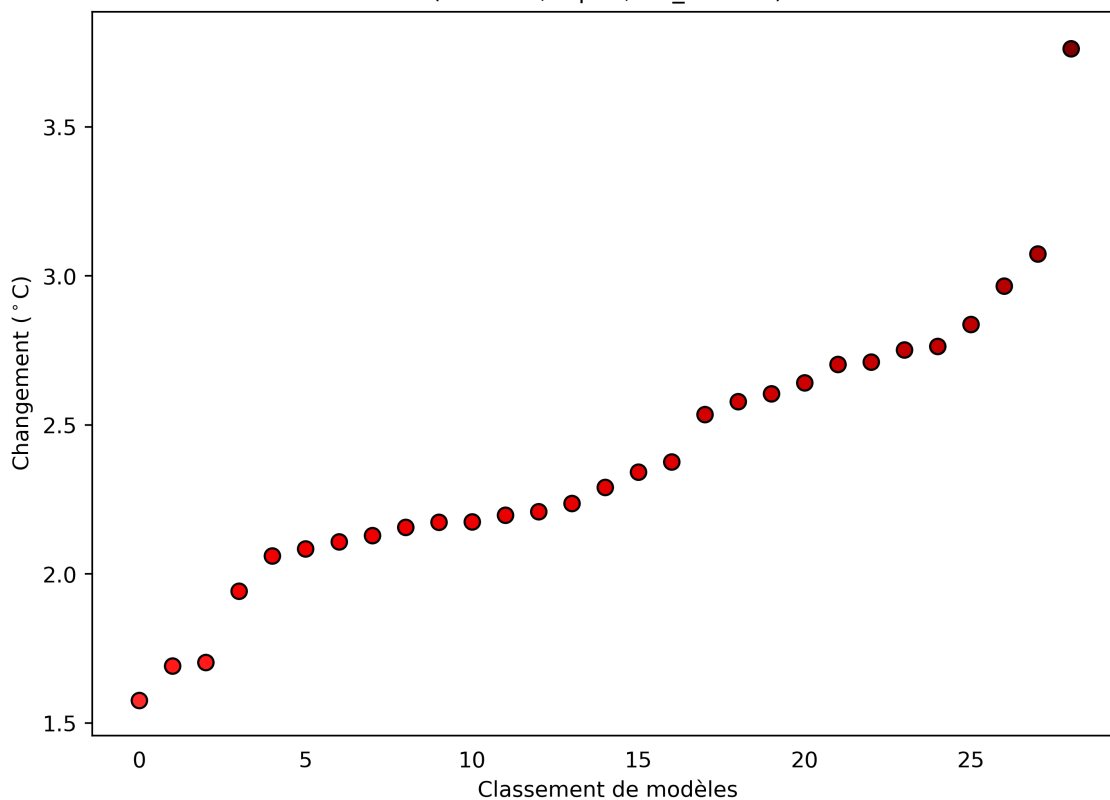
Figure 40: Ce diagramme de dispersion illustre la variation absolue de la minimum de température minimale journalière entre 2040 et 2059 (par rapport à la période de référence de 1950 à 2000) pour octobre. Chaque point indique la moyenne spatiale d'un modèle sur Zone de la côte guinéenne; les points sont organisés ("rank", sur l'axe des abscisses) en fonction de la magnitude de leur valeur sur l'axe des ordonnées. Ce diagramme montre la variation absolue pour le scénario RCP8.5.
