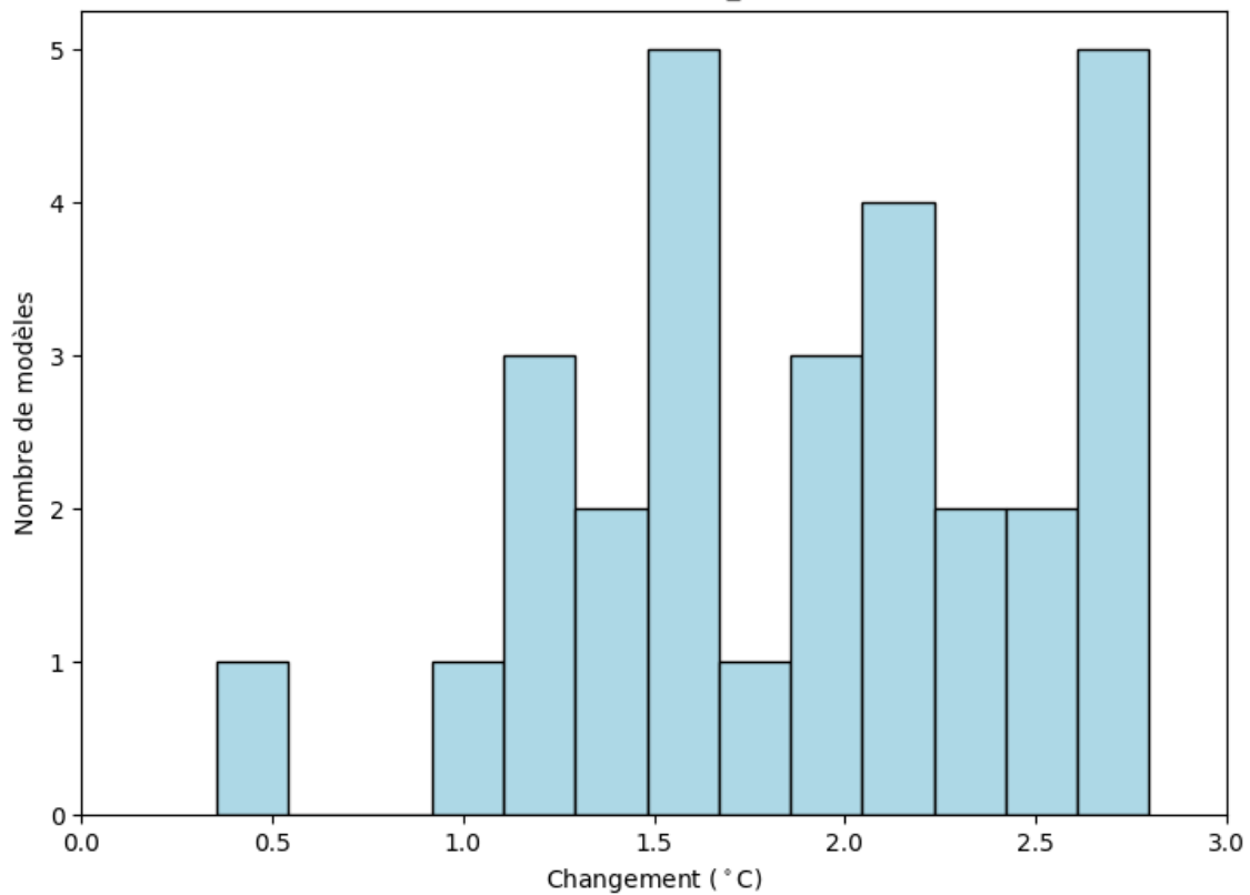
Zone de la côte guinéenne : Changements du maximum de Température Maximale Journalière (octobre ; rcp85; BC_0.5x0.5)
