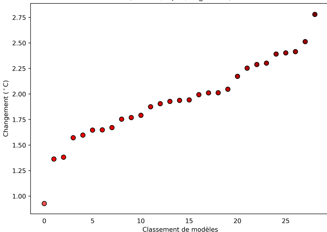
Zone de la côte guinéenne : Changements de la moyenne de Température Moyenne Journalière (octobre ; rcp85; BC_0.5x0.5)
