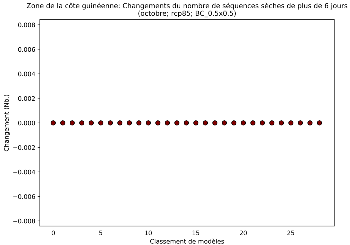
Figure 24: Ce diagramme de dispersion illustre la variation absolue du nombre de séquences sèches de plus de 6 jours entre 2040 et 2059 (par rapport à la période de référence de 1950 à 2000) pour octobre. Chaque point indique la moyenne spatiale d'un modèle sur Zone de la côte guinéenne; les points sont organisés ("rank", sur l'axe des abscisses) en fonction de la magnitude de leur valeur sur l'axe des ordonnées. Ce diagramme montre la variation absolue pour le scénario RCP8.5.
