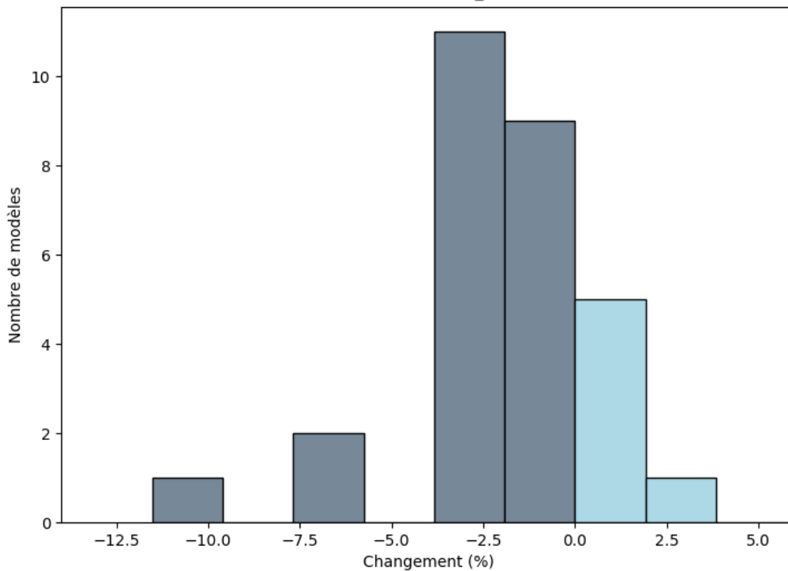
Zone de la côte guinéenne : Changements (%) du maximum de Flux Solaire Entrant À La Surface (octobre ; rcp85; BC_0.5x0.5)
