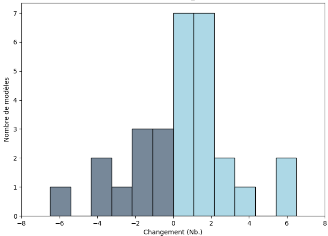
Zone de la côte guinéenne: Changements du nombre de séquences pluvieuses de plus de 10 jours (octobre; rcp85; BC_0.5x0.5)
