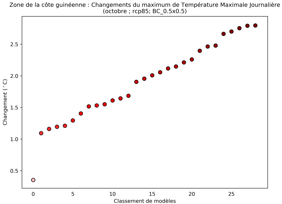
Figure 32: Ce diagramme de dispersion illustre la variation absolue du maximum de température maximale journalière entre 2040 et 2059 (par rapport à la période de référence de 1950 à 2000) pour octobre. Chaque point indique la moyenne spatiale d'un modèle sur Zone de la côte guinéenne; les points sont organisés ("rank", sur l'axe des abscisses) en fonction de la magnitude de leur valeur sur l'axe des ordonnées. Ce diagramme montre la variation absolue pour le scénario RCP8.5.
