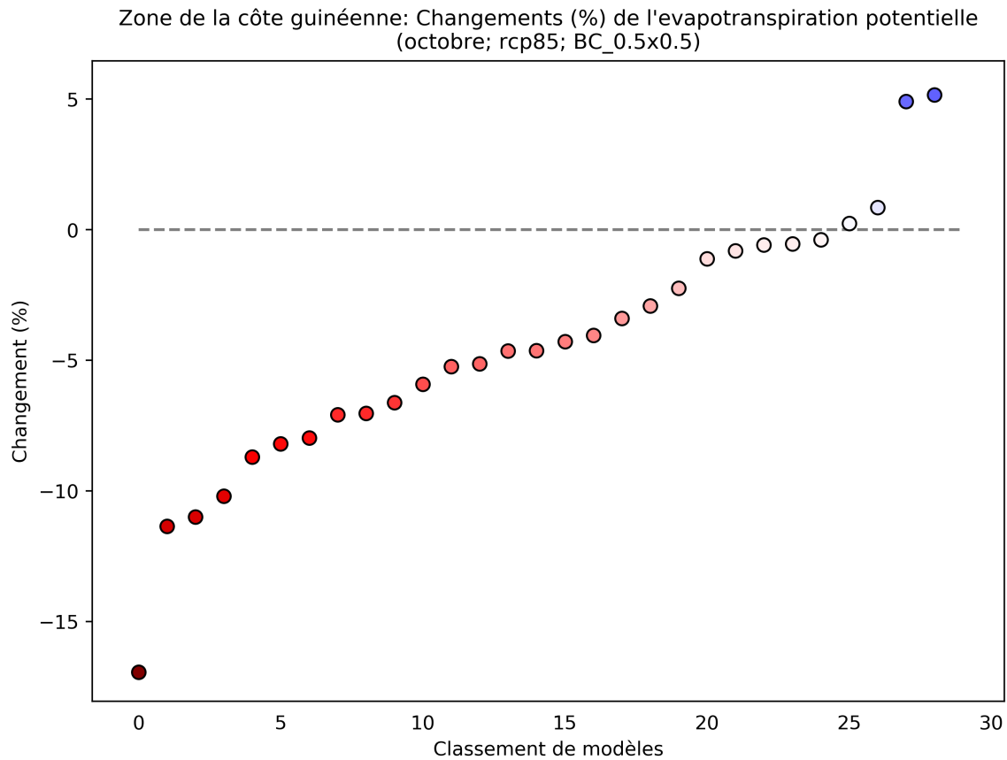
Figure 4: Ce diagramme de dispersion illustre du pourcentage de variation de l'évapotranspiration potentielle entre 2040 et 2059 (par rapport à la période de référence de 1950 à 2000) pour octobre. Chaque point indique la moyenne spatiale d'un modèle sur Zone de la côte guinéenne; les points sont organisés ("rank", sur l'axe des abscisses) en fonction de la magnitude de leur valeur sur l'axe des ordonnées. Ce diagramme montre le pourcentage de variation pour le scénario RCP8.5.
