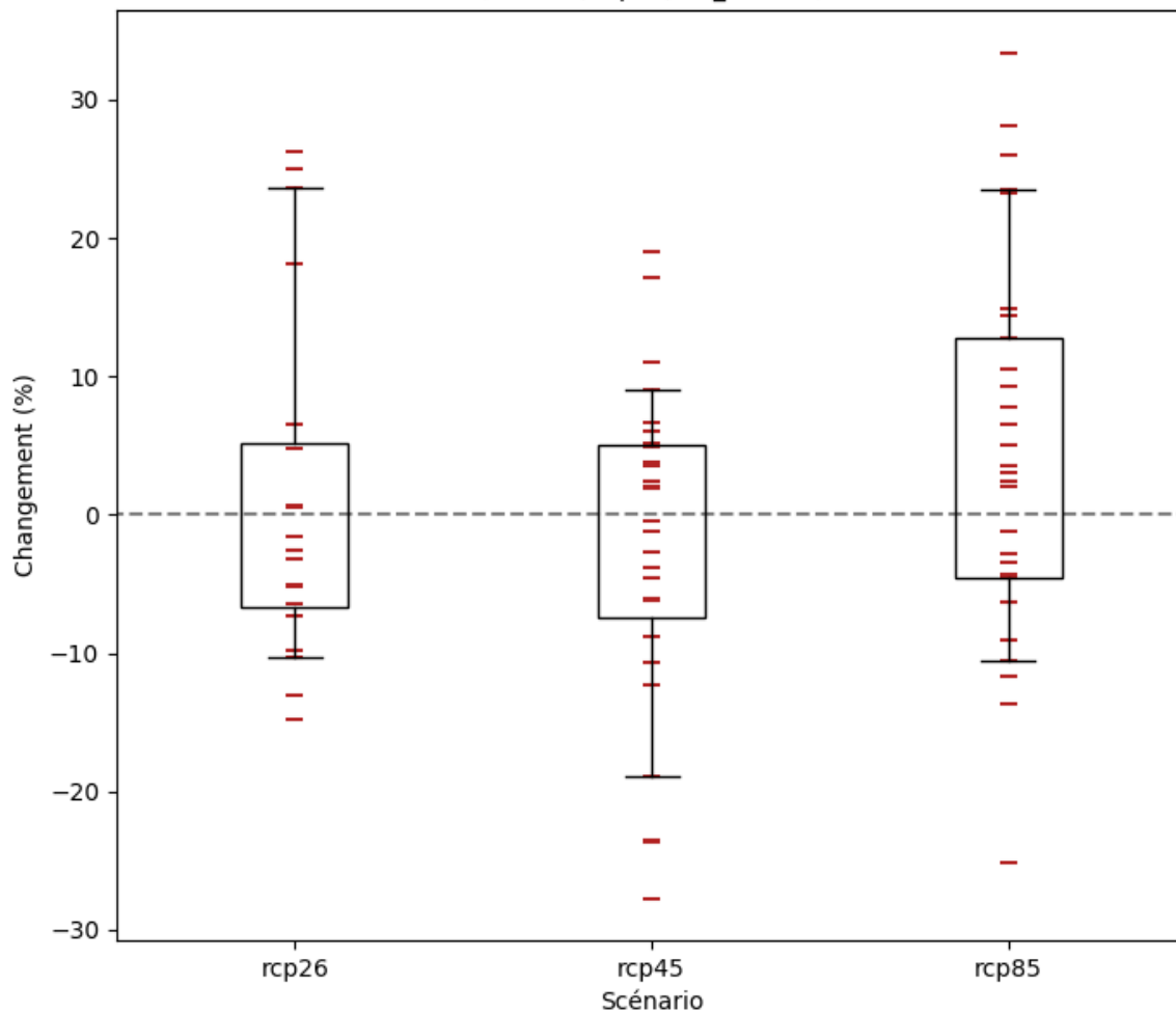
Zone de la côte guinéenne: Changements (%) du maximum de précipitations totales sur une période de 3 jours (octobre; rcp85; BC_0.5x0.5)
