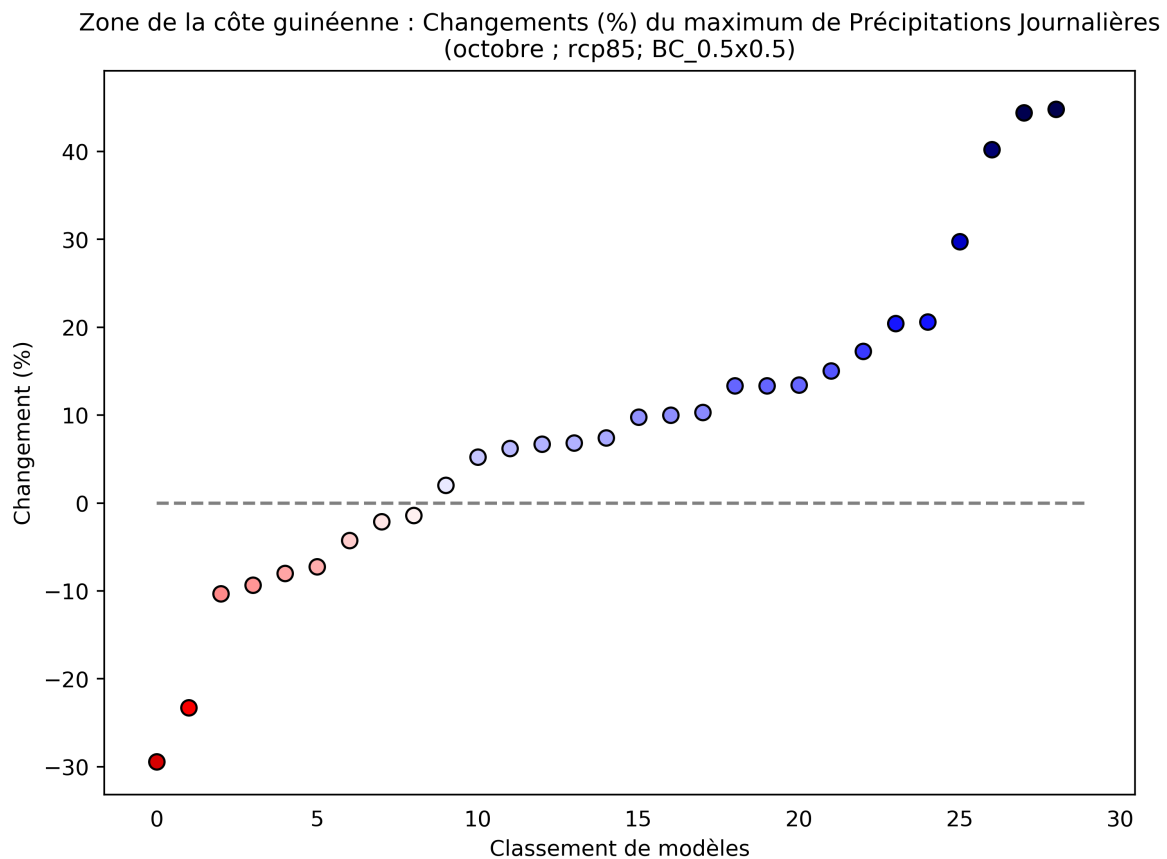
Figure 28: Ce diagramme de dispersion illustre du pourcentage de variation du maximum de précipitations journalières entre 2040 et 2059 (par rapport à la période de référence de 1950 à 2000) pour octobre. Chaque point indique la moyenne spatiale d'un modèle sur Zone de la côte guinéenne; les points sont organisés ("rank", sur l'axe des abscisses) en fonction de la magnitude de leur valeur sur l'axe des ordonnées. Ce diagramme montre le pourcentage de variation pour le scénario RCP8.5.
