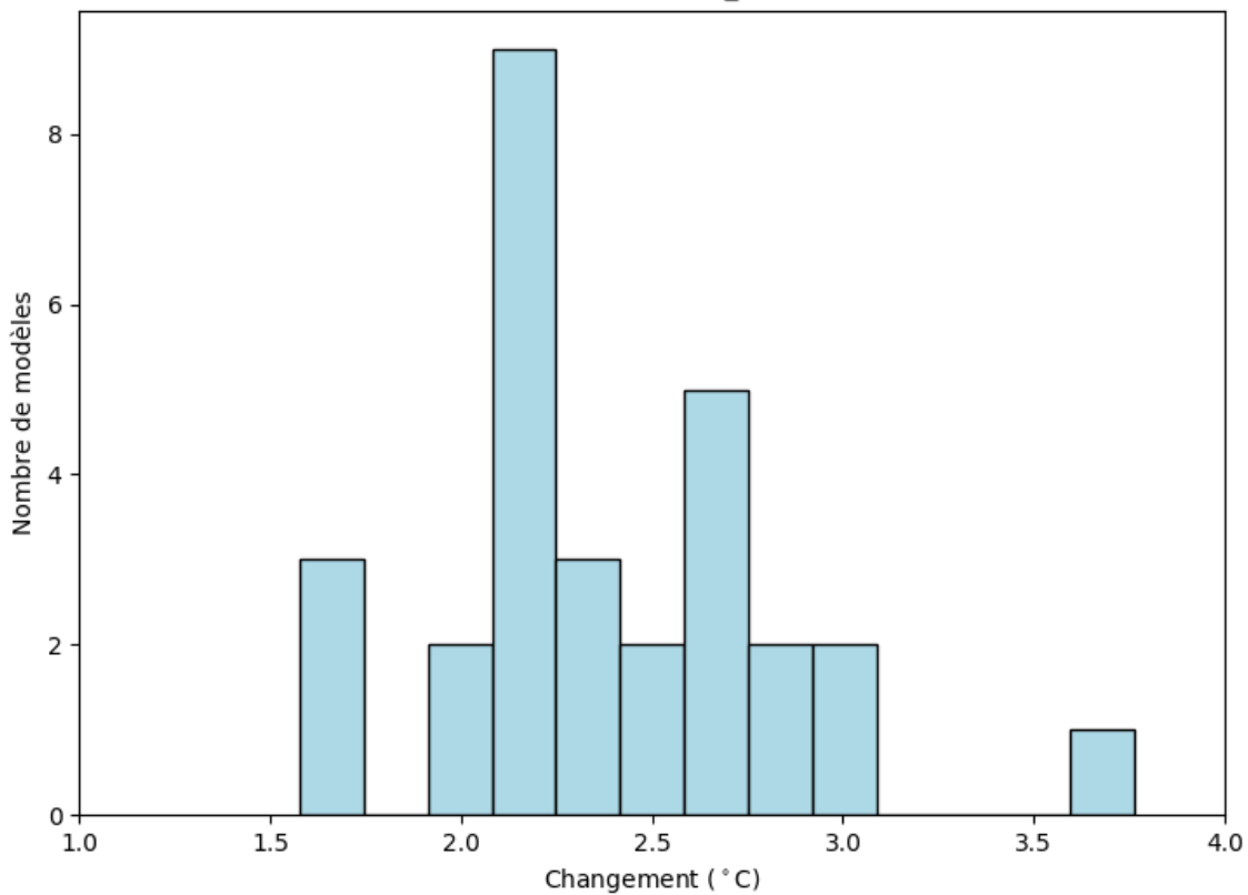
Zone de la côte guinéenne : Changements de la minimum de Température Minimale Journalière (octobre ; rcp85; BC_0.5x0.5)
