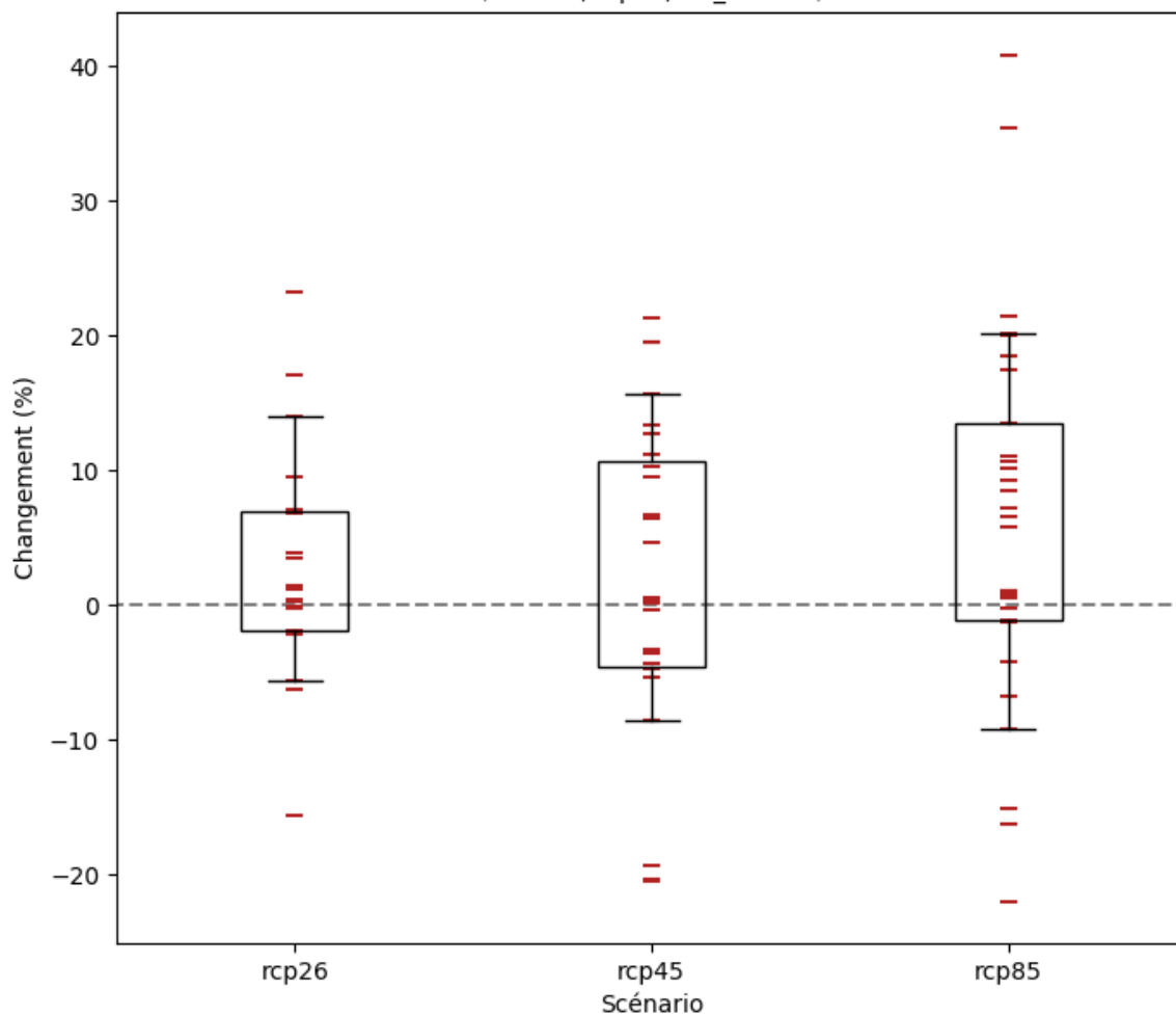
Zone de la côte guinéenne: Changements (%) du maximum de précipitations totales sur une période de 5 jours (octobre; rcp85; BC_0.5x0.5)
