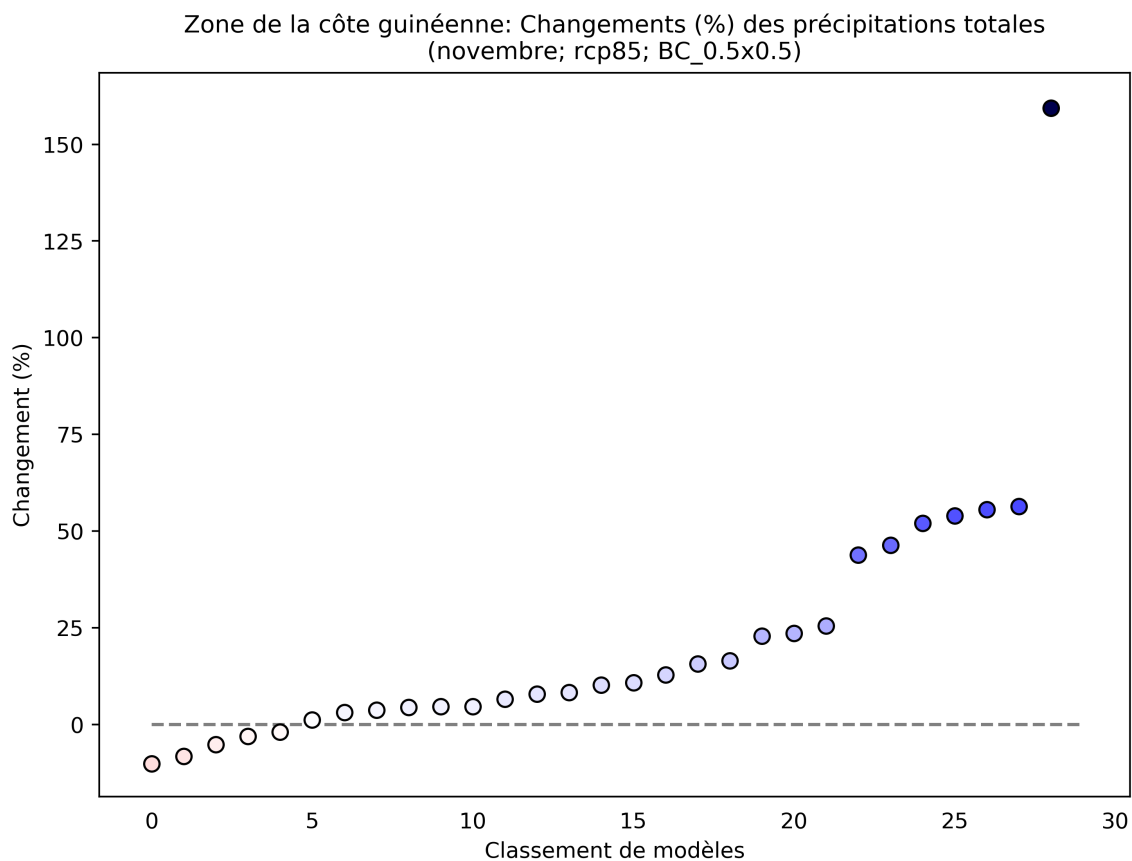
Figure 44: Ce diagramme de dispersion illustre du pourcentage de variation des précipitations totales entre 2040 et 2059 (par rapport à la période de référence de 1950 à 2000) pour novembre. Chaque point indique la moyenne spatiale d'un modèle sur Zone de la côte guinéenne; les points sont organisés ("rank", sur l'axe des abscisses) en fonction de la magnitude de leur valeur sur l'axe des ordonnées. Ce diagramme montre le pourcentage de variation pour le scénario RCP8.5.
