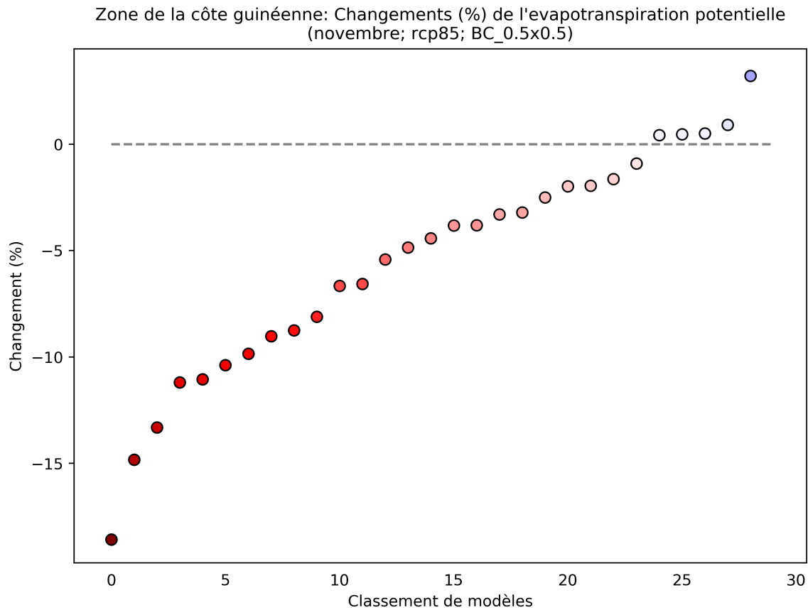
Figure 4: Ce diagramme de dispersion illustre du pourcentage de variation de l'évapotranspiration potentielle entre 2040 et 2059 (par rapport à la période de référence de 1950 à 2000) pour novembre. Chaque point indique la moyenne spatiale d'un modèle sur Zone de la côte guinéenne; les points sont organisés ("rank", sur l'axe des abscisses) en fonction de la magnitude de leur valeur sur l'axe des ordonnées. Ce diagramme montre le pourcentage de variation pour le scénario RCP8.5.
