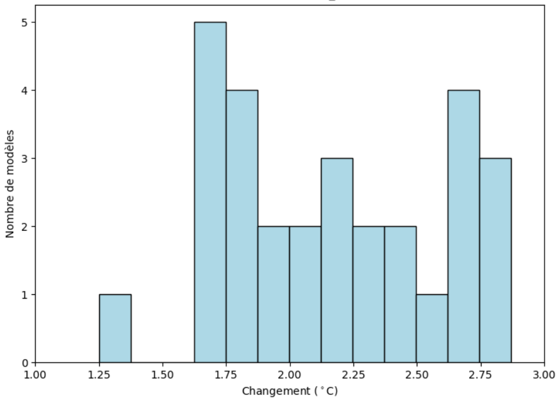
Zone de la côte guinéenne : Changements de la moyenne de Température Moyenne Journalière (novembre ; rcp85; BC_0.5x0.5)
