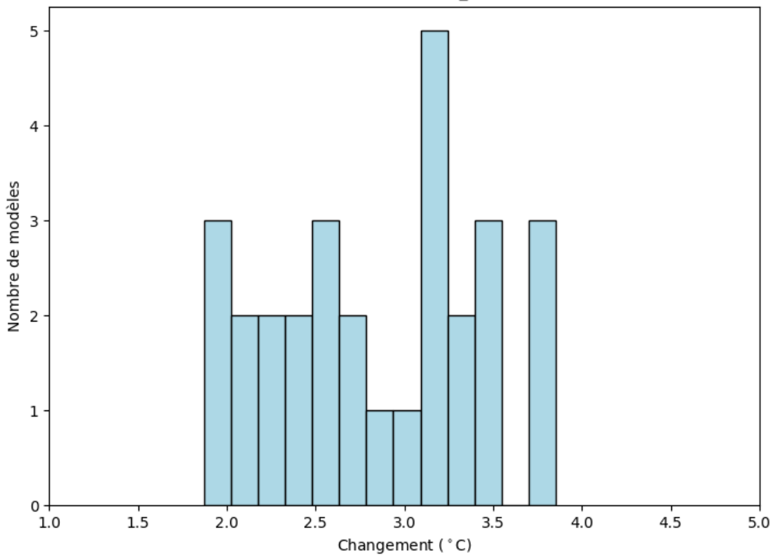
Zone de la côte guinéenne : Changements de la minimum de Température Minimale Journalière (novembre ; rcp85; BC_0.5x0.5)
