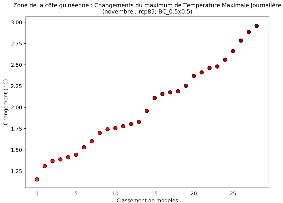
Figure 32: Ce diagramme de dispersion illustre la variation absolue du maximum de température maximale journalière entre 2040 et 2059 (par rapport à la période de référence de 1950 à 2000) pour novembre. Chaque point indique la moyenne spatiale d'un modèle sur Zone de la côte guinéenne; les points sont organisés ("rank", sur l'axe des abscisses) en fonction de la magnitude de leur valeur sur l'axe des ordonnées. Ce diagramme montre la variation absolue pour le scénario RCP8.5.
