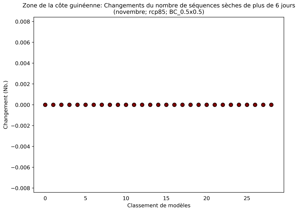
Figure 24: Ce diagramme de dispersion illustre la variation absolue du nombre de séquences sèches de plus de 6 jours entre 2040 et 2059 (par rapport à la période de référence de 1950 à 2000) pour novembre. Chaque point indique la moyenne spatiale d'un modèle sur Zone de la côte guinéenne; les points sont organisés ("rank", sur l'axe des abscisses) en fonction de la magnitude de leur valeur sur l'axe des ordonnées. Ce diagramme montre la variation absolue pour le scénario RCP8.5.
