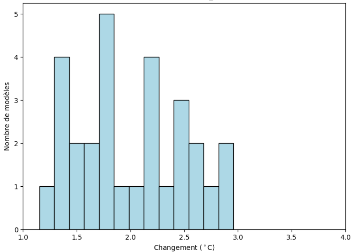
Zone de la côte guinéenne : Changements du maximum de Température Maximale Journalière (novembre ; rcp85; BC_0.5x0.5)
