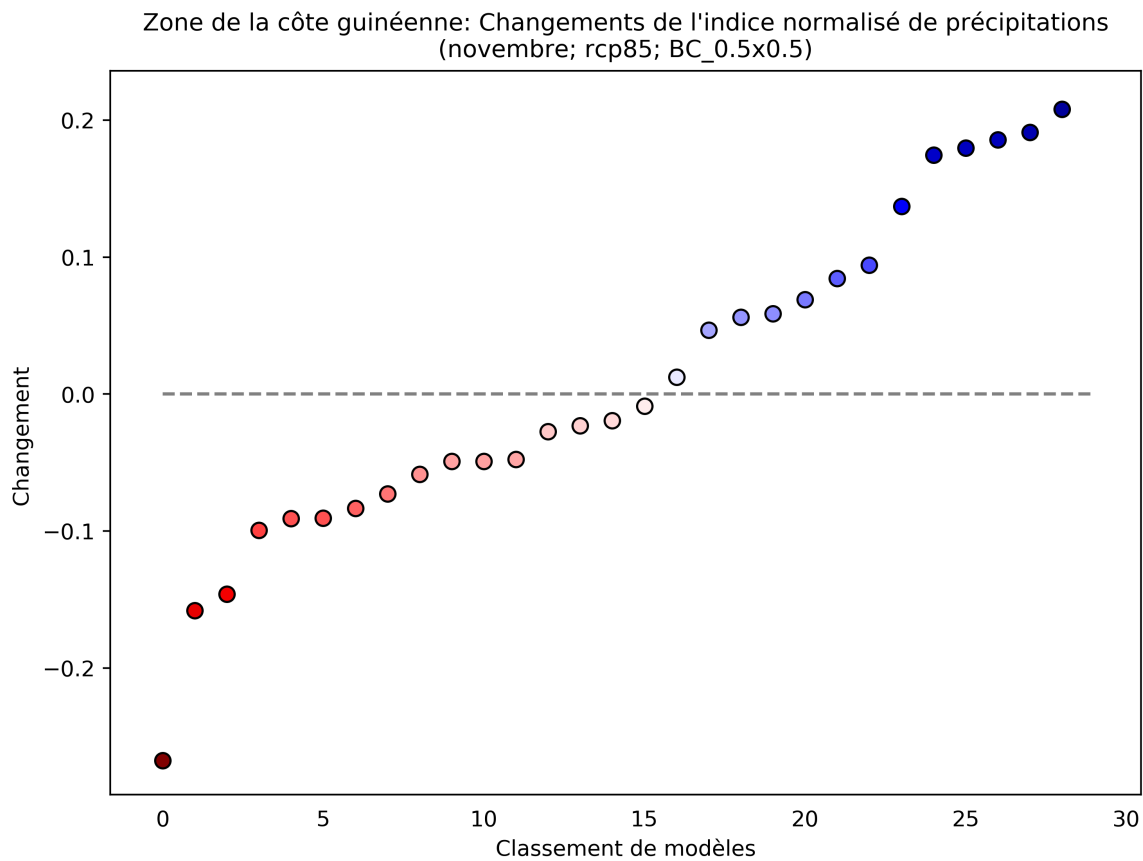
Figure 12: Ce diagramme de dispersion illustre la variation absolue de l'indice normalisé de précipitations entre 2040 et 2059 (par rapport à la période de référence de 1950 à 2000) pour novembre. Chaque point indique la moyenne spatiale d'un modèle sur Zone de la côte guinéenne; les points sont organisés ("rank", sur l'axe des abscisses) en fonction de la magnitude de leur valeur sur l'axe des ordonnées. Ce diagramme montre la variation absolue pour le scénario RCP8.5.
