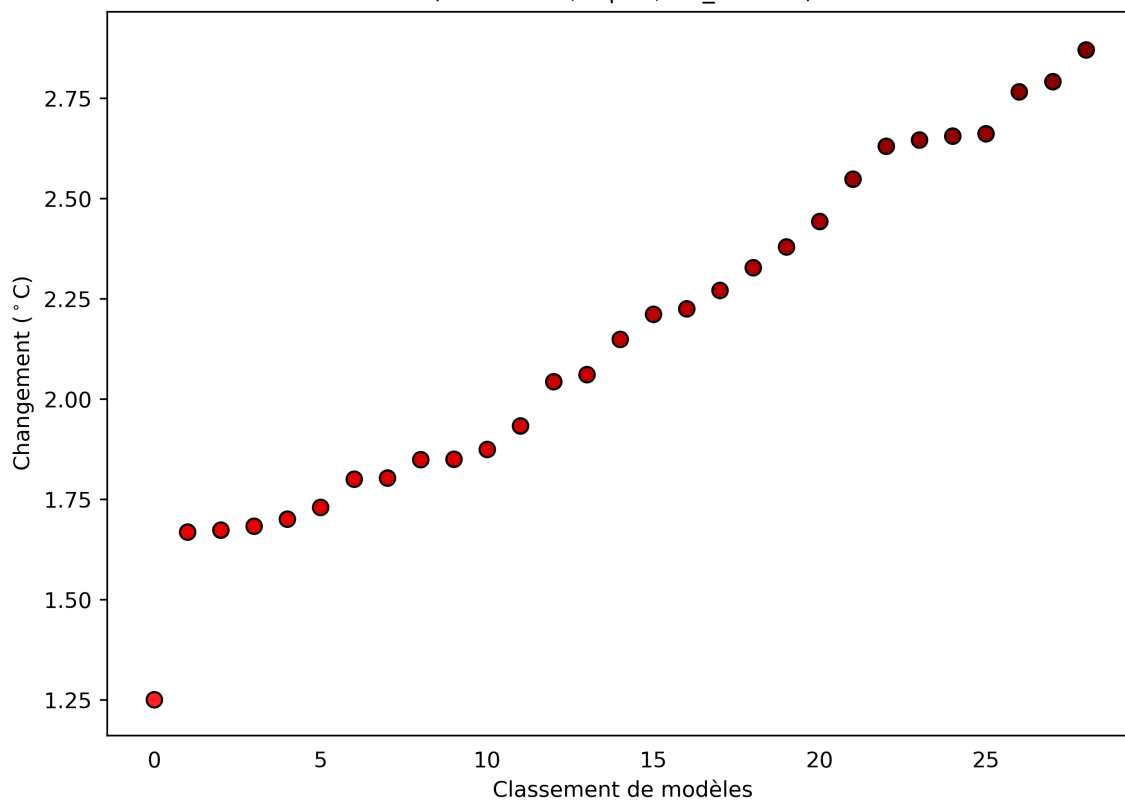
Figure 48: Ce diagramme de dispersion illustre la variation absolue de la moyenne de température moyenne journalière entre 2040 et 2059 (par rapport à la période de référence de 1950 à 2000) pour novembre. Chaque point indique la moyenne spatiale d'un modèle sur Zone de la côte guinéenne; les points sont organisés ("rank", sur l'axe des abscisses) en fonction de la magnitude de leur valeur sur l'axe des ordonnées. Ce diagramme montre la variation absolue pour le scénario RCP8.5.
