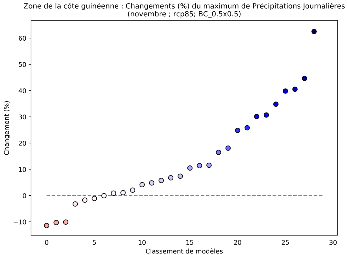
Figure 28: Ce diagramme de dispersion illustre du pourcentage de variation du maximum de précipitations journalières entre 2040 et 2059 (par rapport à la période de référence de 1950 à 2000) pour novembre. Chaque point indique la moyenne spatiale d'un modèle sur Zone de la côte guinéenne; les points sont organisés ("rank", sur l'axe des abscisses) en fonction de la magnitude de leur valeur sur l'axe des ordonnées. Ce diagramme montre le pourcentage de variation pour le scénario RCP8.5.
