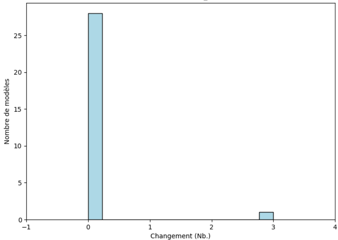
Figure 18: Cet histogramme illustre le nombre de modèles en accord avec la variation absolue du nombre de séquences pluvieuses de plus de 10 jours pour la période entre 2040 et 2059 (par rapport à la période de référence de 1950 à 2000) pour novembre. Chaque barre verticale indique le nombre de modèles en accord avec la gamme de valeur indiquée sur l'axe des abscisses pour la région Zone de la côte guinéenne. Ce diagramme montre la variation absolue pour le scénario RCP8.5.
