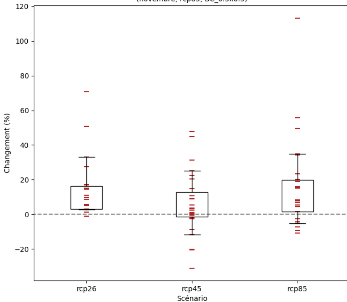
Zone de la côte guinéenne: Changements (%) du maximum de précipitations totales sur une période de 5 jours (novembre; rcp85; BC_0.5x0.5)
