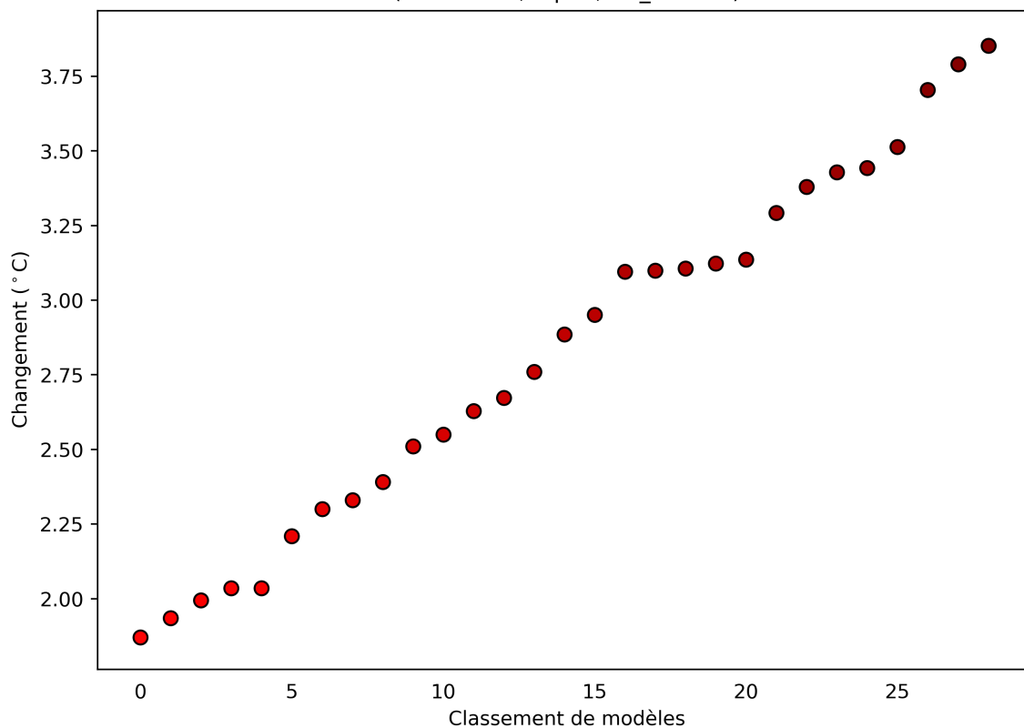
Figure 40: Ce diagramme de dispersion illustre la variation absolue de la minimum de température minimale journalière entre 2040 et 2059 (par rapport à la période de référence de 1950 à 2000) pour novembre. Chaque point indique la moyenne spatiale d'un modèle sur Zone de la côte guinéenne; les points sont organisés ("rank", sur l'axe des abscisses) en fonction de la magnitude de leur valeur sur l'axe des ordonnées. Ce diagramme montre la variation absolue pour le scénario RCP8.5.
