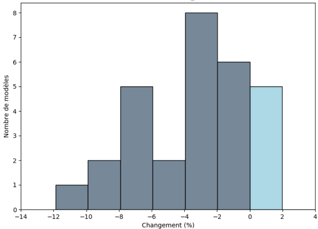
Zone de la côte guinéenne : Changements (%) de la moyenne de Flux Solaire Entrant À La Surface (novembre ; rcp85; BC_0.5x0.5)
