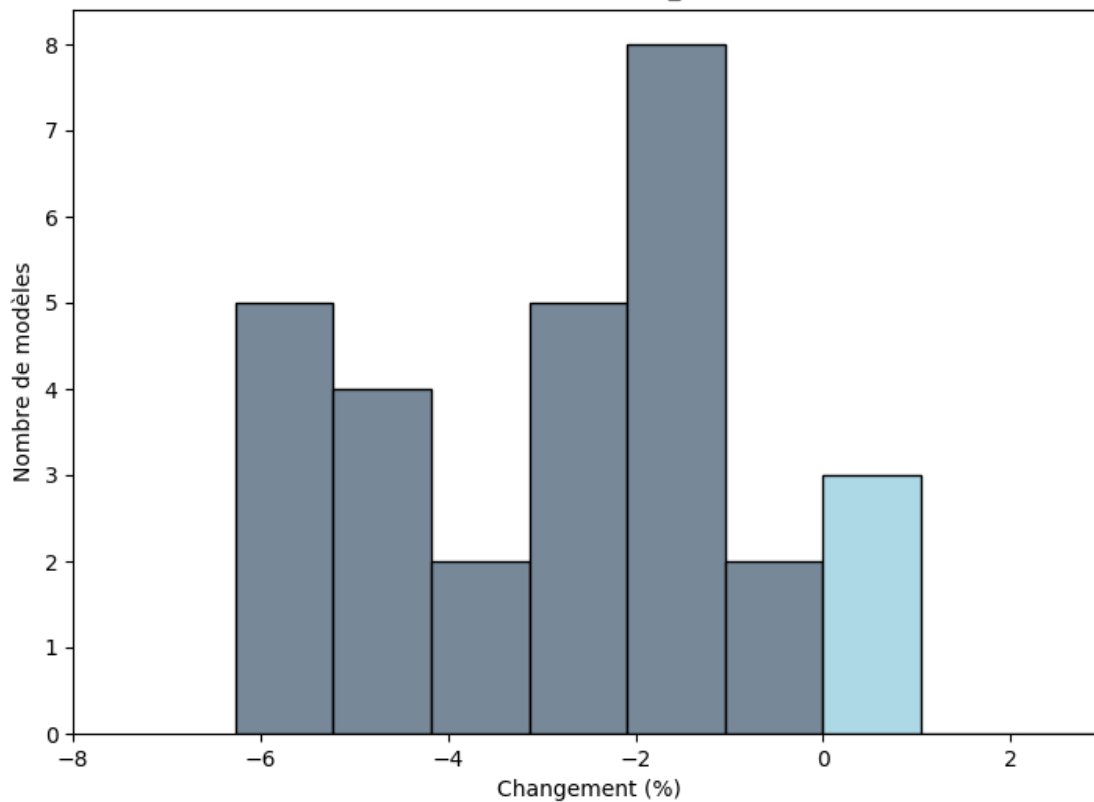
Zone de la côte guinéenne : Changements (%) du maximum de Flux Solaire Entrant À La Surface (novembre ; rcp85; BC_0.5x0.5)
