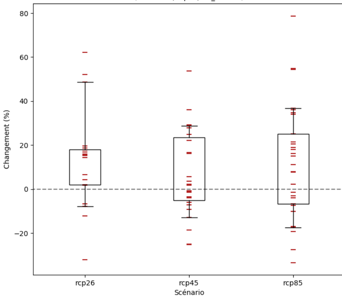
Zone de la côte guinéenne: Changements (%) du maximum de précipitations totales sur une période de 2 jours (novembre; rcp85; BC_0.5x0.5)
