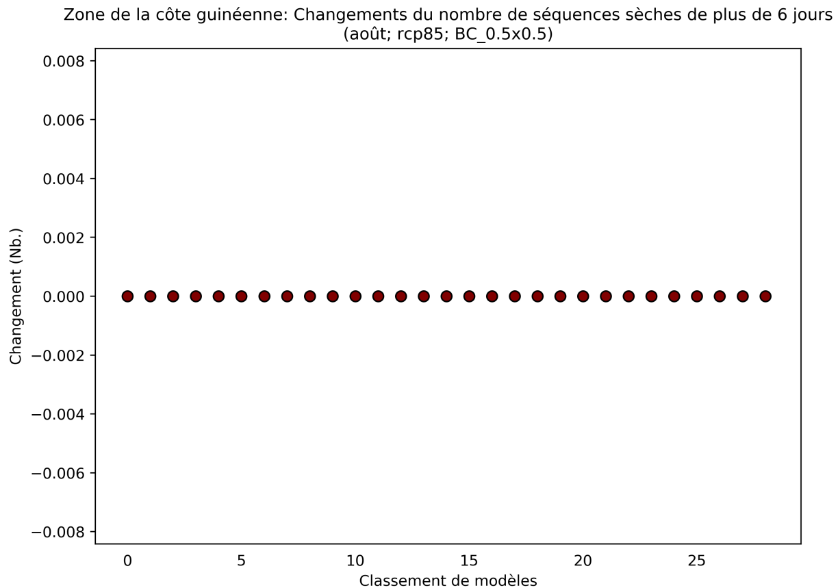
Figure 24: Ce diagramme de dispersion illustre la variation absolue du nombre de séquences sèches de plus de 6 jours entre 2040 et 2059 (par rapport à la période de référence de 1950 à 2000) pour août. Chaque point indique la moyenne spatiale d'un modèle sur Zone de la côte guinéenne; les points sont organisés ("rank", sur l'axe des abscisses) en fonction de la magnitude de leur valeur sur l'axe des ordonnées. Ce diagramme montre la variation absolue pour le scénario RCP8.5.
