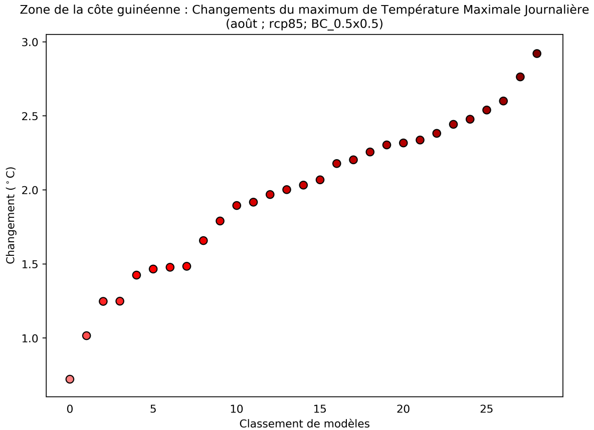
Figure 32: Ce diagramme de dispersion illustre la variation absolue du maximum de température maximale journalière entre 2040 et 2059 (par rapport à la période de référence de 1950 à 2000) pour août. Chaque point indique la moyenne spatiale d'un modèle sur Zone de la côte guinéenne; les points sont organisés ("rank", sur l'axe des abscisses) en fonction de la magnitude de leur valeur sur l'axe des ordonnées. Ce diagramme montre la variation absolue pour le scénario RCP8.5.
