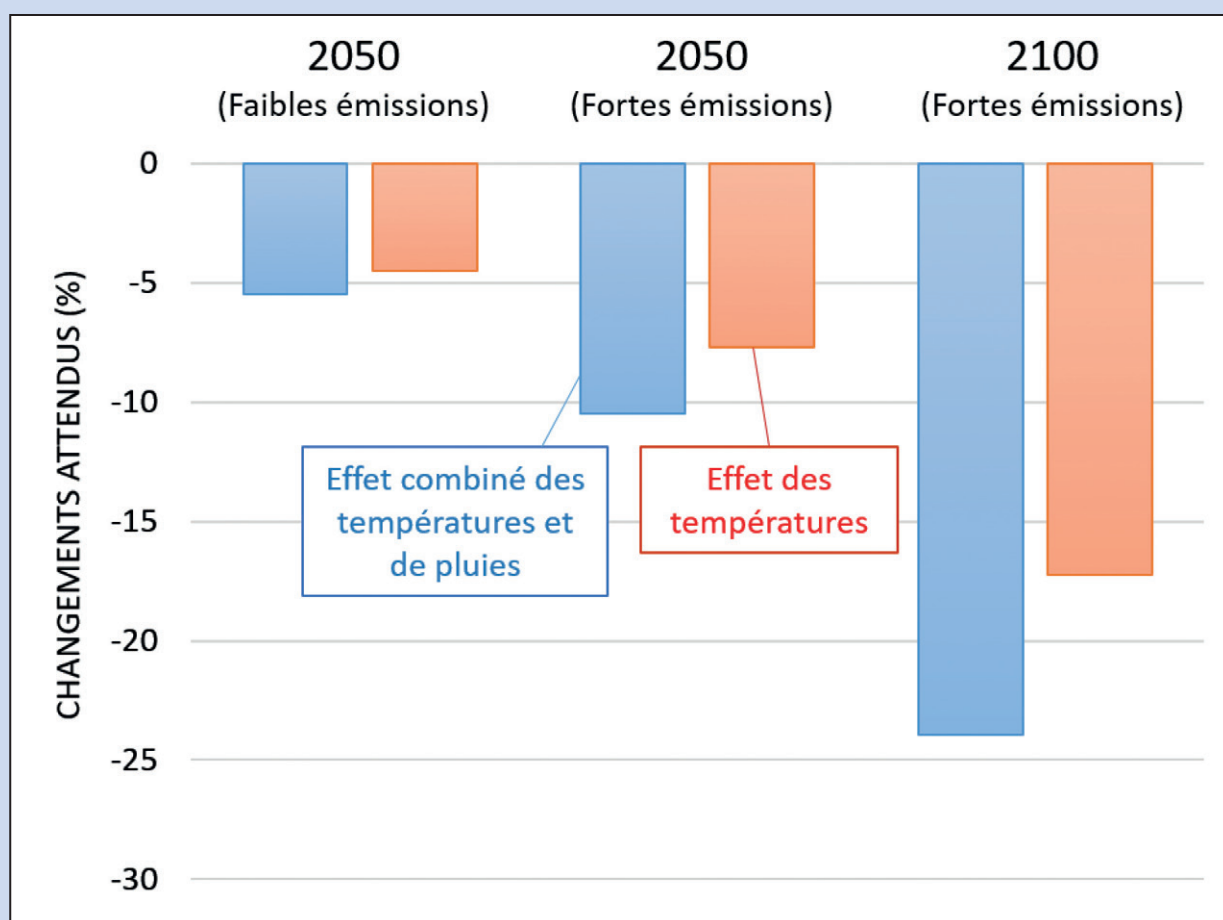
Figure 10: Changements attendus du rendement agricole du mil dans la région de Bamby au Sénégal simulés avec le modèle agronomique CELCIUS et les anomalies de 30 modèles CMIP5. Les valeurs en bleu prennent en compte les effets combinés des changements de températures et de pluies tandis que les valeurs en rouge prennent en compte uniquement les changements de température.
