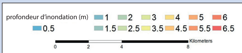
Figure 8: Cartes illustrant comment les changements des pluies intenses et de la couverture végétale de 2016 (en haut) à 2050 (en bas) affecteront la profondeur des inondations dans la ville de Ouagadougou pour un orage particulièrement extrême (attendu une seule fois en 100 ans). Une plus grande partie de la ville sera inondée et les zones déjà sujettes aux inondations connaîtront des niveaux d'inondation plus élevés pendant une plus longue période.
