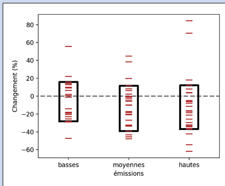
Figure 4: Evolution des précipitations au milieu du 21e siècle, telle que simulée par les modèles climatiques dans des scénarios d'émissions faibles, moyennes et élevées. Chaque ligne rouge indique la projection d'un modèle. Il y a 90% de chances que les changements se situent dans la plage couverte par les rectangles. Les réductions des précipitations se situent en dessous de la ligne pointillée et les augmentations sont au dessus.
