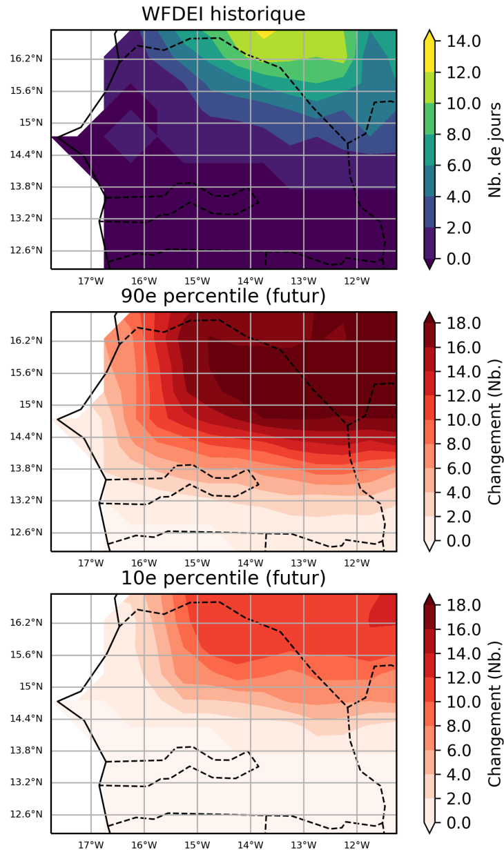
Figure 68: Ces cartes illustrent la projection multi-modèles pour la variation absolue du nombre de jours avec une température maximale > 40^{\circ}\text{C} , pour la période entre 2040 et 2059 (par rapport à la période de référence de 1950 à 2000) pour octobre. Elles indiquent les 90ème et 10ème percentiles de la distribution des modèles dans l'ensemble multi-modèles, calculés séparément en chaque point de grille, sur la région Sénégal. Ce diagramme montre la variation absolue pour le scénario RCP8.5.
