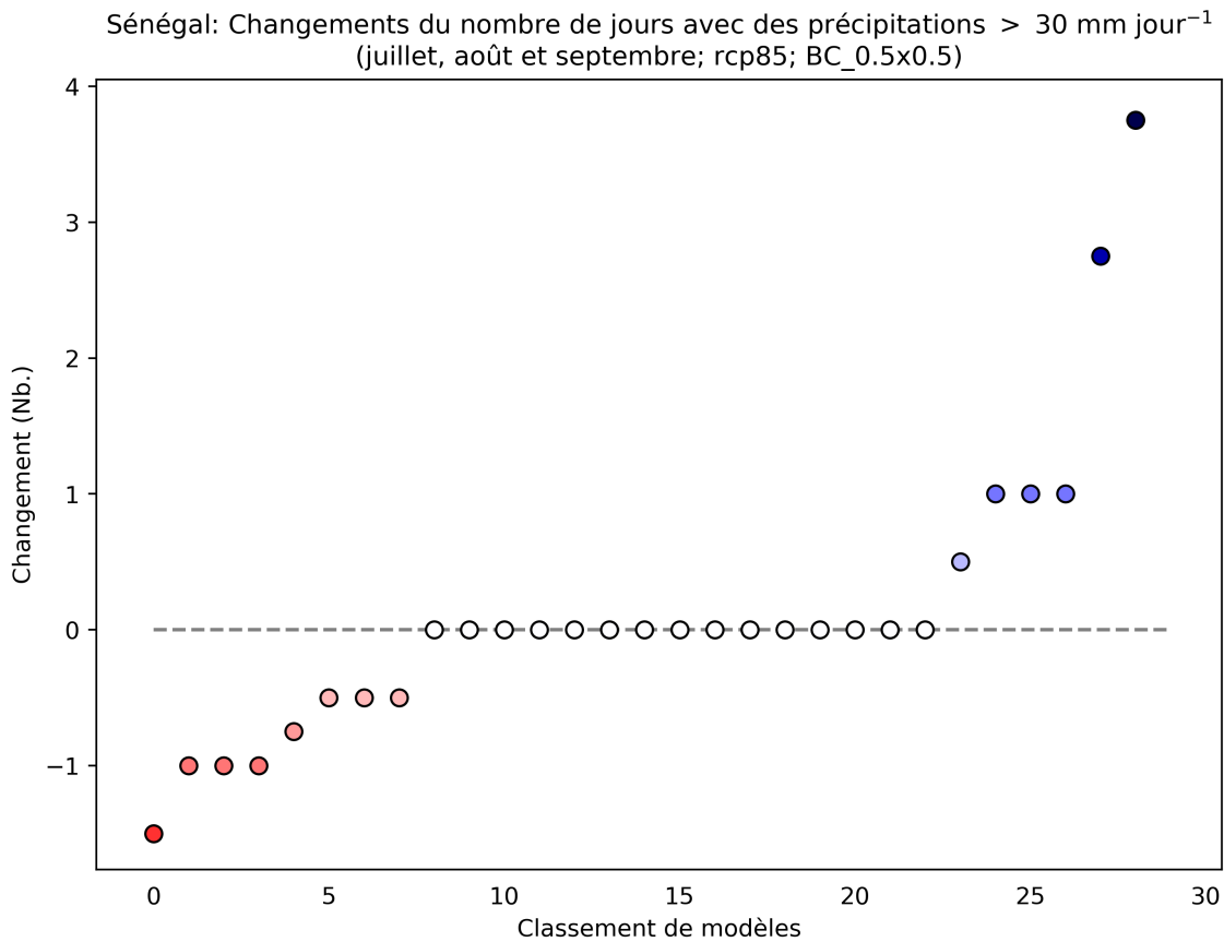
Figure 75: Ce diagramme de dispersion illustre la variation absolue du nombre de jours avec des précipitations > 30 mm jour -1 entre 2040 et 2059 (par rapport à la période de référence de 1950 à 2000) pour juillet, août et septembre. Chaque point indique la moyenne spatiale d'un modèle sur Sénégal; les points sont organisés ("rank", sur l'axe des abscisses) en fonction de la magnitude de leur valeur sur l'axe des ordonnées. Ce diagramme montre la variation absolue pour le scénario RCP8.5.
