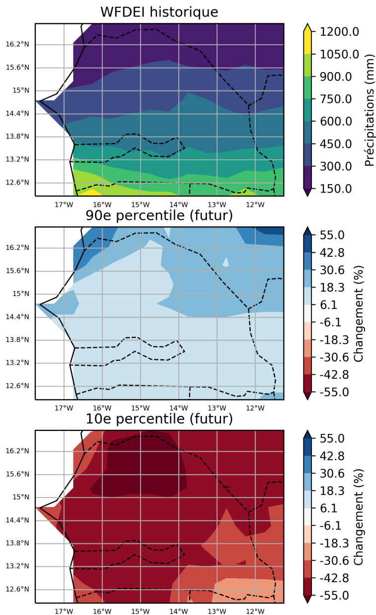
Figure 41: Ces cartes illustrent la projection multi-modèles pour du pourcentage de variation des précipitations totales, pour la période entre 2040 et 2059 (par rapport à la période de référence de 1950 à 2000) pour juillet, août et septembre. Elles indiquent les 90ème et 10ème percentiles de la distribution des modèles dans l'ensemble multi-modèles, calculés séparément en chaque point de grille, sur la région Sénégal. Ce diagramme montre le pourcentage de variation pour le scénario RCP8.5.
