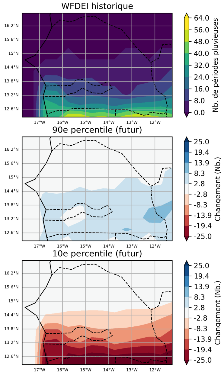
Figure 17: Ces cartes illustrent la projection multi-modèles pour la variation absolue du nombre de séquences pluvieuses de plus de 10 jours, pour la période entre 2040 et 2059 (par rapport à la période de référence de 1950 à 2000) pour juillet, août et septembre. Elles indiquent les 90ème et 10ème percentiles de la distribution des modèles dans l'ensemble multi-modèles, calculés séparément en chaque point de grille, sur la région Sénégal. Ce diagramme montre la variation absolue pour le scénario RCP8.5.
