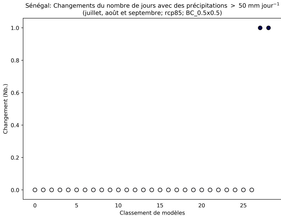
Figure 79: Ce diagramme de dispersion illustre la variation absolue du nombre de jours avec des précipitations > 50 mm jour -1 entre 2040 et 2059 (par rapport à la période de référence de 1950 à 2000) pour juillet, août et septembre. Chaque point indique la moyenne spatiale d'un modèle sur Sénégal; les points sont organisés ("rank", sur l'axe des abscisses) en fonction de la magnitude de leur valeur sur l'axe des ordonnées. Ce diagramme montre la variation absolue pour le scénario RCP8.5.
