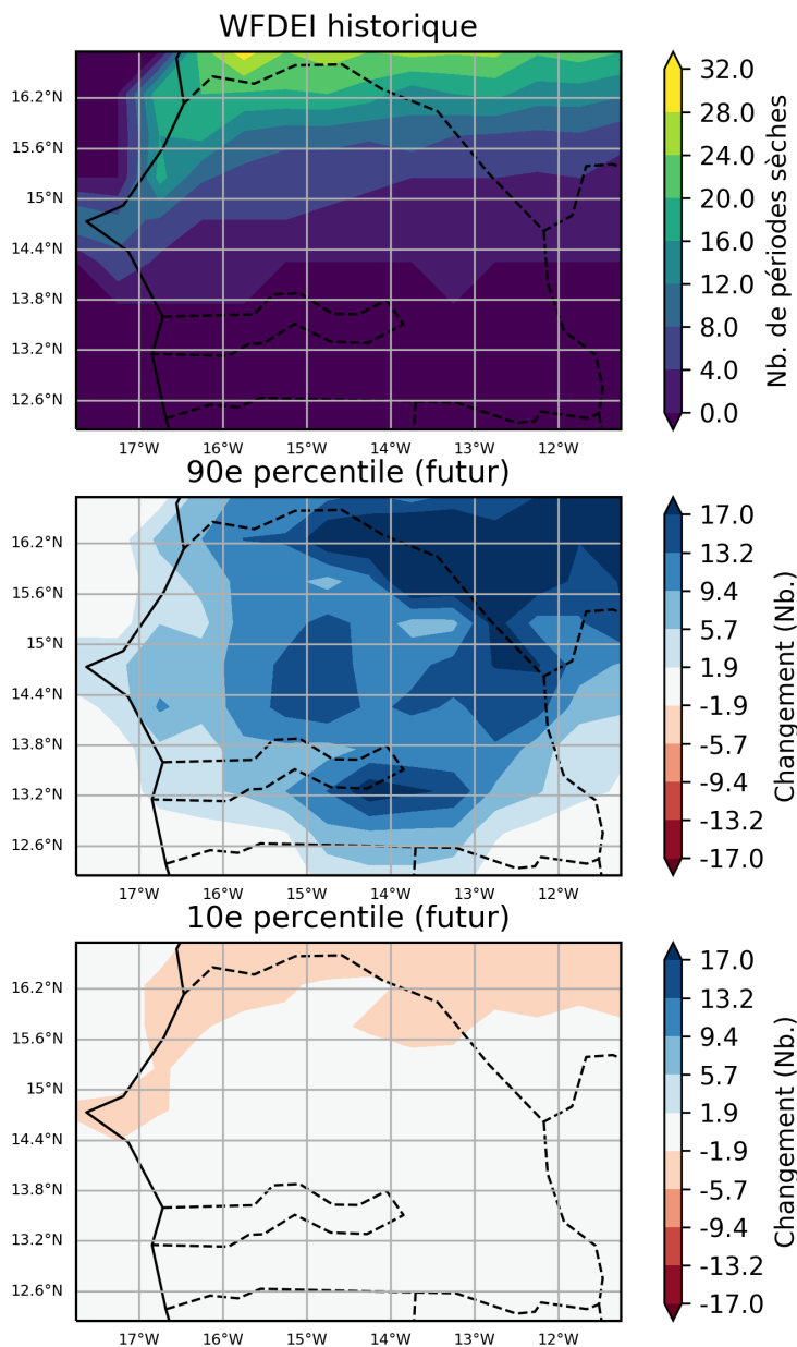
Figure 21: Ces cartes illustrent la projection multi-modèles pour la variation absolue du nombre de séquences sèches de plus de 6 jours, pour la période entre 2040 et 2059 (par rapport à la période de référence de 1950 à 2000) pour juillet, août et septembre. Elles indiquent les 90ème et 10ème percentiles de la distribution des modèles dans l'ensemble multi-modèles, calculés séparément en chaque point de grille, sur la région Sénégal. Ce diagramme montre la variation absolue pour le scénario RCP8.5.
