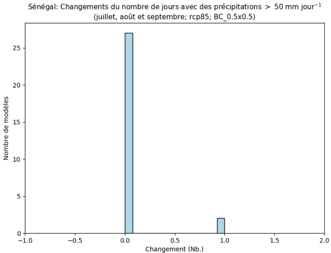
Figure 77: Cet histogramme illustre le nombre de modèles en accord avec la variation absolue du nombre de jours avec des précipitations > 50 mm jour -1 pour la période entre 2040 et 2059 (par rapport à la période de référence de 1950 à 2000) pour juillet, août et septembre. Chaque barre verticale indique le nombre de modèles en accord avec la gamme de valeur indiquée sur l'axe des abscisses pour la région Sénégal. Ce diagramme montre la variation absolue pour le scénario RCP8.5.
