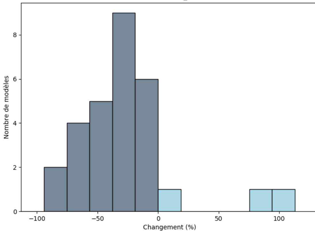
Sénégal: Changements (%) du maximum de précipitations totales sur une période de 2 jours (juillet; rcp85; BC_0.5x0.5)
