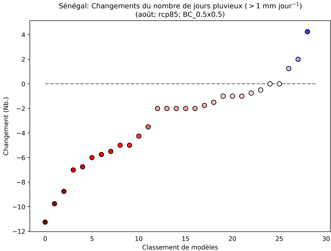
Figure 67: Ce diagramme de dispersion illustre la variation absolue du nombre de jours pluvieux (>1 mm jour -1 ) entre 2040 et 2059 (par rapport à la période de référence de 1950 à 2000) pour août. Chaque point indique la moyenne spatiale d'un modèle sur Sénégal; les points sont organisés ("rank", sur l'axe des abscisses) en fonction de la magnitude de leur valeur sur l'axe des ordonnées. Ce diagramme montre la variation absolue pour le scénario RCP8.5.
