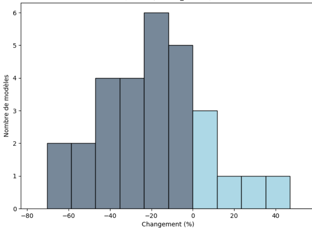
Sénégal: Changements (%) du maximum de précipitations totales sur une période de 5 jours (août; rcp85; BC_0.5x0.5)
