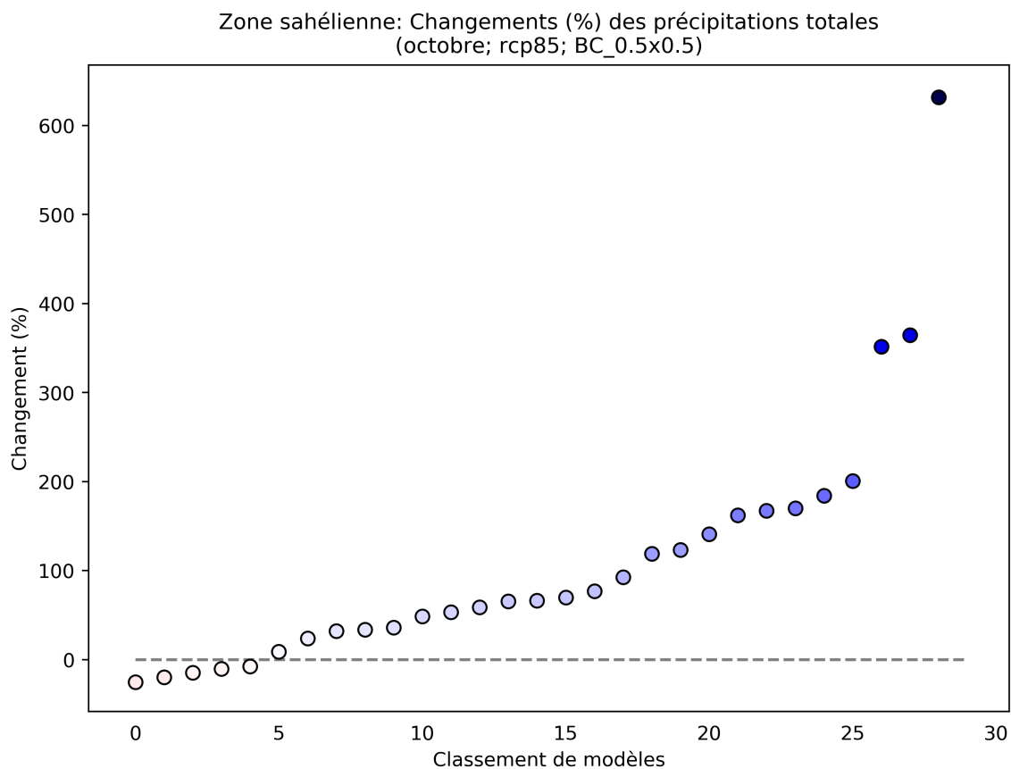
Figure 44: Ce diagramme de dispersion illustre du pourcentage de variation des précipitations totales entre 2040 et 2059 (par rapport à la période de référence de 1950 à 2000) pour octobre. Chaque point indique la moyenne spatiale d'un modèle sur Zone sahélienne; les points sont organisés ("rank", sur l'axe des abscisses) en fonction de la magnitude de leur valeur sur l'axe des ordonnées. Ce diagramme montre le pourcentage de variation pour le scénario RCP8.5.
