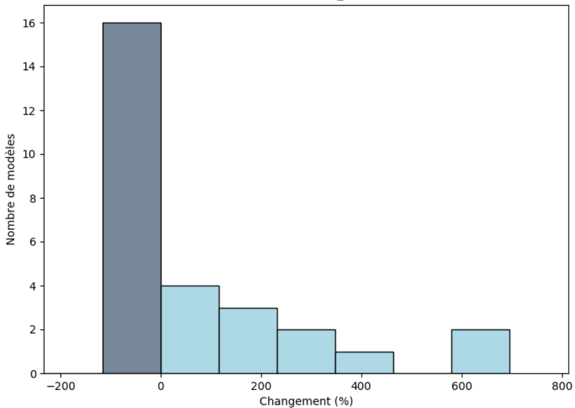
Figure 89: Cet histogramme illustre le nombre de modèles en accord avec du pourcentage de variation du maximum de précipitations totales sur une période de 2 jours pour la période entre 2040 et 2059 (par rapport à la période de référence de 1950 à 2000) pour octobre. Chaque barre verticale indique le nombre de modèles en accord avec la gamme de valeur indiquée sur l'axe des abscisses pour la région Zone sahélienne. Ce diagramme montre le pourcentage de variation pour le scénario RCP8.5.
