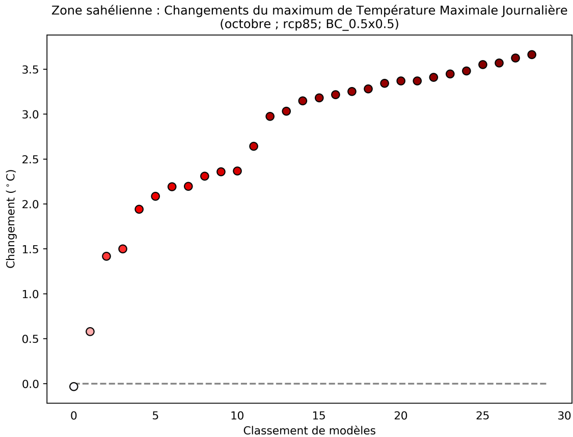
Figure 32: Ce diagramme de dispersion illustre la variation absolue du maximum de température maximale journalière entre 2040 et 2059 (par rapport à la période de référence de 1950 à 2000) pour octobre. Chaque point indique la moyenne spatiale d'un modèle sur Zone sahélienne; les points sont organisés ("rank", sur l'axe des abscisses) en fonction de la magnitude de leur valeur sur l'axe des ordonnées. Ce diagramme montre la variation absolue pour le scénario RCP8.5.
