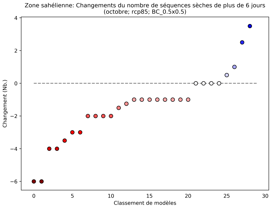
Figure 24: Ce diagramme de dispersion illustre la variation absolue du nombre de séquences sèches de plus de 6 jours entre 2040 et 2059 (par rapport à la période de référence de 1950 à 2000) pour octobre. Chaque point indique la moyenne spatiale d'un modèle sur Zone sahélienne; les points sont organisés ("rank", sur l'axe des abscisses) en fonction de la magnitude de leur valeur sur l'axe des ordonnées. Ce diagramme montre la variation absolue pour le scénario RCP8.5.
