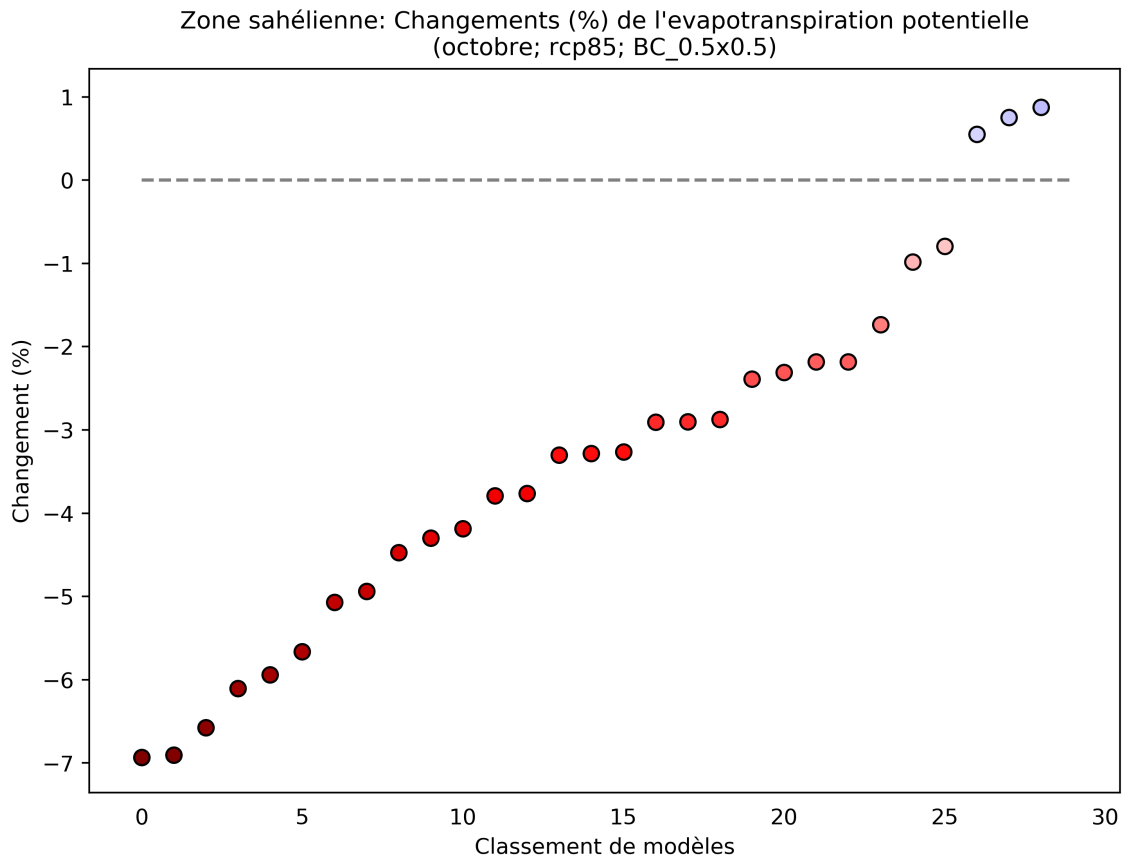
Figure 4: Ce diagramme de dispersion illustre du pourcentage de variation de l'évapotranspiration potentielle entre 2040 et 2059 (par rapport à la période de référence de 1950 à 2000) pour octobre. Chaque point indique la moyenne spatiale d'un modèle sur Zone sahélienne; les points sont organisés ("rank", sur l'axe des abscisses) en fonction de la magnitude de leur valeur sur l'axe des ordonnées. Ce diagramme montre le pourcentage de variation pour le scénario RCP8.5.
