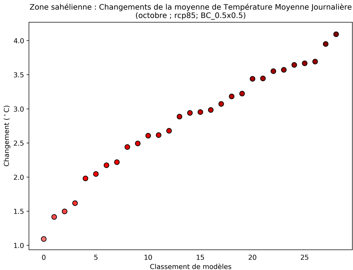
Figure 48: Ce diagramme de dispersion illustre la variation absolue de la moyenne de température moyenne journalière entre 2040 et 2059 (par rapport à la période de référence de 1950 à 2000) pour octobre. Chaque point indique la moyenne spatiale d'un modèle sur Zone sahélienne; les points sont organisés ("rank", sur l'axe des abscisses) en fonction de la magnitude de leur valeur sur l'axe des ordonnées. Ce diagramme montre la variation absolue pour le scénario RCP8.5.
