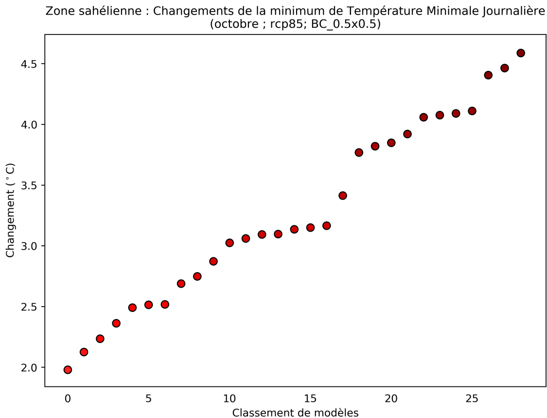
Figure 40: Ce diagramme de dispersion illustre la variation absolue de la minimum de température minimale journalière entre 2040 et 2059 (par rapport à la période de référence de 1950 à 2000) pour octobre. Chaque point indique la moyenne spatiale d'un modèle sur Zone sahélienne; les points sont organisés ("rank", sur l'axe des abscisses) en fonction de la magnitude de leur valeur sur l'axe des ordonnées. Ce diagramme montre la variation absolue pour le scénario RCP8.5.
