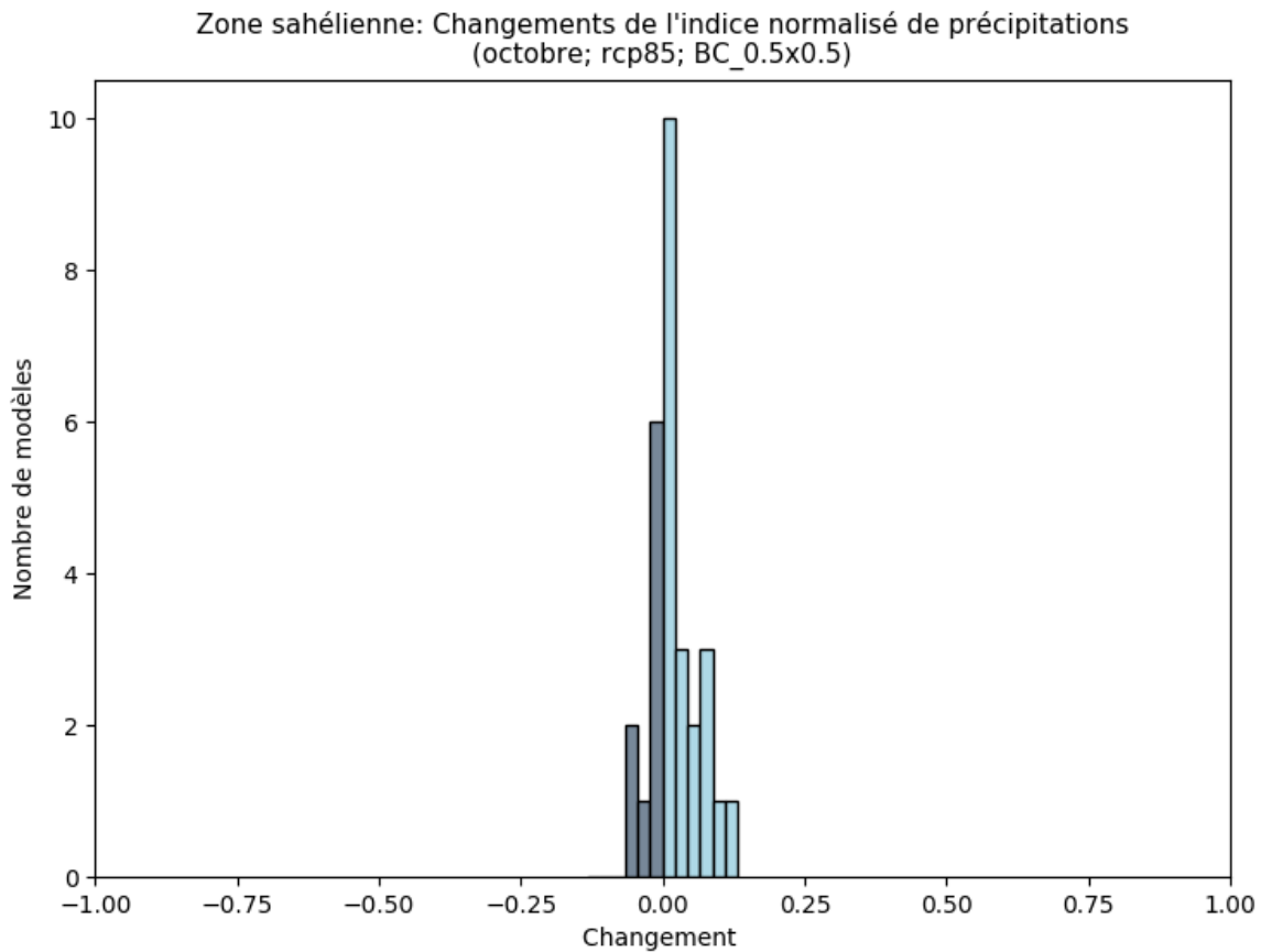
Figure 10: Cet histogramme illustre le nombre de modèles en accord avec la variation absolue de l'indice normalisé de précipitations pour la période entre 2040 et 2059 (par rapport à la période de référence de 1950 à 2000) pour octobre. Chaque barre verticale indique le nombre de modèles en accord avec la gamme de valeur indiquée sur l'axe des abscisses pour la région Zone sahéenne. Ce diagramme montre la variation absolue pour le scénario RCP8.5.
