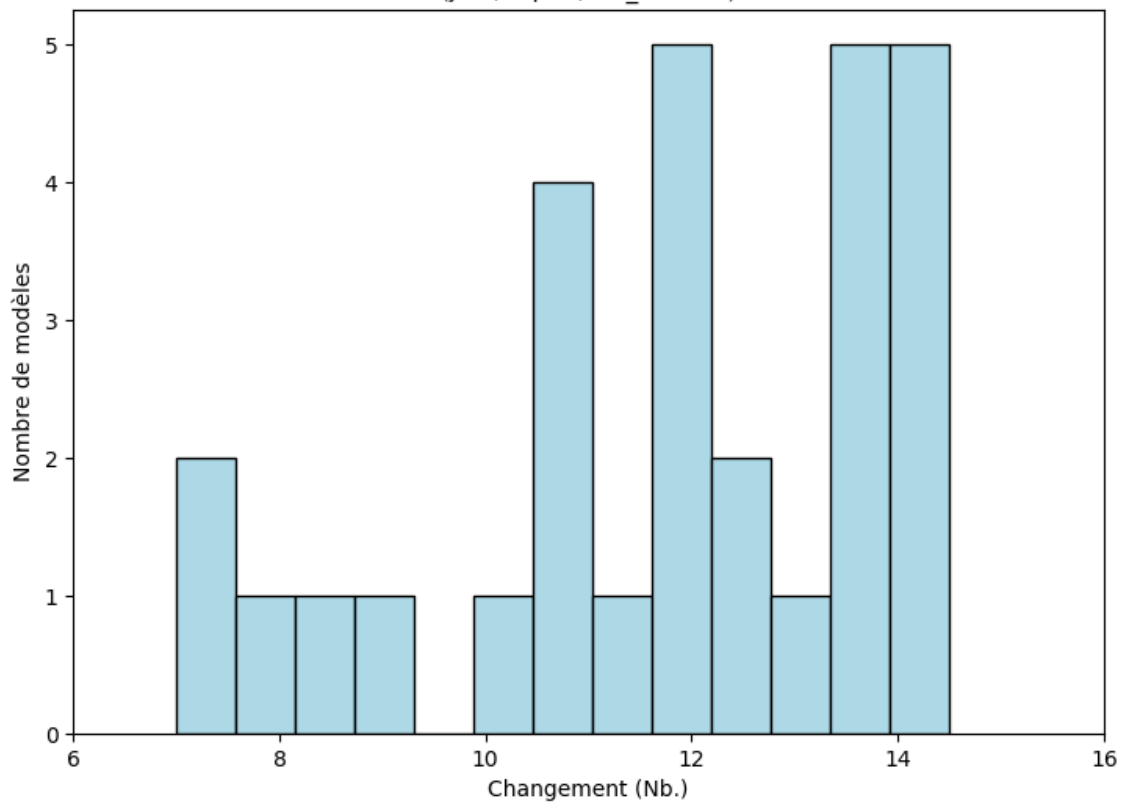
Zone sahélienne: Changements du nombre de jours avec une température maximale > 40 ° c (juin; rcp85; BC_0.5x0.5)
