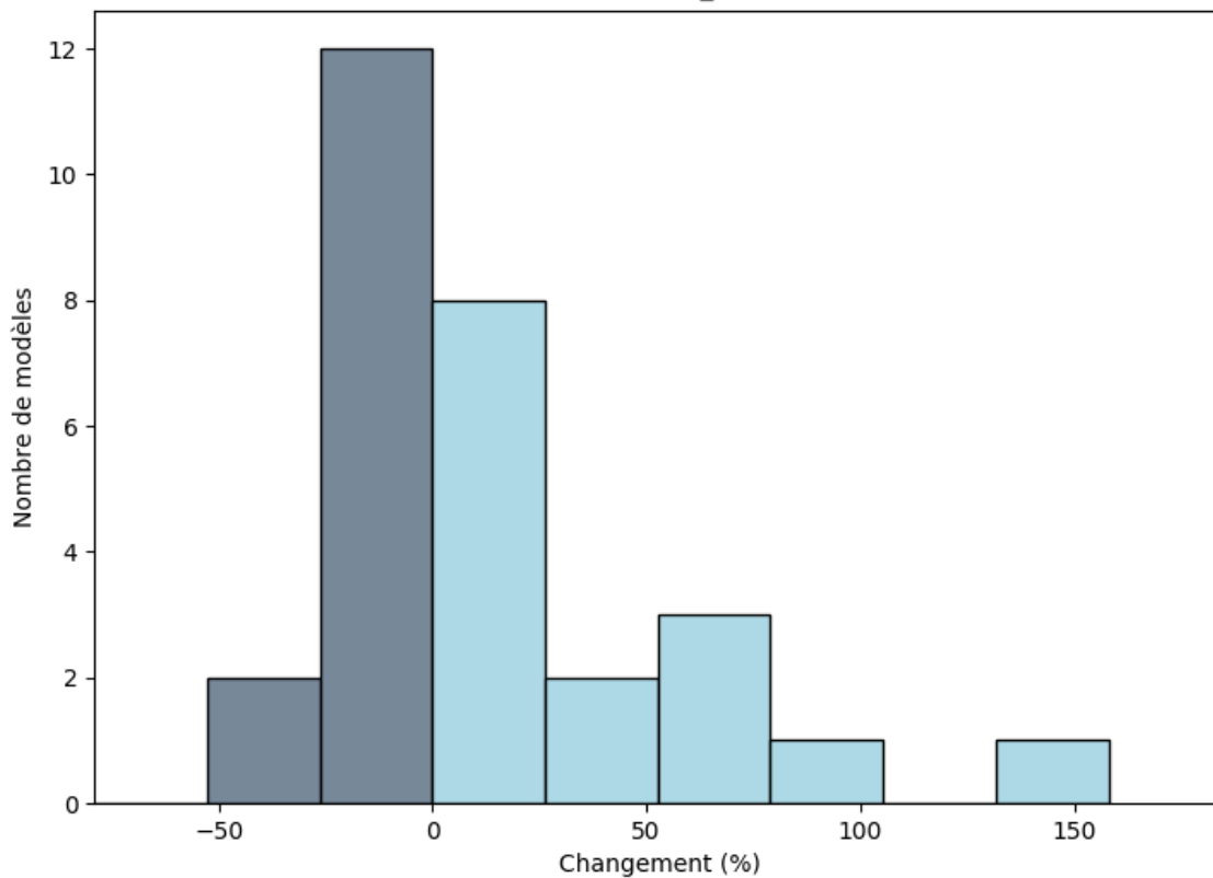
Zone sahélienne: Changements (%) du maximum de précipitations totales sur une période de 5 jours (juin; rcp85; BC_0.5x0.5)
