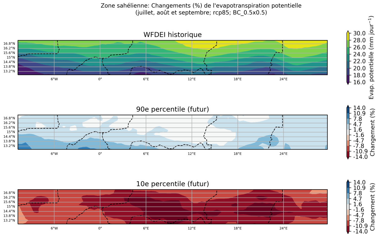
Figure 1: Ces cartes illustrent la projection multi-modèles pour du pourcentage de variation de l'évapotranspiration potentielle, pour la période entre 2040 et 2059 (par rapport à la période de référence de 1950 à 2000) pour juillet, août et septembre. Elles indiquent les 90ème et 10ème percentiles de la distribution des modèles dans l'ensemble multi-modèles, calculés séparément en chaque point de grille, sur la région Zone sahélienne. Ce diagramme montre le pourcentage de variation pour le scénario RCP8.5.
