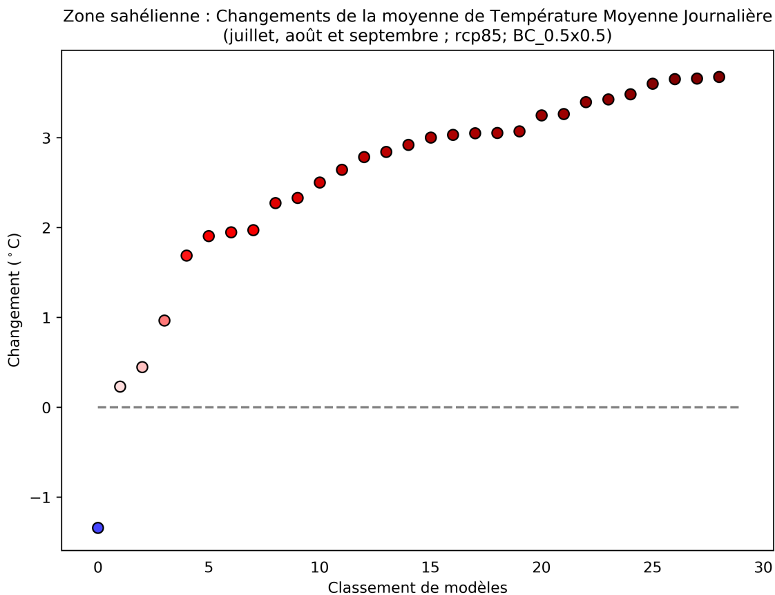
Figure 48: Ce diagramme de dispersion illustre la variation absolue de la moyenne de température moyenne journalière entre 2040 et 2059 (par rapport à la période de référence de 1950 à 2000) pour juillet, août et septembre. Chaque point indique la moyenne spatiale d'un modèle sur Zone sahélienne; les points sont organisés ("rank", sur l'axe des abscisses) en fonction de la magnitude de leur valeur sur l'axe des ordonnées. Ce diagramme montre la variation absolue pour le scénario RCP8.5.
