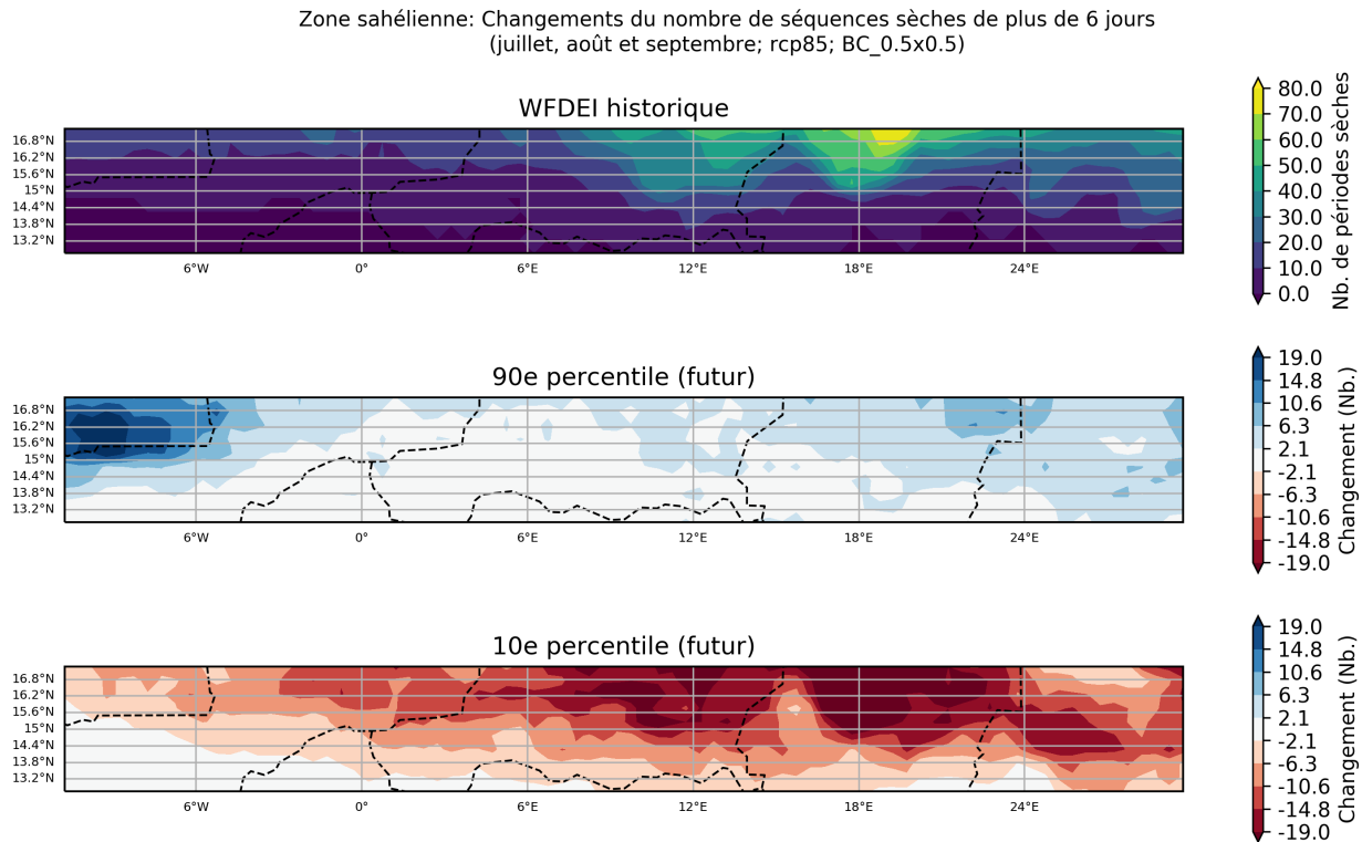
Figure 21: Ces cartes illustrent la projection multi-modèles pour la variation absolue du nombre de séquences sèches de plus de 6 jours, pour la période entre 2040 et 2059 (par rapport à la période de référence de 1950 à 2000) pour juillet, août et septembre. Elles indiquent les 90ème et 10ème percentiles de la distribution des modèles dans l'ensemble multi-modèles, calculés séparément en chaque point de grille, sur la région Zone sahélienne. Ce diagramme montre la variation absolue pour le scénario RCP8.5.
