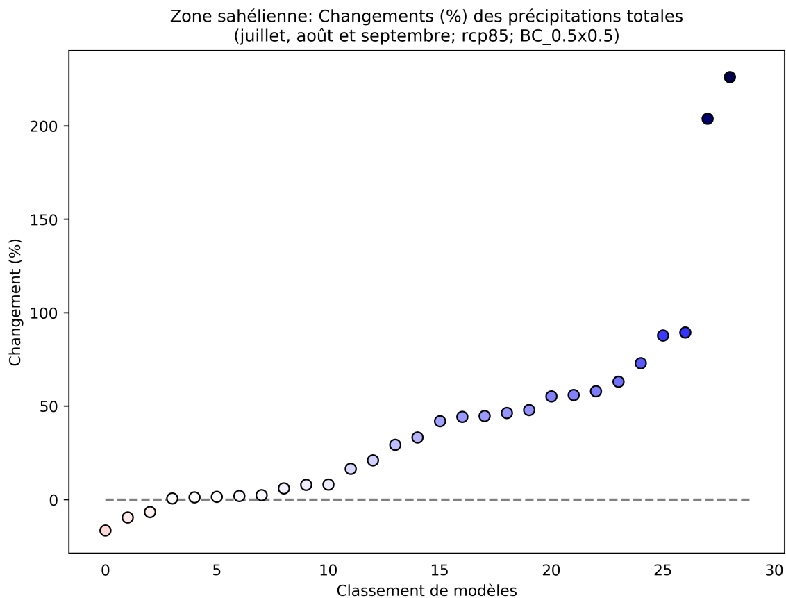
Figure 44: Ce diagramme de dispersion illustre du pourcentage de variation des précipitations totales entre 2040 et 2059 (par rapport à la période de référence de 1950 à 2000) pour juillet, août et septembre. Chaque point indique la moyenne spatiale d'un modèle sur Zone sahélienne; les points sont organisés ("rank", sur l'axe des abscisses) en fonction de la magnitude de leur valeur sur l'axe des ordonnées. Ce diagramme montre le pourcentage de variation pour le scénario RCP8.5.
