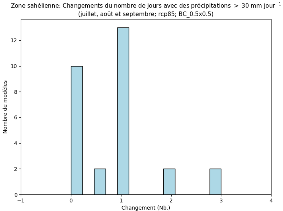
Figure 73: Cet histogramme illustre le nombre de modèles en accord avec la variation absolue du nombre de jours avec des précipitations > 30 \text{ mm jour}^{-1} pour la période entre 2040 et 2059 (par rapport à la période de référence de 1950 à 2000) pour juillet, août et septembre. Chaque barre verticale indique le nombre de modèles en accord avec la gamme de valeur indiquée sur l'axe des abscisses pour la région Zone sahélienne. Ce diagramme montre la variation absolue pour le scénario RCP8.5.
