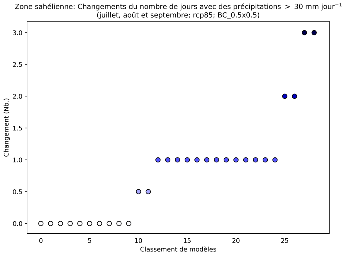
Figure 75: Ce diagramme de dispersion illustre la variation absolue du nombre de jours avec des précipitations > 30 \text{ mm jour}^{-1} entre 2040 et 2059 (par rapport à la période de référence de 1950 à 2000) pour juillet, août et septembre. Chaque point indique la moyenne spatiale d'un modèle sur Zone sahélienne; les points sont organisés ("rank", sur l'axe des abscisses) en fonction de la magnitude de leur valeur sur l'axe des ordonnées. Ce diagramme montre la variation absolue pour le scénario RCP8.5.
