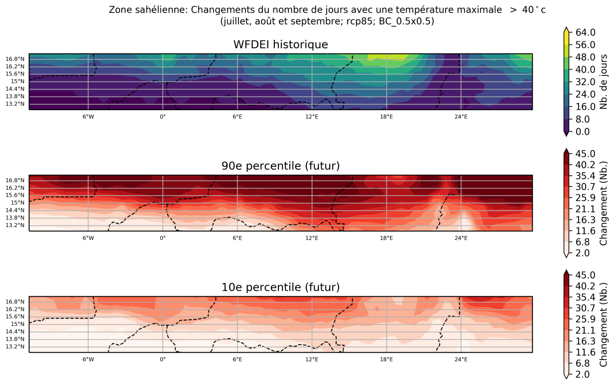
Figure 68: Ces cartes illustrent la projection multi-modèles pour la variation absolue du nombre de jours avec une température maximale > 40°C, pour la période entre 2040 et 2059 (par rapport à la période de référence de 1950 à 2000) pour juillet, août et septembre. Elles indiquent les 90ème et 10ème percentiles de la distribution des modèles dans l'ensemble multi-modèles, calculés séparément en chaque point de grille, sur la région Zone sahélienne. Ce diagramme montre la variation absolue pour le scénario RCP8.5.
