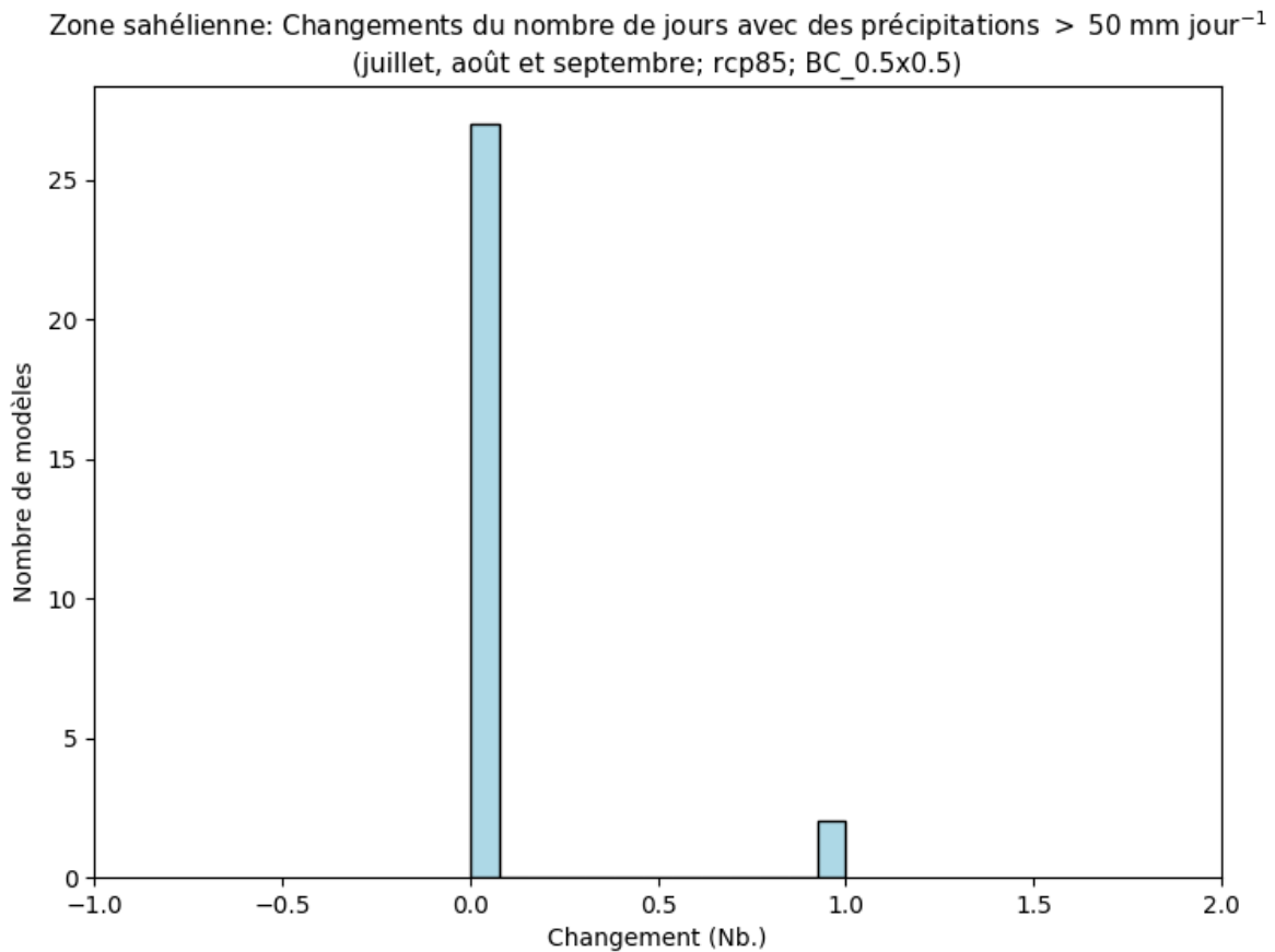
Figure 77: Cet histogramme illustre le nombre de modèles en accord avec la variation absolue du nombre de jours avec des précipitations > 50 \text{ mm jour}^{-1} pour la période entre 2040 et 2059 (par rapport à la période de référence de 1950 à 2000) pour juillet, août et septembre. Chaque barre verticale indique le nombre de modèles en accord avec la gamme de valeur indiquée sur l'axe des abscisses pour la région Zone sahélienne. Ce diagramme montre la variation absolue pour le scénario RCP8.5.
