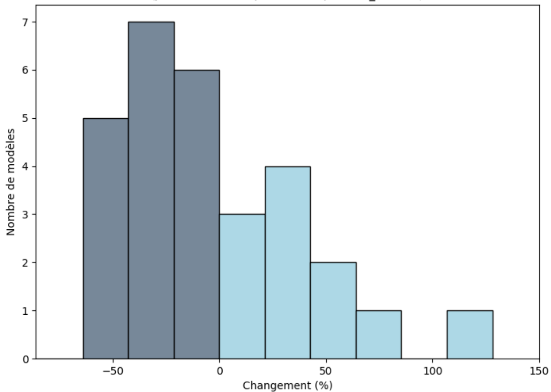
Figure 81: Cet histogramme illustre le nombre de modèles en accord avec du pourcentage de variation du maximum de précipitations totales sur une période de 5 jours pour la période entre 2040 et 2059 (par rapport à la période de référence de 1950 à 2000) pour juillet, août et septembre. Chaque barre verticale indique le nombre de modèles en accord avec la gamme de valeur indiquée sur l'axe des abscisses pour la région Zone sahélienne. Ce diagramme montre le pourcentage de variation pour le scénario RCP8.5.
