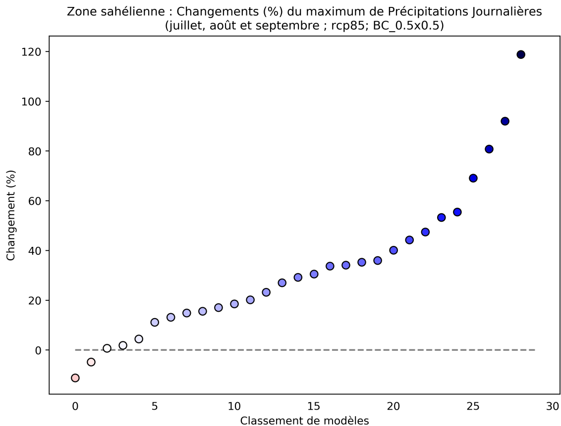
Figure 28: Ce diagramme de dispersion illustre du pourcentage de variation du maximum de précipitations journalières entre 2040 et 2059 (par rapport à la période de référence de 1950 à 2000) pour juillet, août et septembre. Chaque point indique la moyenne spatiale d'un modèle sur Zone sahélienne; les points sont organisés ("rank", sur l'axe des abscisses) en fonction de la magnitude de leur valeur sur l'axe des ordonnées. Ce diagramme montre le pourcentage de variation pour le scénario RCP8.5.
