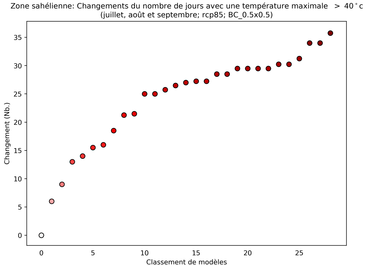
Figure 71: Ce diagramme de dispersion illustre la variation absolue du nombre de jours avec une température maximale > 40°C entre 2040 et 2059 (par rapport à la période de référence de 1950 à 2000) pour juillet, août et septembre. Chaque point indique la moyenne spatiale d'un modèle sur Zone sahélienne; les points sont organisés ("rank", sur l'axe des abscisses) en fonction de la magnitude de leur valeur sur l'axe des ordonnées. Ce diagramme montre la variation absolue pour le scénario RCP8.5.
