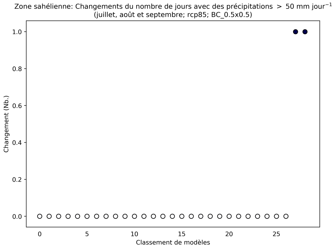
Figure 79: Ce diagramme de dispersion illustre la variation absolue du nombre de jours avec des précipitations > 50 \text{ mm jour}^{-1} entre 2040 et 2059 (par rapport à la période de référence de 1950 à 2000) pour juillet, août et septembre. Chaque point indique la moyenne spatiale d'un modèle sur Zone sahélienne; les points sont organisés ("rank", sur l'axe des abscisses) en fonction de la magnitude de leur valeur sur l'axe des ordonnées. Ce diagramme montre la variation absolue pour le scénario RCP8.5.
