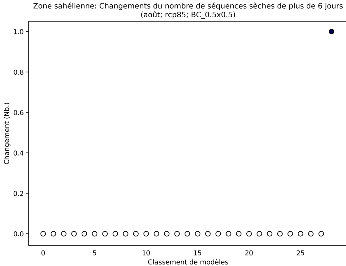
Figure 24: Ce diagramme de dispersion illustre la variation absolue du nombre de séquences sèches de plus de 6 jours entre 2040 et 2059 (par rapport à la période de référence de 1950 à 2000) pour août. Chaque point indique la moyenne spatiale d'un modèle sur Zone sahélienne; les points sont organisés ("rank", sur l'axe des abscisses) en fonction de la magnitude de leur valeur sur l'axe des ordonnées. Ce diagramme montre la variation absolue pour le scénario RCP8.5.
