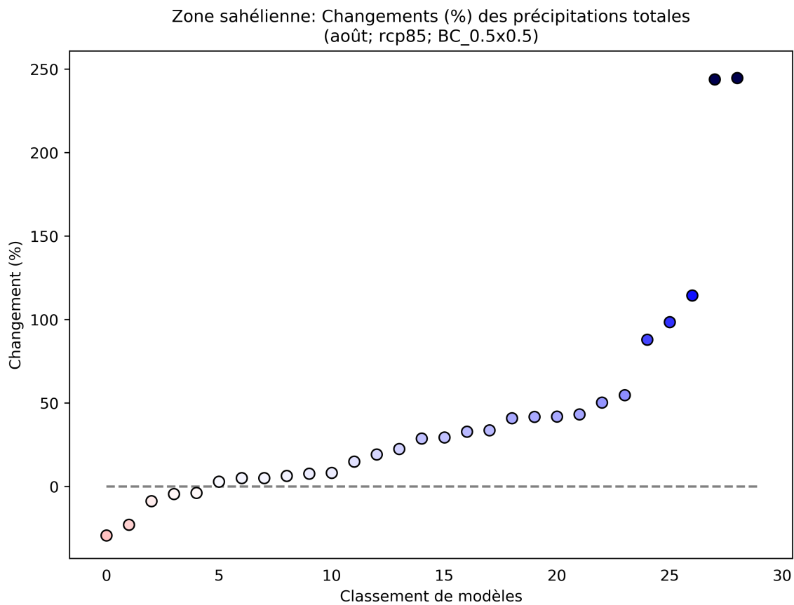
Figure 44: Ce diagramme de dispersion illustre du pourcentage de variation des précipitations totales entre 2040 et 2059 (par rapport à la période de référence de 1950 à 2000) pour août. Chaque point indique la moyenne spatiale d'un modèle sur Zone sahélienne; les points sont organisés ("rank", sur l'axe des abscisses) en fonction de la magnitude de leur valeur sur l'axe des ordonnées. Ce diagramme montre le pourcentage de variation pour le scénario RCP8.5.
