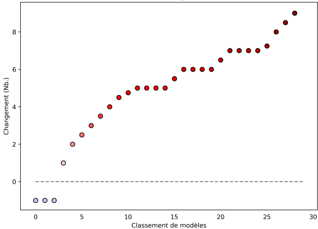
Figure 71: Ce diagramme de dispersion illustre la variation absolue du nombre de jours avec une température maximale > 40^{\circ}\text{C} entre 2040 et 2059 (par rapport à la période de référence de 1950 à 2000) pour août. Chaque point indique la moyenne spatiale d'un modèle sur Zone sahélienne; les points sont organisés ("rank", sur l'axe des abscisses) en fonction de la magnitude de leur valeur sur l'axe des ordonnées. Ce diagramme montre la variation absolue pour le scénario RCP8.5.
