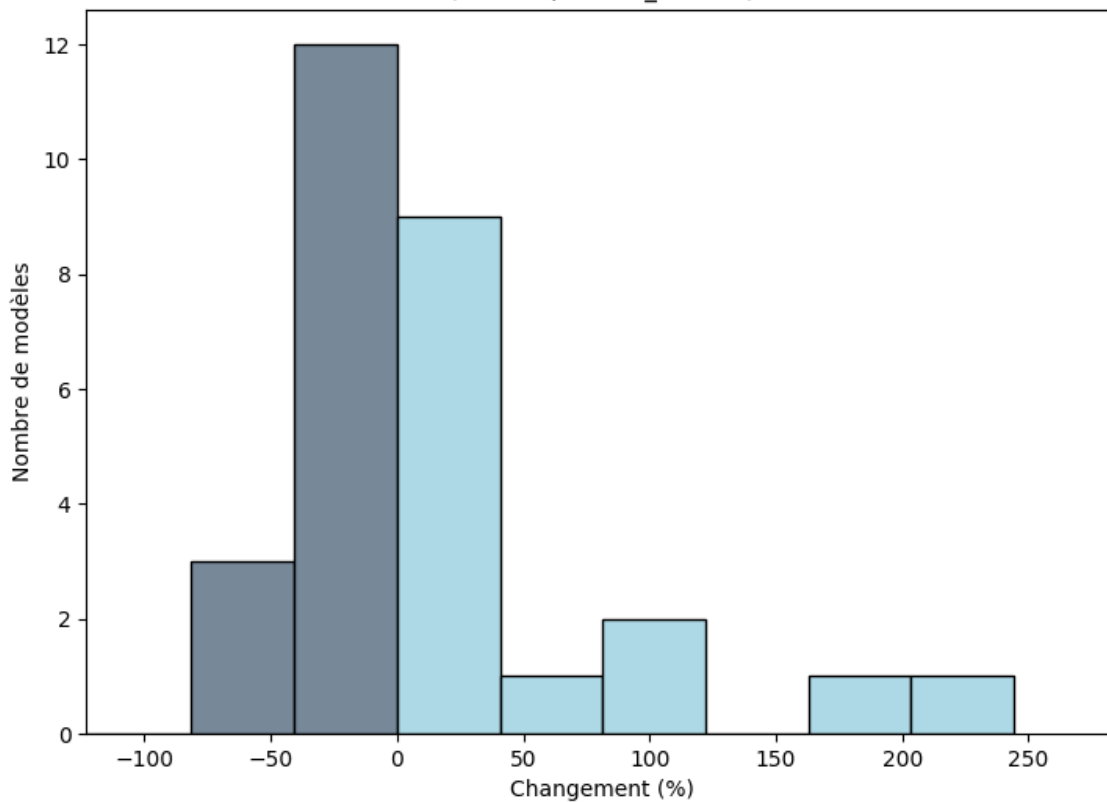
Zone sahélienne: Changements (%) du maximum de précipitations totales sur une période de 2 jours (août; rcp85; BC_0.5x0.5)
