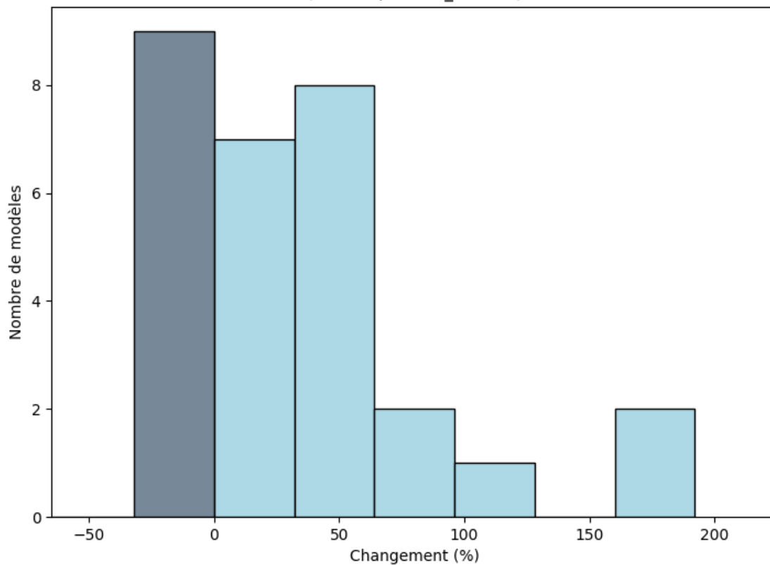
Zone sahélienne: Changements (%) du maximum de précipitations totales sur une période de 5 jours (août; rcp85; BC_0.5x0.5)
