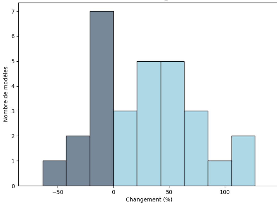
Burkina Faso: Changements (%) du maximum de précipitations totales sur une période de 2 jours (octobre; rcp85; BC_0.5x0.5)
