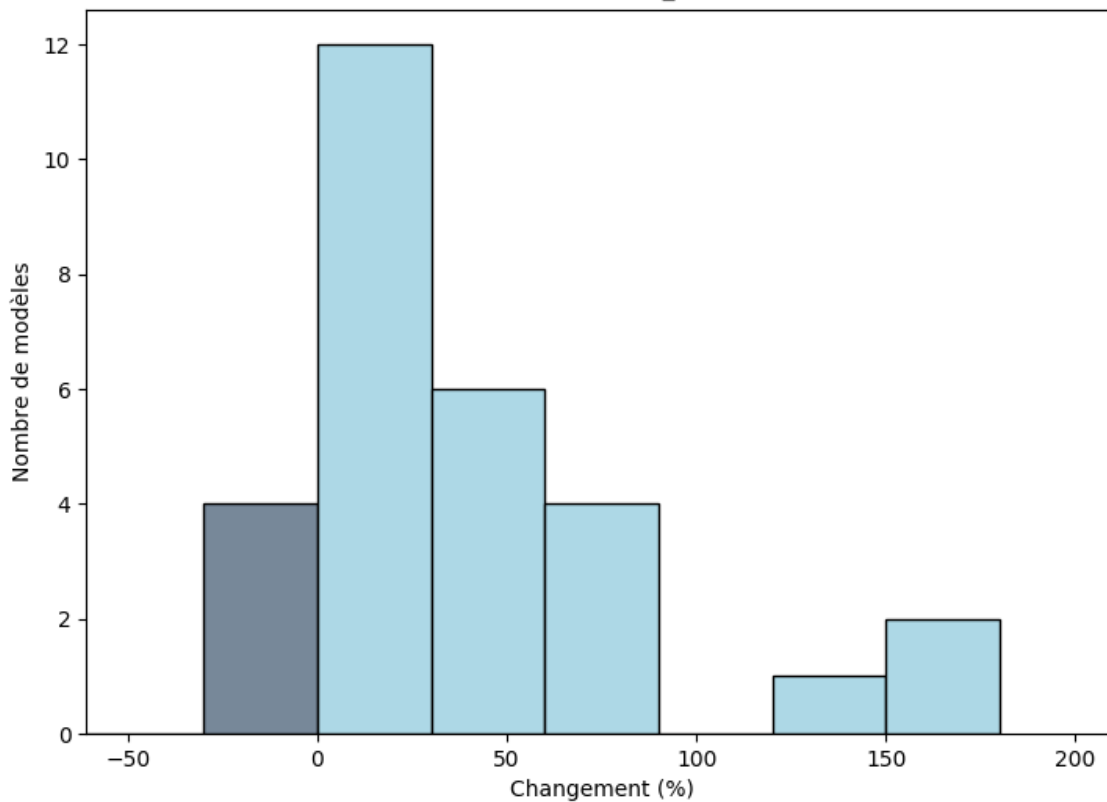
Burkina Faso: Changements (%) du maximum de précipitations totales sur une période de 5 jours (octobre; rcp85; BC_0.5x0.5)
