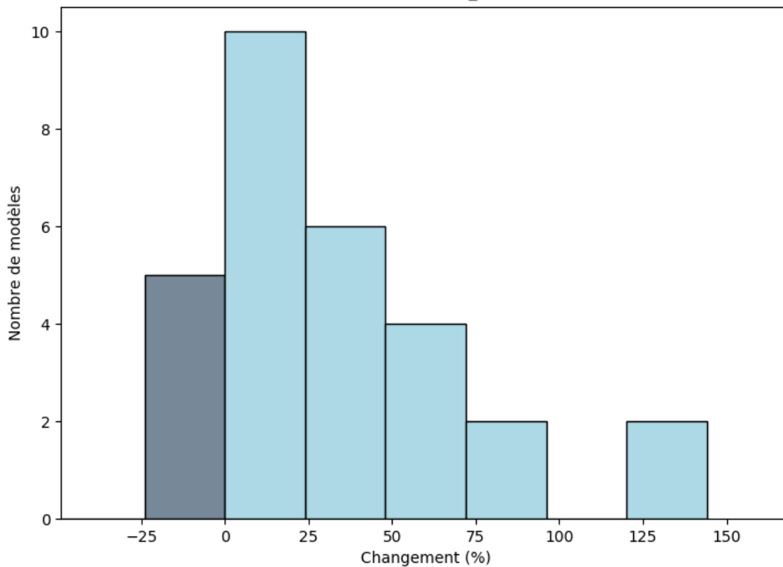
Burkina Faso: Changements (%) du maximum de précipitations totales sur une période de 3 jours (octobre; rcp85; BC_0.5x0.5)
