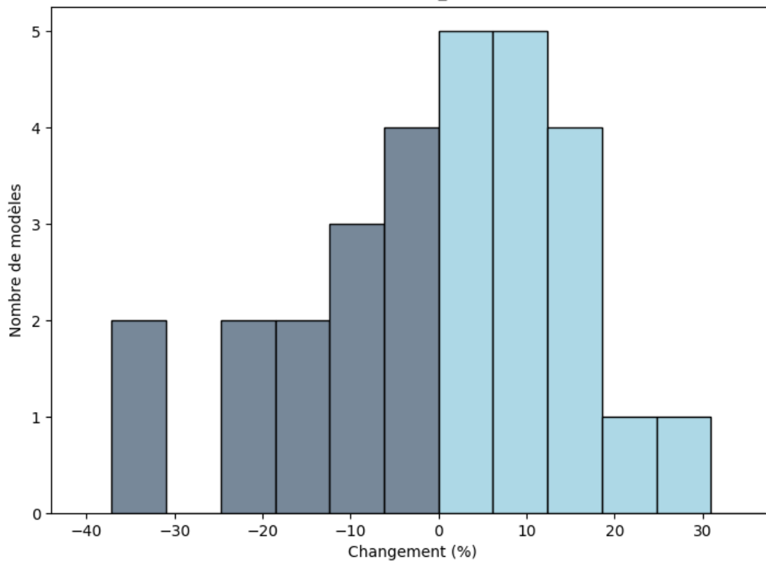
Burkina Faso: Changements (%) du maximum de précipitations totales sur une période de 5 jours (juin; rcp85; BC_0.5x0.5)
