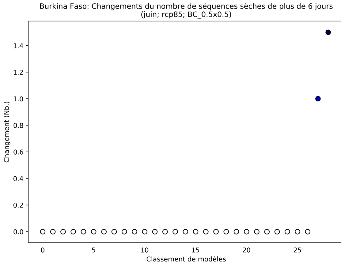
Figure 24: Ce diagramme de dispersion illustre la variation absolue du nombre de séquences sèches de plus de 6 jours entre 2040 et 2059 (par rapport à la période de référence de 1950 à 2000) pour juin. Chaque point indique la moyenne spatiale d'un modèle sur Burkina Faso; les points sont organisés ("rank", sur l'axe des abscisses) en fonction de la magnitude de leur valeur sur l'axe des ordonnées. Ce diagramme montre la variation absolue pour le scénario RCP8.5.
