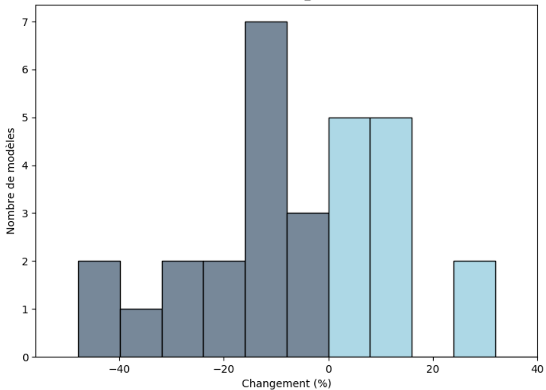
Burkina Faso: Changements (%) du maximum de précipitations totales sur une période de 2 jours (juin; rcp85; BC_0.5x0.5)
