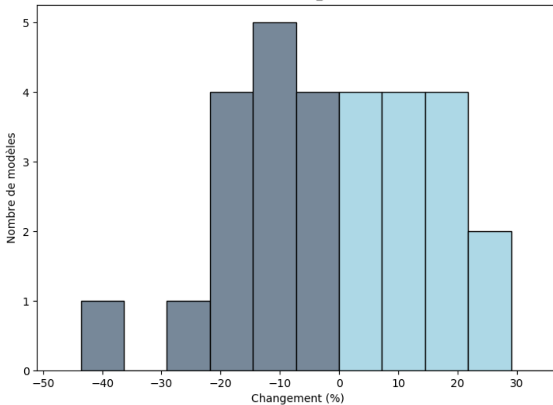
Burkina Faso: Changements (%) du maximum de précipitations totales sur une période de 3 jours (juin; rcp85; BC_0.5x0.5)
