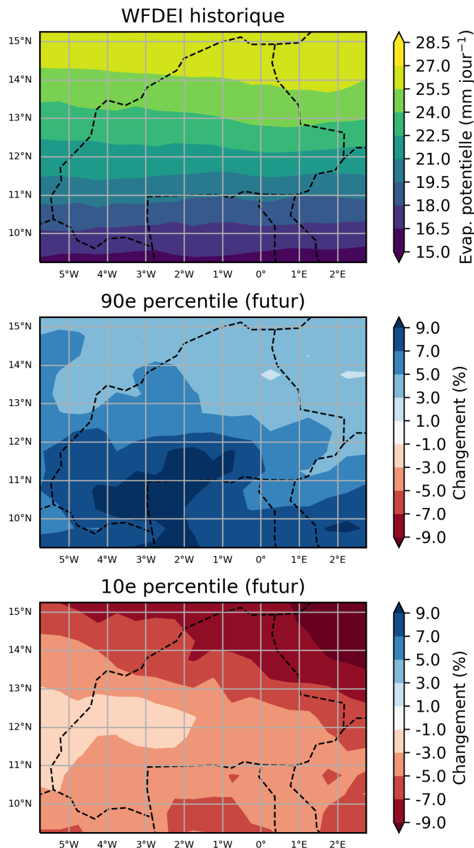
Figure 1: Ces cartes illustrent la projection multi-modèles pour du pourcentage de variation de l'évapotranspiration potentielle, pour la période entre 2040 et 2059 (par rapport à la période de référence de 1950 à 2000) pour juin. Elles indiquent les 90ème et 10ème percentiles de la distribution des modèles dans l'ensemble multi-modèles, calculés séparément en chaque point de grille, sur la région Burkina Faso. Ce diagramme montre le pourcentage de variation pour le scénario RCP8.5.
