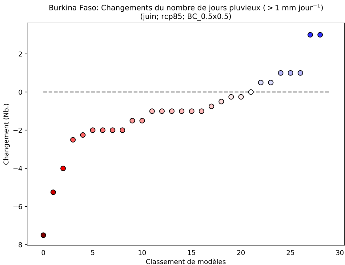
Figure 67: Ce diagramme de dispersion illustre la variation absolue du nombre de jours pluvieux (>1 mm jour -1 ) entre 2040 et 2059 (par rapport à la période de référence de 1950 à 2000) pour juin. Chaque point indique la moyenne spatiale d'un modèle sur Burkina Faso; les points sont organisés ("rank", sur l'axe des abscisses) en fonction de la magnitude de leur valeur sur l'axe des ordonnées. Ce diagramme montre la variation absolue pour le scénario RCP8.5.
