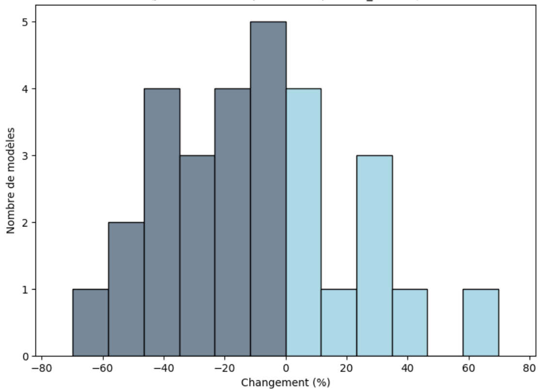
Burkina Faso: Changements (%) du maximum de précipitations totales sur une période de 3 jours (juillet, août et septembre; rcp85; BC_0.5x0.5)
