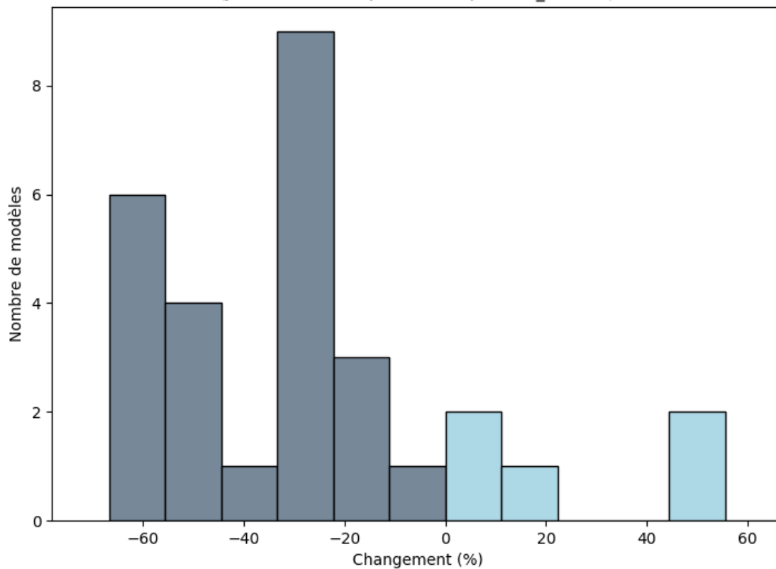
Burkina Faso: Changements (%) du maximum de précipitations totales sur une période de 2 jours (juillet, août et septembre; rcp85; BC_0.5x0.5)
