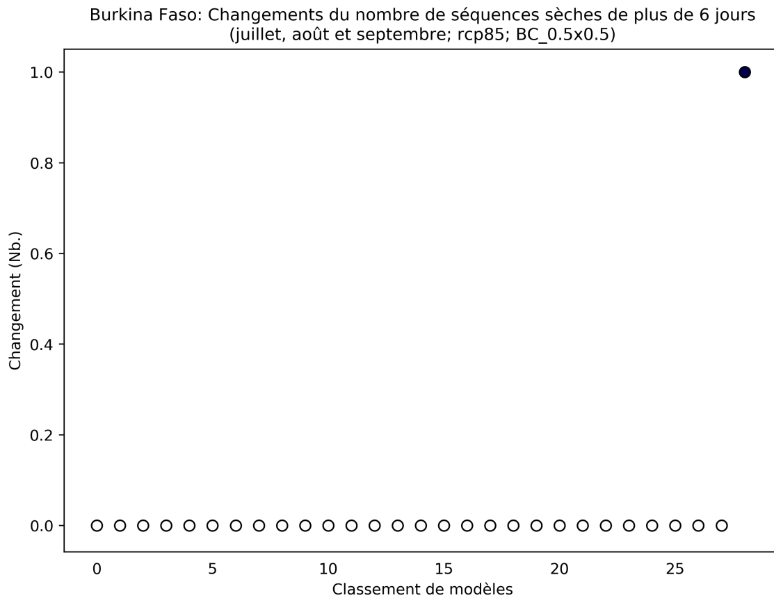
Figure 24: Ce diagramme de dispersion illustre la variation absolue du nombre de séquences sèches de plus de 6 jours entre 2040 et 2059 (par rapport à la période de référence de 1950 à 2000) pour juillet, août et septembre. Chaque point indique la moyenne spatiale d'un modèle sur Burkina Faso; les points sont organisés ("rank", sur l'axe des abscisses) en fonction de la magnitude de leur valeur sur l'axe des ordonnées. Ce diagramme montre la variation absolue pour le scénario RCP8.5.
