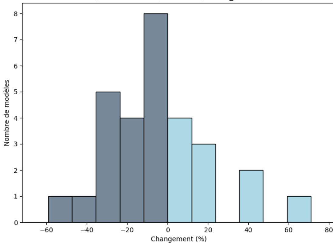
Burkina Faso: Changements (%) du maximum de précipitations totales sur une période de 5 jours (juillet, août et septembre; rcp85; BC_0.5x0.5)
