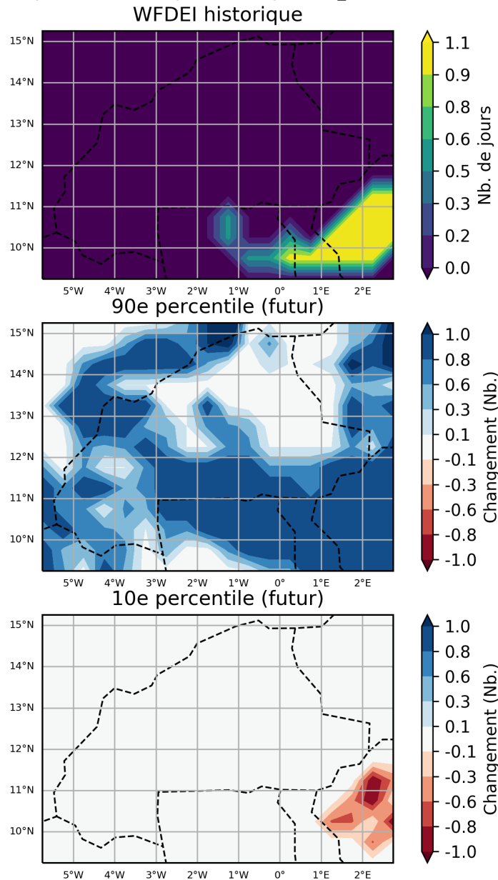
Figure 76: Ces cartes illustrent la projection multi-modèles pour la variation absolue du nombre de jours avec des précipitations > 50 \text{ mm jour}^{-1} , pour la période entre 2040 et 2059 (par rapport à la période de référence de 1950 à 2000) pour juillet, août et septembre. Elles indiquent les 90ème et 10ème percentiles de la distribution des modèles dans l'ensemble multi-modèles, calculés séparément en chaque point de grille, sur la région Burkina Faso. Ce diagramme montre la variation absolue pour le scénario RCP8.5.
