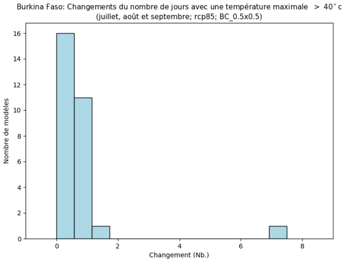
Figure 69: Cet histogramme illustre le nombre de modèles en accord avec la variation absolue du nombre de jours avec une température maximale > 40^{\circ}\text{C} pour la période entre 2040 et 2059 (par rapport à la période de référence de 1950 à 2000) pour juillet, août et septembre. Chaque barre verticale indique le nombre de modèles en accord avec la gamme de valeur indiquée sur l'axe des abscisses pour la région Burkina Faso. Ce diagramme montre la variation absolue pour le scénario RCP8.5.
