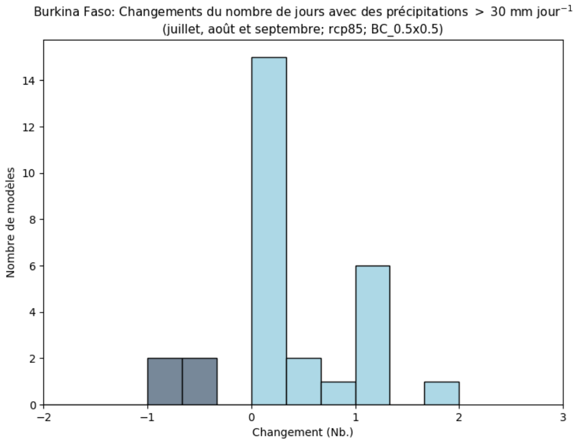
Figure 73: Cet histogramme illustre le nombre de modèles en accord avec la variation absolue du nombre de jours avec des précipitations > 30 mm jour -1 pour la période entre 2040 et 2059 (par rapport à la période de référence de 1950 à 2000) pour juillet, août et septembre. Chaque barre verticale indique le nombre de modèles en accord avec la gamme de valeur indiquée sur l'axe des abscisses pour la région Burkina Faso. Ce diagramme montre la variation absolue pour le scénario RCP8.5.
