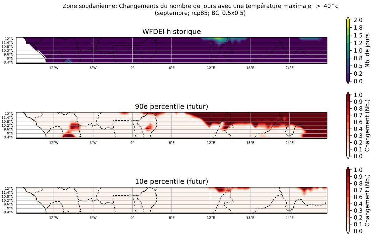
Figure 68: Ces cartes illustrent la projection multi-modèles pour la variation absolue du nombre de jours avec une température maximale > 40^{\circ}\text{C} , pour la période entre 2040 et 2059 (par rapport à la période de référence de 1950 à 2000) pour septembre. Elles indiquent les 90ème et 10ème percentiles de la distribution des modèles dans l'ensemble multi-modèles, calculés séparément en chaque point de grille, sur la région Zone soudanienne. Ce diagramme montre la variation absolue pour le scénario RCP8.5.
