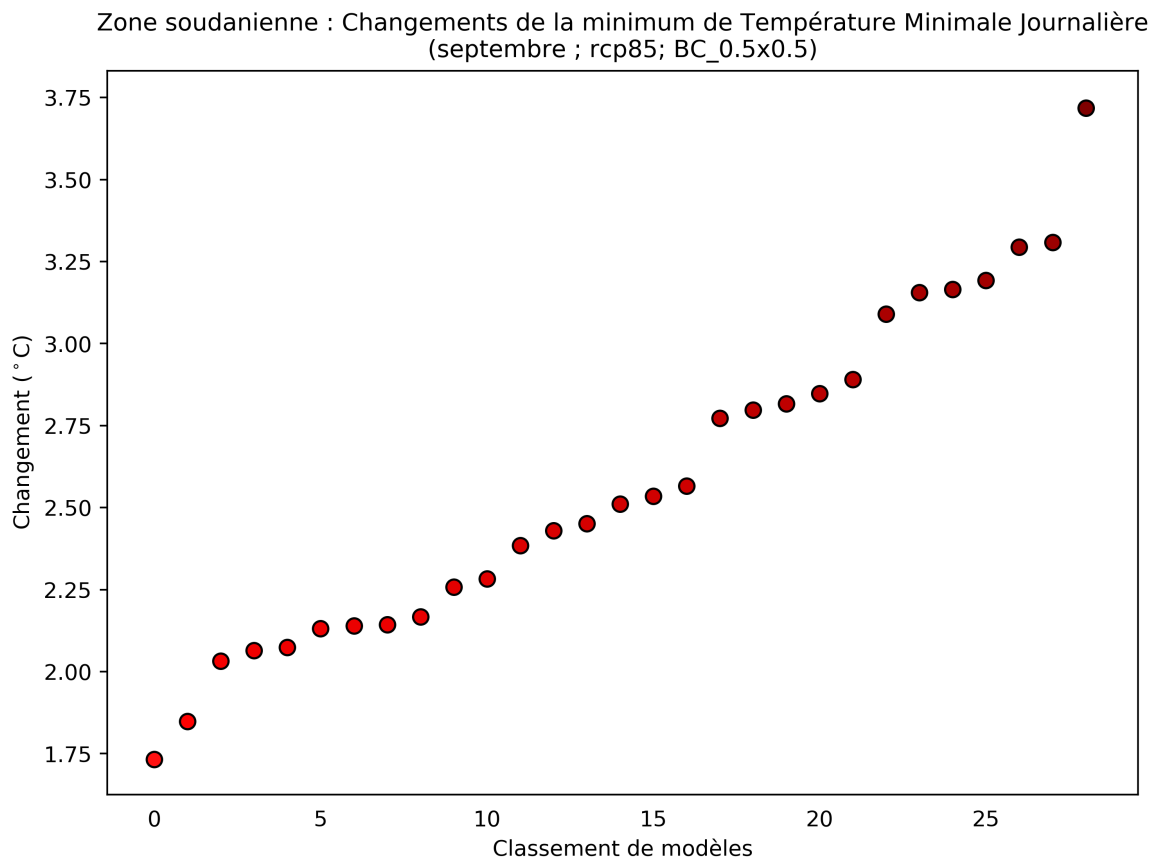
Figure 40: Ce diagramme de dispersion illustre la variation absolue de la minimum de température minimale journalière entre 2040 et 2059 (par rapport à la période de référence de 1950 à 2000) pour septembre. Chaque point indique la moyenne spatiale d'un modèle sur Zone soudanienne; les points sont organisés ("rank", sur l'axe des abscisses) en fonction de la magnitude de leur valeur sur l'axe des ordonnées. Ce diagramme montre la variation absolue pour le scénario RCP8.5.
