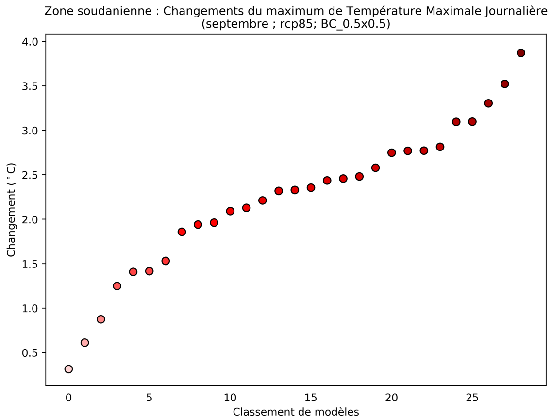
Figure 32: Ce diagramme de dispersion illustre la variation absolue du maximum de température maximale journalière entre 2040 et 2059 (par rapport à la période de référence de 1950 à 2000) pour septembre. Chaque point indique la moyenne spatiale d'un modèle sur Zone soudanienne; les points sont organisés ("rank", sur l'axe des abscisses) en fonction de la magnitude de leur valeur sur l'axe des ordonnées. Ce diagramme montre la variation absolue pour le scénario RCP8.5.
