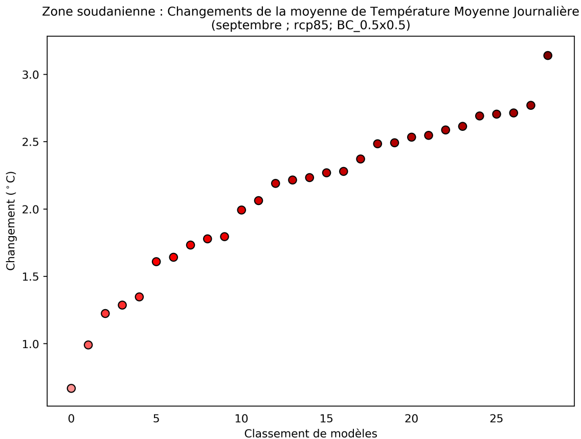
Figure 48: Ce diagramme de dispersion illustre la variation absolue de la moyenne de température moyenne journalière entre 2040 et 2059 (par rapport à la période de référence de 1950 à 2000) pour septembre. Chaque point indique la moyenne spatiale d'un modèle sur Zone soudanienne; les points sont organisés ("rank", sur l'axe des abscisses) en fonction de la magnitude de leur valeur sur l'axe des ordonnées. Ce diagramme montre la variation absolue pour le scénario RCP8.5.
