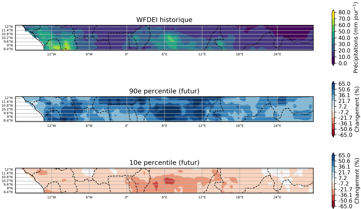
Figure 25: Ces cartes illustrent la projection multi-modèles pour du pourcentage de variation du maximum de précipitations journalières, pour la période entre 2040 et 2059 (par rapport à la période de référence de 1950 à 2000) pour septembre. Elles indiquent les 90ème et 10ème percentiles de la distribution des modèles dans l'ensemble multi-modèles, calculés séparément en chaque point de grille, sur la région Zone soudanienne. Ce diagramme montre le pourcentage de variation pour le scénario RCP8.5.
