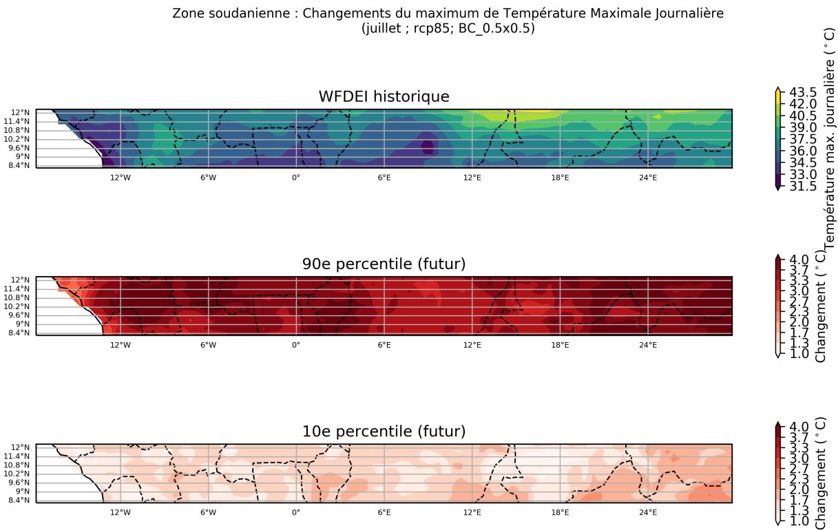
Figure 29: Ces cartes illustrent la projection multi-modèles pour la variation absolue du maximum de température maximale journalière, pour la période entre 2040 et 2059 (par rapport à la période de référence de 1950 à 2000) pour juillet. Elles indiquent les 90ème et 10ème percentiles de la distribution des modèles dans l'ensemble multi-modèles, calculés séparément en chaque point de grille, sur la région Zone soudanienne. Ce diagramme montre la variation absolue pour le scénario RCP8.5.
