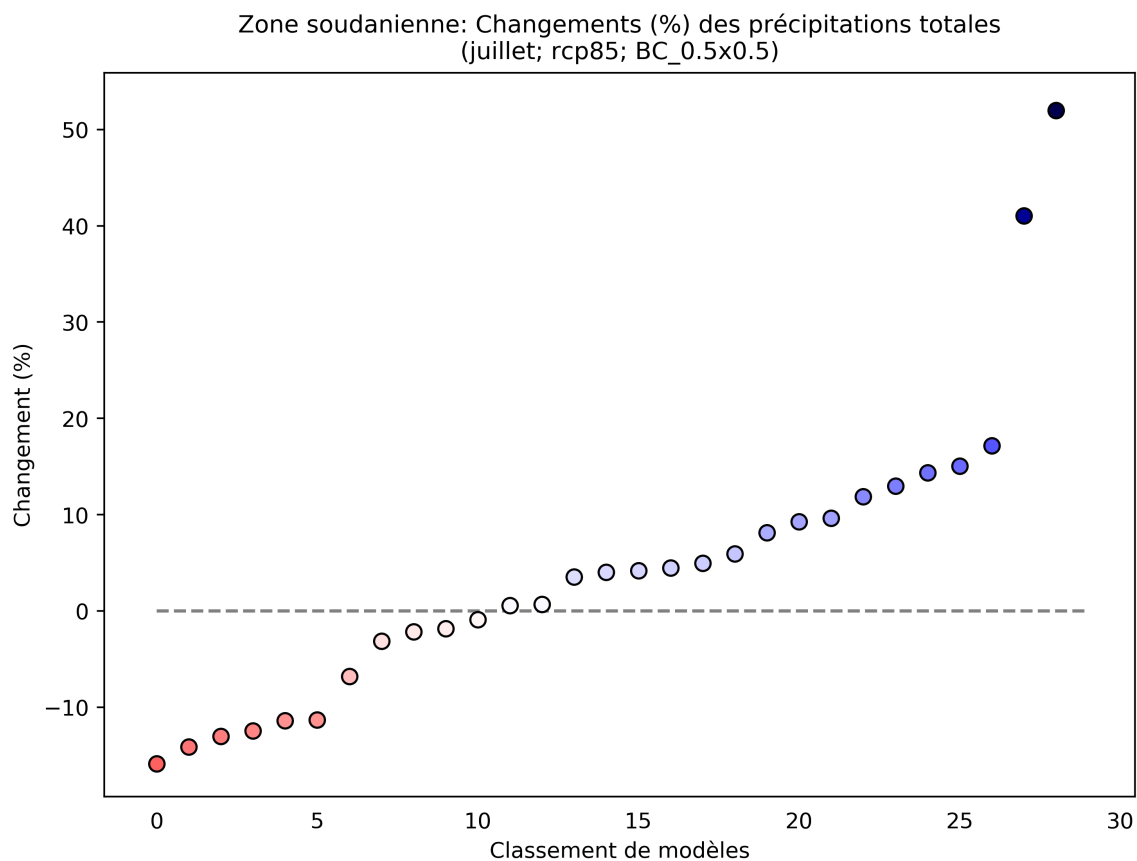
Figure 44: Ce diagramme de dispersion illustre du pourcentage de variation des précipitations totales entre 2040 et 2059 (par rapport à la période de référence de 1950 à 2000) pour juillet. Chaque point indique la moyenne spatiale d'un modèle sur Zone soudanienne; les points sont organisés ("rank", sur l'axe des abscisses) en fonction de la magnitude de leur valeur sur l'axe des ordonnées. Ce diagramme montre le pourcentage de variation pour le scénario RCP8.5.
