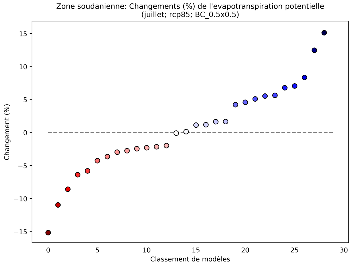
Figure 4: Ce diagramme de dispersion illustre du pourcentage de variation de l'évapotranspiration potentielle entre 2040 et 2059 (par rapport à la période de référence de 1950 à 2000) pour juillet. Chaque point indique la moyenne spatiale d'un modèle sur Zone soudanienne; les points sont organisés ("rank", sur l'axe des abscisses) en fonction de la magnitude de leur valeur sur l'axe des ordonnées. Ce diagramme montre le pourcentage de variation pour le scénario RCP8.5.
