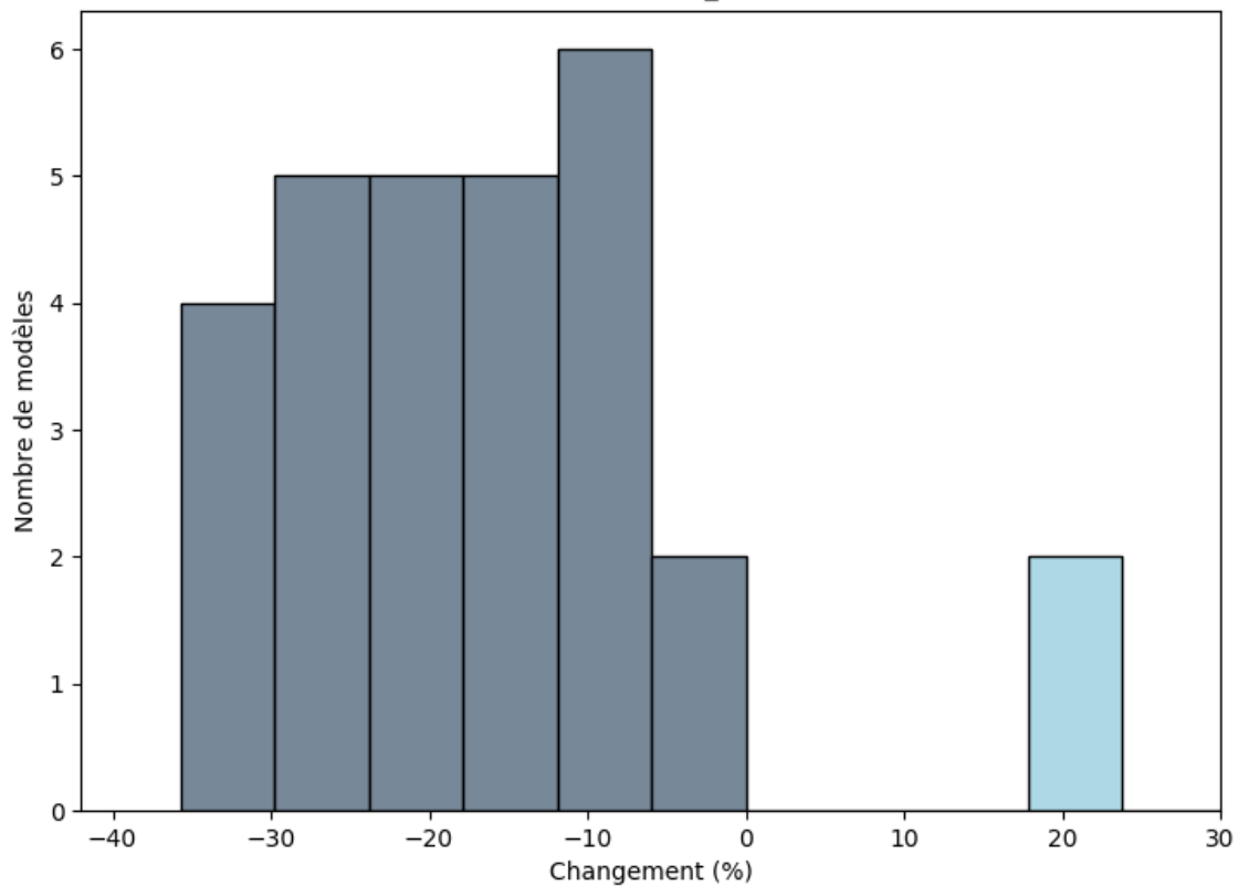
Zone soudanienne: Changements (%) du maximum de précipitations totales sur une période de 2 jours (juillet; rcp85; BC_0.5x0.5)
