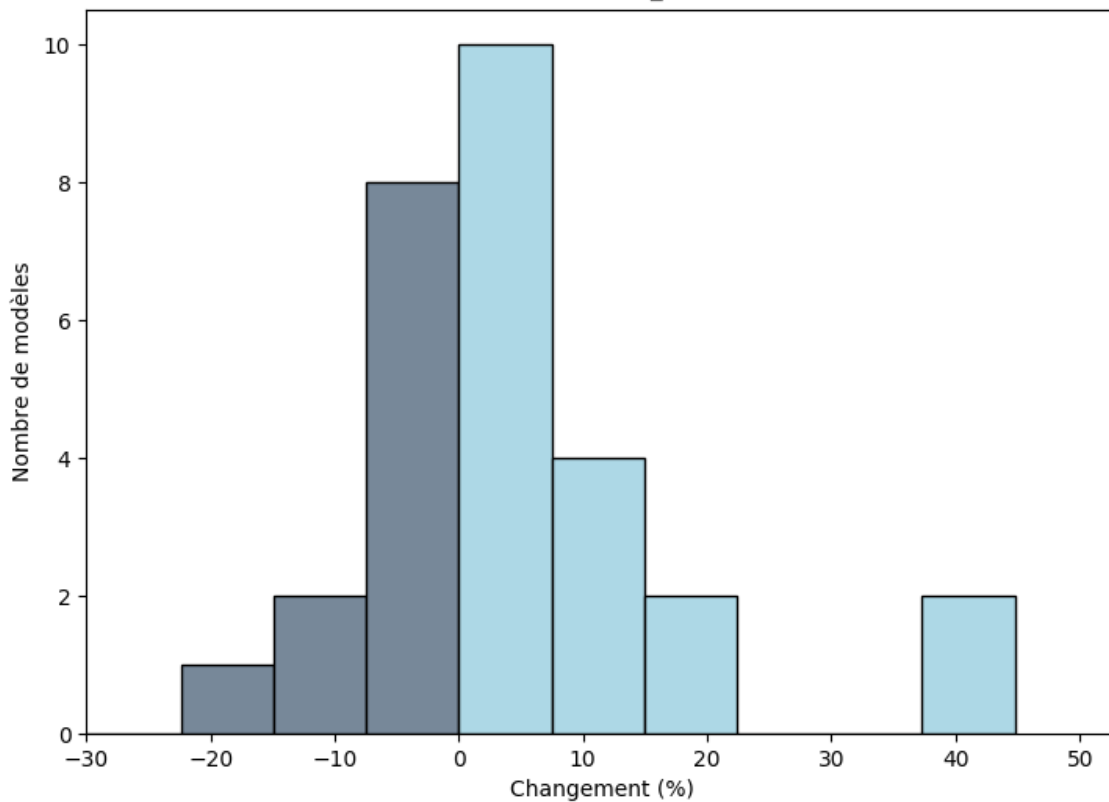
Zone soudanienne: Changements (%) du maximum de précipitations totales sur une période de 5 jours (juillet; rcp85; BC_0.5x0.5)
