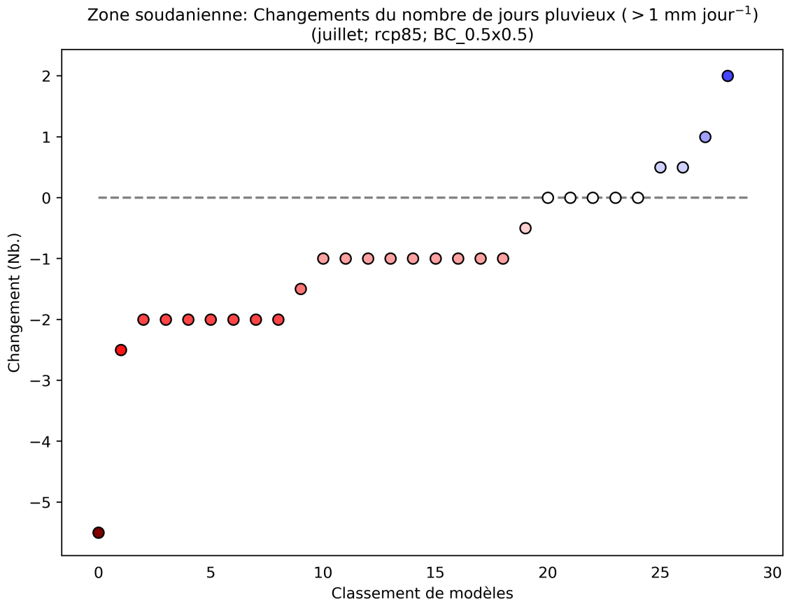
Figure 67: Ce diagramme de dispersion illustre la variation absolue du nombre de jours pluvieux (>1 mm jour -1 ) entre 2040 et 2059 (par rapport à la période de référence de 1950 à 2000) pour juillet. Chaque point indique la moyenne spatiale d'un modèle sur Zone soudanienne; les points sont organisés ("rank", sur l'axe des abscisses) en fonction de la magnitude de leur valeur sur l'axe des ordonnées. Ce diagramme montre la variation absolue pour le scénario RCP8.5.
