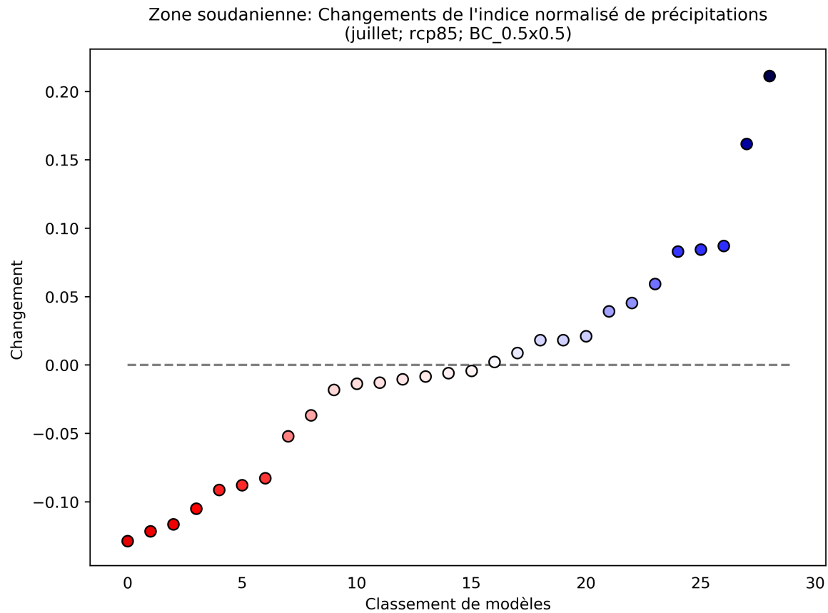
Figure 12: Ce diagramme de dispersion illustre la variation absolue de l'indice normalisé de précipitations entre 2040 et 2059 (par rapport à la période de référence de 1950 à 2000) pour juillet. Chaque point indique la moyenne spatiale d'un modèle sur Zone soudanienne; les points sont organisés ("rank", sur l'axe des abscisses) en fonction de la magnitude de leur valeur sur l'axe des ordonnées. Ce diagramme montre la variation absolue pour le scénario RCP8.5.
