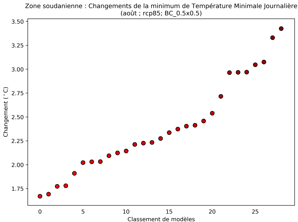
Figure 40: Ce diagramme de dispersion illustre la variation absolue de la minimum de température minimale journalière entre 2040 et 2059 (par rapport à la période de référence de 1950 à 2000) pour août. Chaque point indique la moyenne spatiale d'un modèle sur Zone soudanienne; les points sont organisés ("rank", sur l'axe des abscisses) en fonction de la magnitude de leur valeur sur l'axe des ordonnées. Ce diagramme montre la variation absolue pour le scénario RCP8.5.
