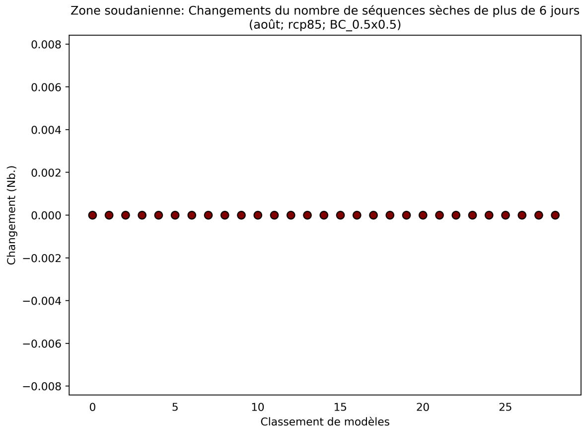
Figure 24: Ce diagramme de dispersion illustre la variation absolue du nombre de séquences sèches de plus de 6 jours entre 2040 et 2059 (par rapport à la période de référence de 1950 à 2000) pour août. Chaque point indique la moyenne spatiale d'un modèle sur Zone soudanienne; les points sont organisés ("rank", sur l'axe des abscisses) en fonction de la magnitude de leur valeur sur l'axe des ordonnées. Ce diagramme montre la variation absolue pour le scénario RCP8.5.
