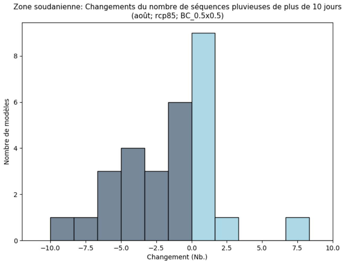
Figure 18: Cet histogramme illustre le nombre de modèles en accord avec la variation absolue du nombre de séquences pluvieuses de plus de 10 jours pour la période entre 2040 et 2059 (par rapport à la période de référence de 1950 à 2000) pour août. Chaque barre verticale indique le nombre de modèles en accord avec la gamme de valeur indiquée sur l'axe des abscisses pour la région Zone soudanienne. Ce diagramme montre la variation absolue pour le scénario RCP8.5.
