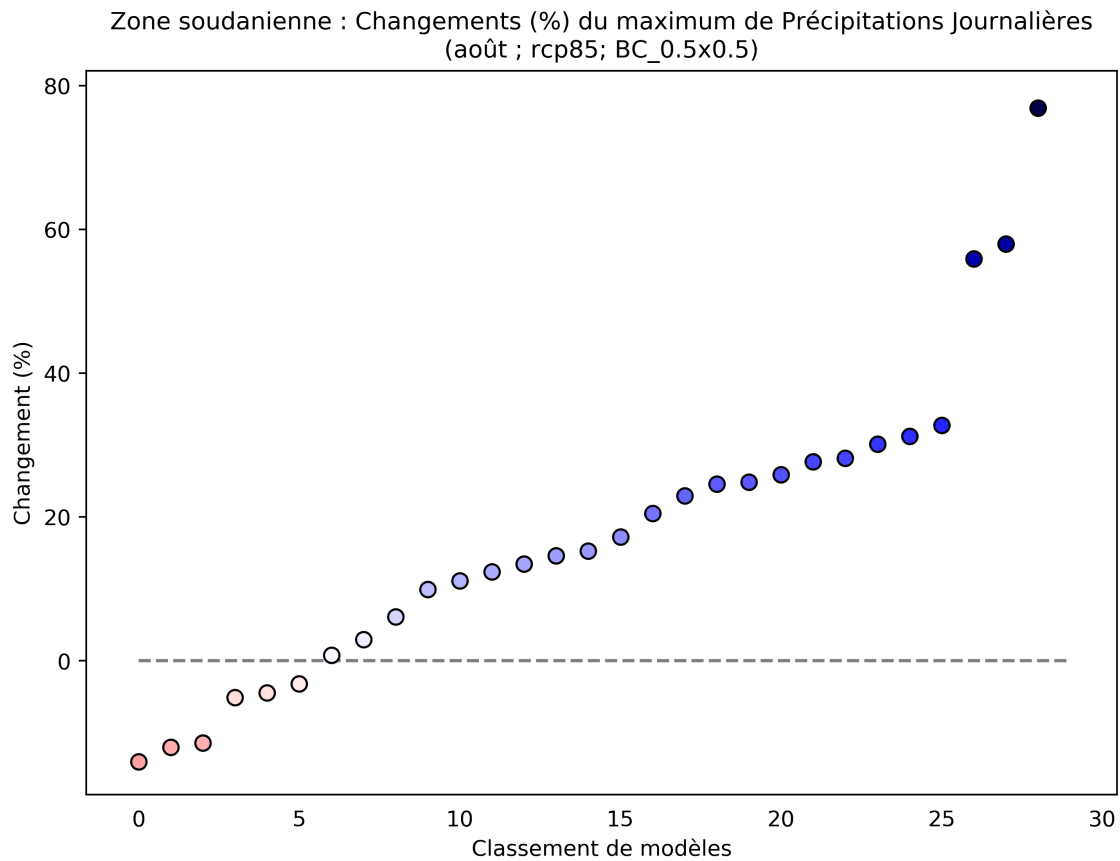
Figure 28: Ce diagramme de dispersion illustre du pourcentage de variation du maximum de précipitations journalières entre 2040 et 2059 (par rapport à la période de référence de 1950 à 2000) pour août. Chaque point indique la moyenne spatiale d'un modèle sur Zone soudanienne; les points sont organisés ("rank", sur l'axe des abscisses) en fonction de la magnitude de leur valeur sur l'axe des ordonnées. Ce diagramme montre le pourcentage de variation pour le scénario RCP8.5.
