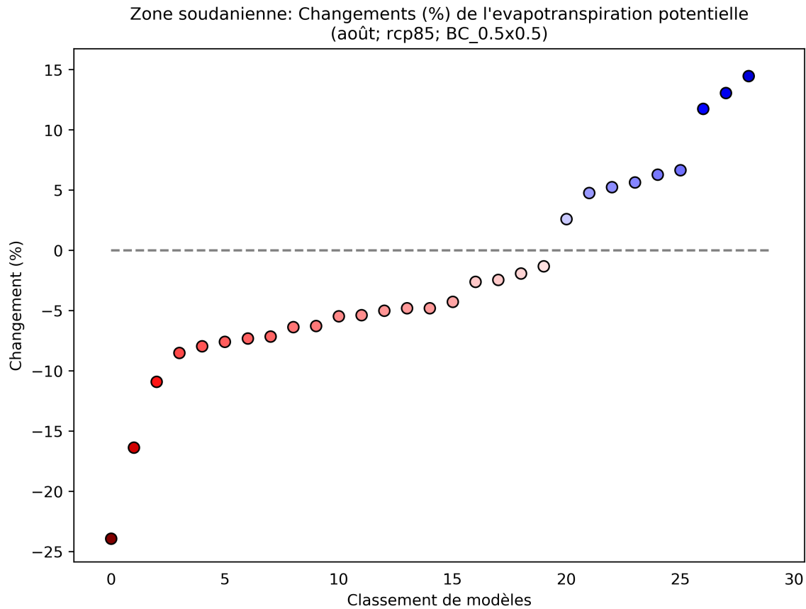
Figure 4: Ce diagramme de dispersion illustre du pourcentage de variation de l'évapotranspiration potentielle entre 2040 et 2059 (par rapport à la période de référence de 1950 à 2000) pour août. Chaque point indique la moyenne spatiale d'un modèle sur Zone soudanienne; les points sont organisés ("rank", sur l'axe des abscisses) en fonction de la magnitude de leur valeur sur l'axe des ordonnées. Ce diagramme montre le pourcentage de variation pour le scénario RCP8.5.
