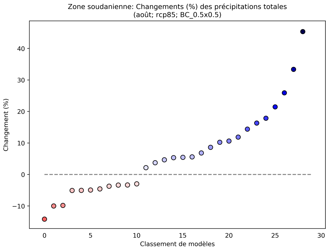
Figure 44: Ce diagramme de dispersion illustre du pourcentage de variation des précipitations totales entre 2040 et 2059 (par rapport à la période de référence de 1950 à 2000) pour août. Chaque point indique la moyenne spatiale d'un modèle sur Zone soudanienne; les points sont organisés ("rank", sur l'axe des abscisses) en fonction de la magnitude de leur valeur sur l'axe des ordonnées. Ce diagramme montre le pourcentage de variation pour le scénario RCP8.5.
