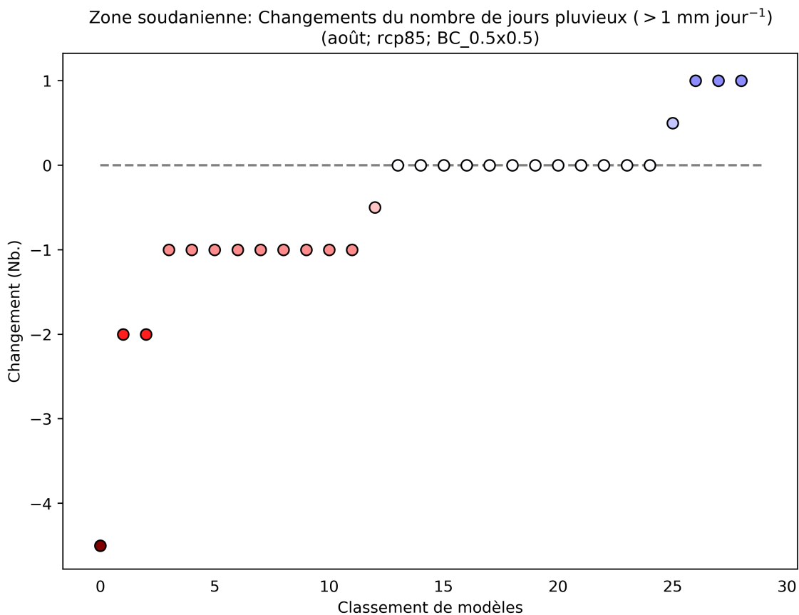
Figure 67: Ce diagramme de dispersion illustre la variation absolue du nombre de jours pluvieux (>1 mm jour -1 ) entre 2040 et 2059 (par rapport à la période de référence de 1950 à 2000) pour août. Chaque point indique la moyenne spatiale d'un modèle sur Zone soudanienne; les points sont organisés ("rank", sur l'axe des abscisses) en fonction de la magnitude de leur valeur sur l'axe des ordonnées. Ce diagramme montre la variation absolue pour le scénario RCP8.5.
