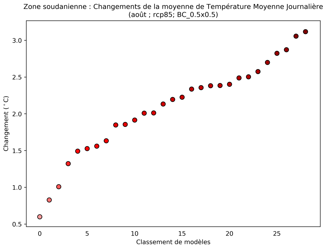
Figure 48: Ce diagramme de dispersion illustre la variation absolue de la moyenne de température moyenne journalière entre 2040 et 2059 (par rapport à la période de référence de 1950 à 2000) pour août. Chaque point indique la moyenne spatiale d'un modèle sur Zone soudanienne; les points sont organisés ("rank", sur l'axe des abscisses) en fonction de la magnitude de leur valeur sur l'axe des ordonnées. Ce diagramme montre la variation absolue pour le scénario RCP8.5.
