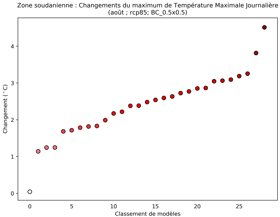
Figure 32: Ce diagramme de dispersion illustre la variation absolue du maximum de température maximale journalière entre 2040 et 2059 (par rapport à la période de référence de 1950 à 2000) pour août. Chaque point indique la moyenne spatiale d'un modèle sur Zone soudanienne; les points sont organisés ("rank", sur l'axe des abscisses) en fonction de la magnitude de leur valeur sur l'axe des ordonnées. Ce diagramme montre la variation absolue pour le scénario RCP8.5.
