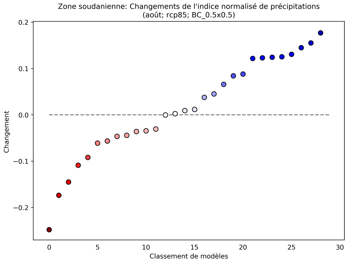
Figure 12: Ce diagramme de dispersion illustre la variation absolue de l'indice normalisé de précipitations entre 2040 et 2059 (par rapport à la période de référence de 1950 à 2000) pour août. Chaque point indique la moyenne spatiale d'un modèle sur Zone soudanienne; les points sont organisés ("rank", sur l'axe des abscisses) en fonction de la magnitude de leur valeur sur l'axe des ordonnées. Ce diagramme montre la variation absolue pour le scénario RCP8.5.
